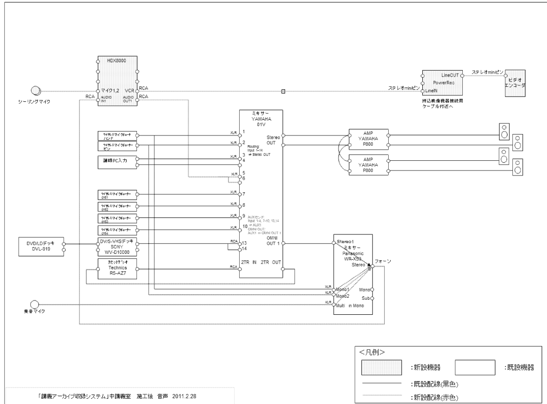
図 10 音響設備配線参考図
