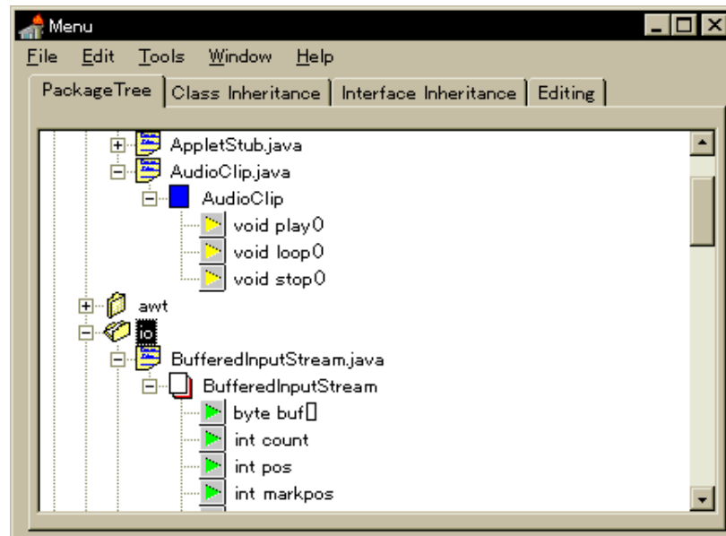
図 5.2: メインクラスブラウザ
