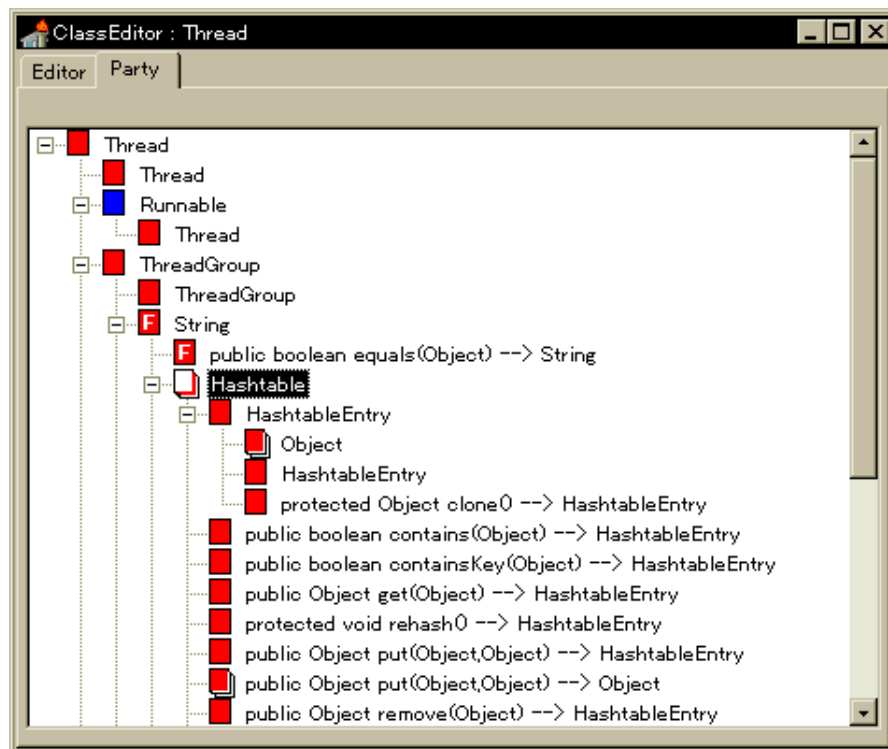
図 5.7: Party 連鎖ブラウザ
