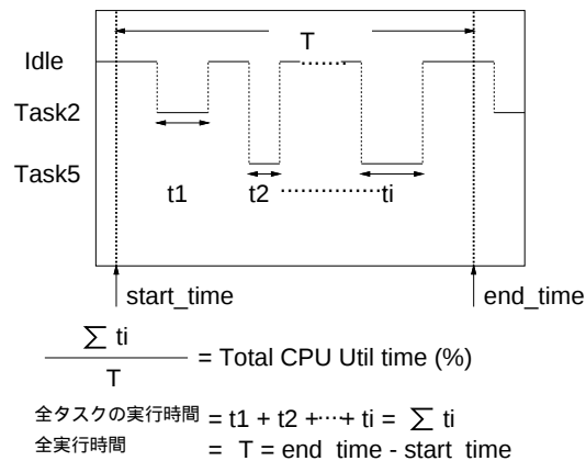
図 4.6: CPU 使用率の算出
