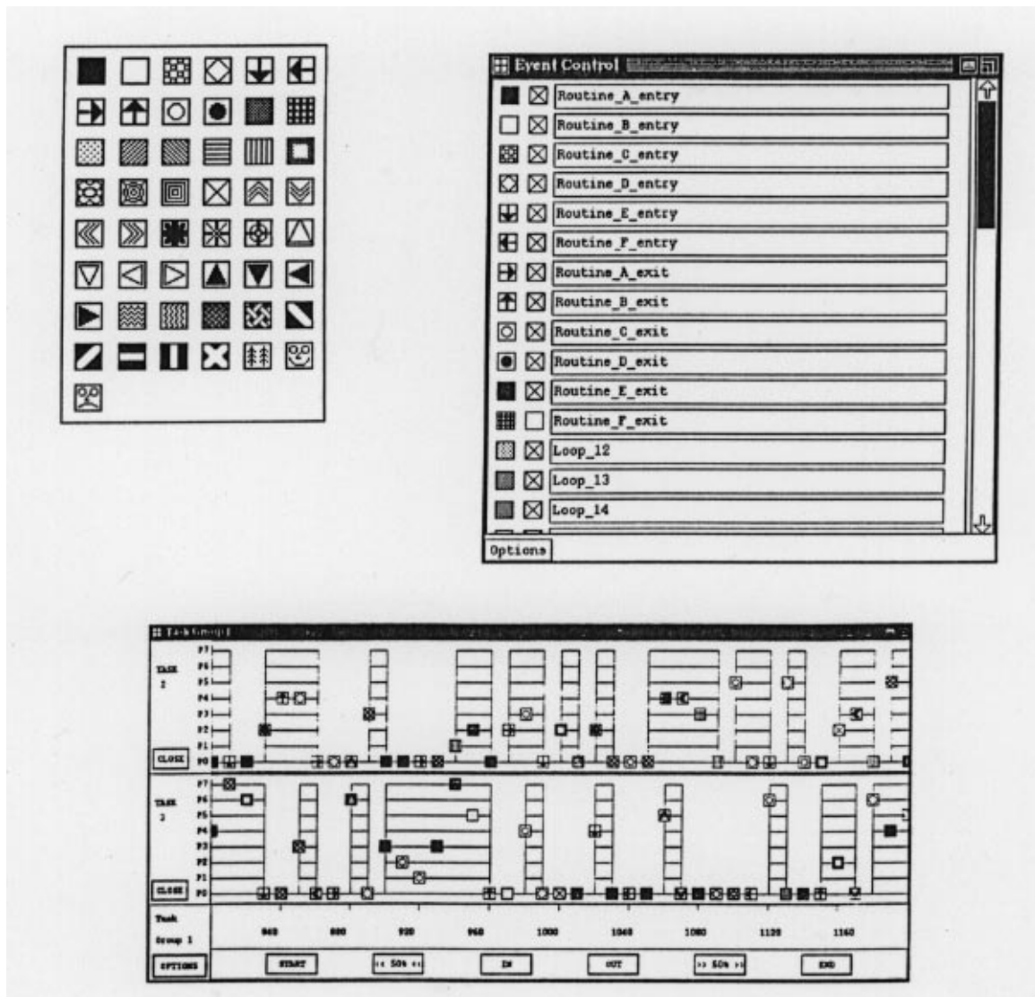
図 2.2: JED による視覚化の例 , 左上 : Event image map , 右上 : Event control , 下 : Task display
