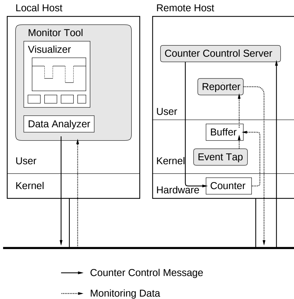
図 3.1: Performance Tool の全体構造の概略
