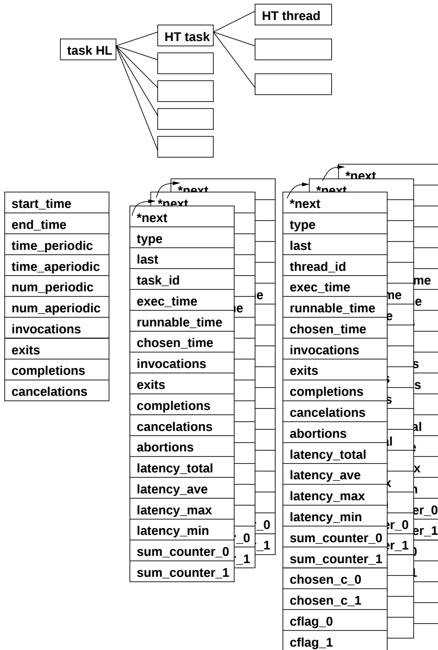
図 4.4: データ構造
