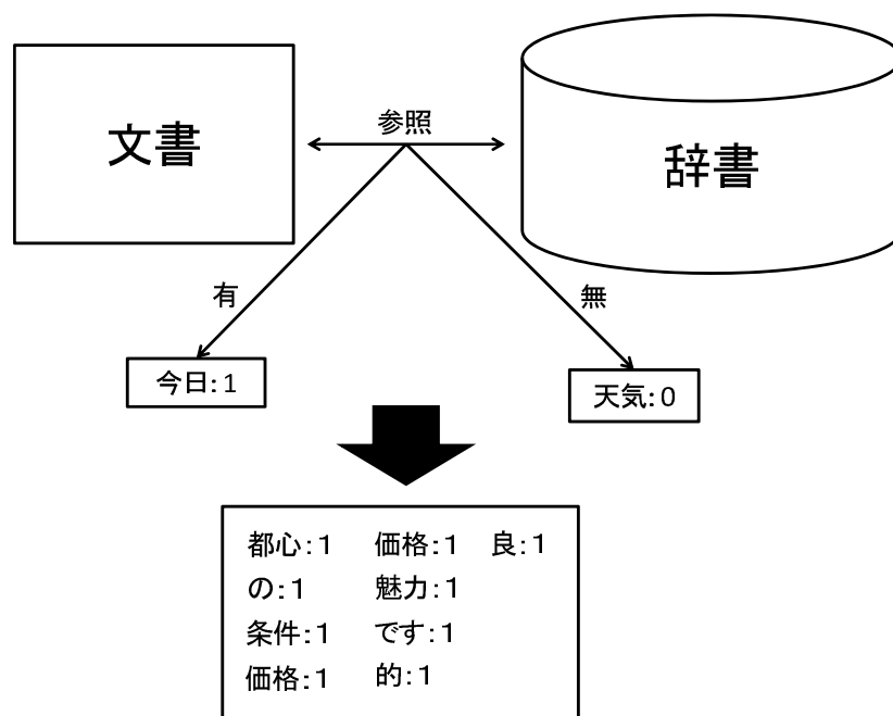
図 3.1: 素性ベクトルの抽出
