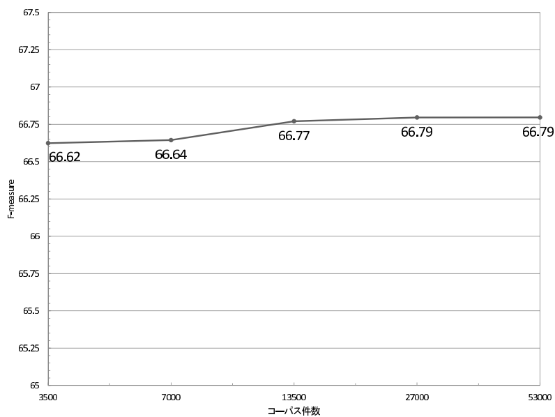
図 4.8: trigram を用いたデータセット
