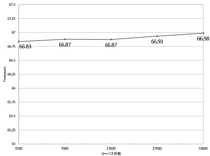
図 4.7: bigram を用いたデータセット
