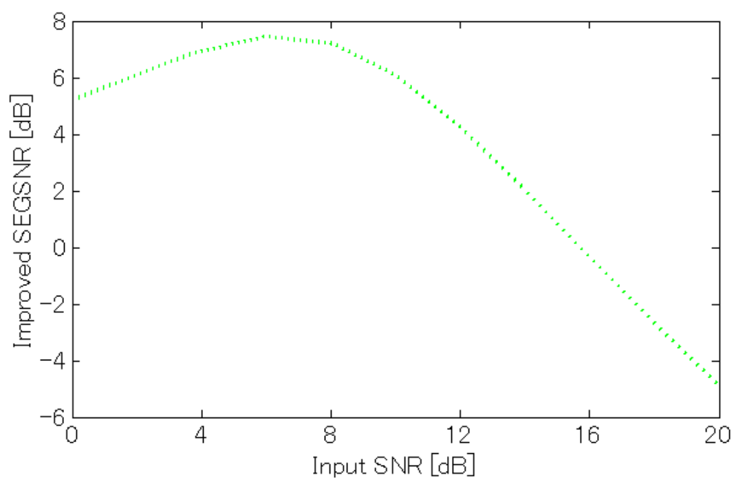
図 6.5: CMS のエコーに対する耐性評価実験結果：縦軸は SEGSNR の改善量，横軸は受信信号の全区間 SN 比を示す
