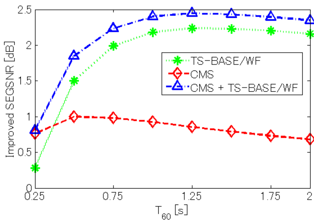
図 7.1: 各手法の残響耐性評価実験結果：縦軸は SEGSR 改善量，横軸は残響時間を示す
