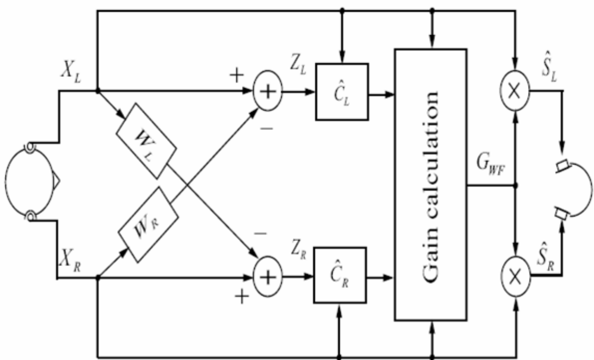
図 2.1: TS-BASE/WF のブロックダイアグラム
