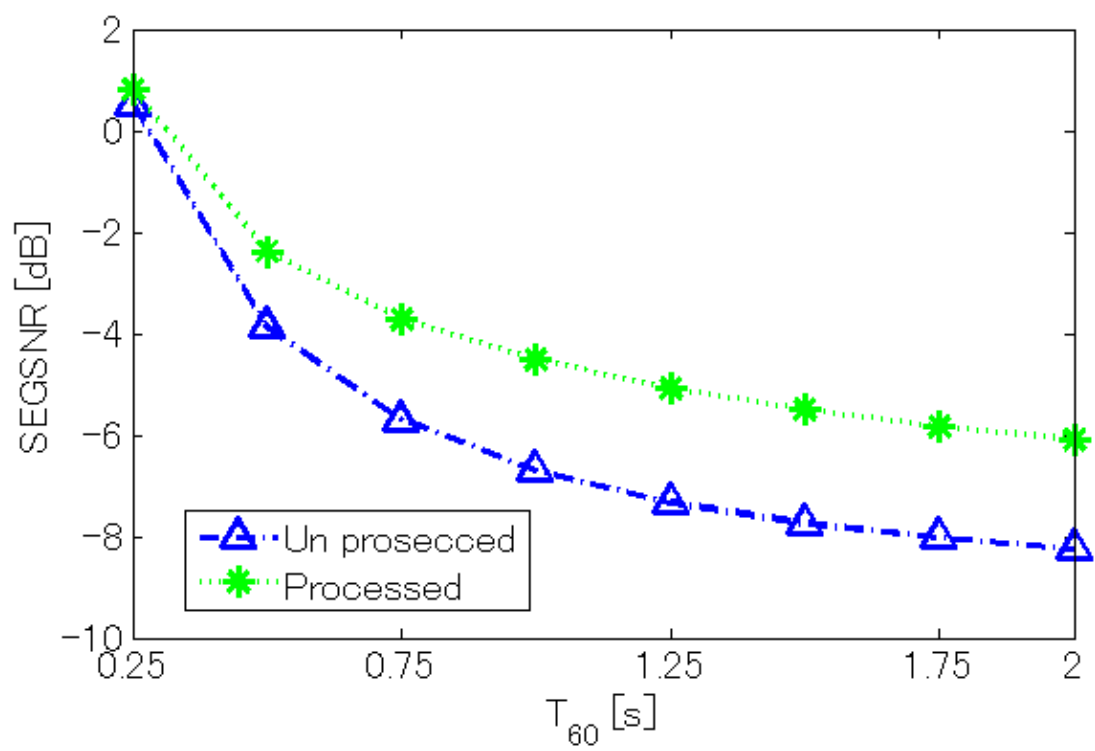
図 4.3: TS-BASE/WF の残響耐性評価実験結果：縦軸は SEGSNR，横軸は残響時間を示す
