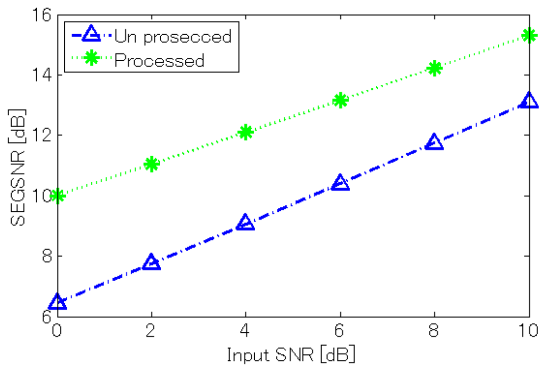
図 4.1: TS-BASE/WF の雑音耐性評価実験結果：縦軸は SEGSR，横軸は受信信号の全区間 SN 比を示す
