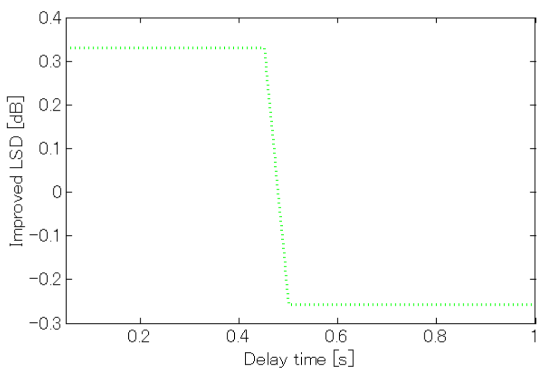
図 6.4: CMS のエコーに対する耐性評価実験結果：縦軸は LSD の改善量，横軸はエコーに付加した遅延時間を示す
