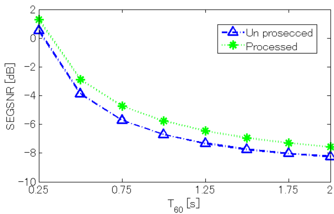
図 6.7: CMS の残響耐性評価実験結果：縦軸は SEGSR, 横軸は残響時間を示す
