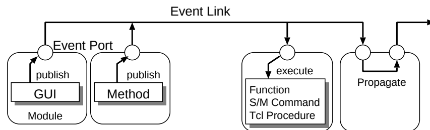
図 4.3: Event
