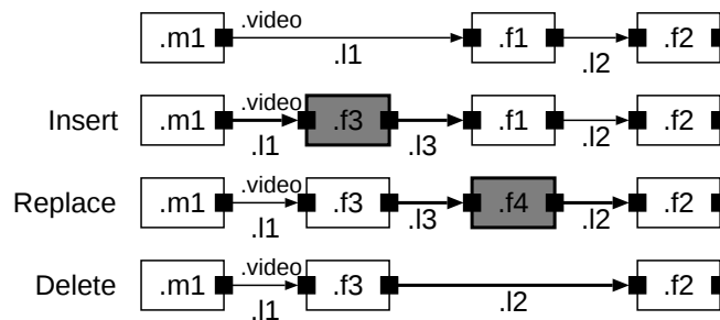
図 6.1: Module Operation
