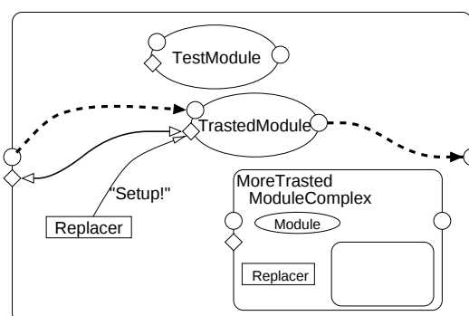
図 3.5: Replace Errored Module
