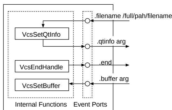
図 A.1: VideoCrasSrc Module
