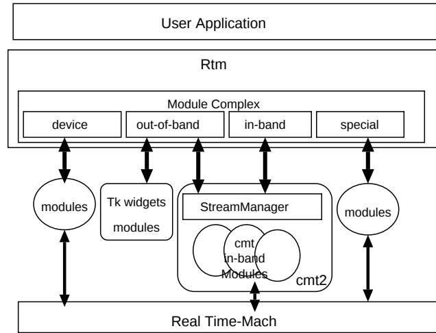
図 5.1: Rtm and Cmt
