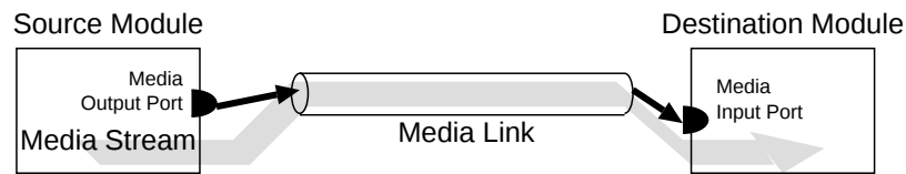
図 4.2: Media Link
