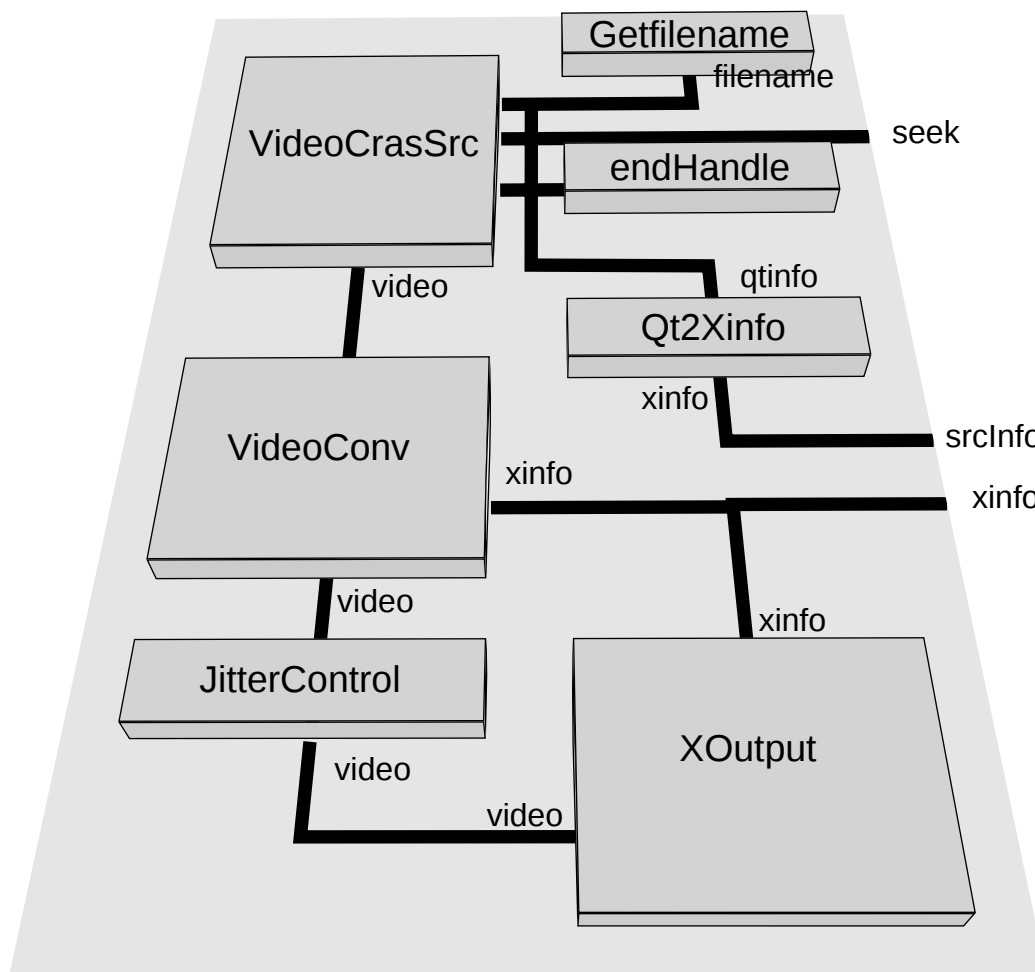
❏ 6.2: QtCmt
