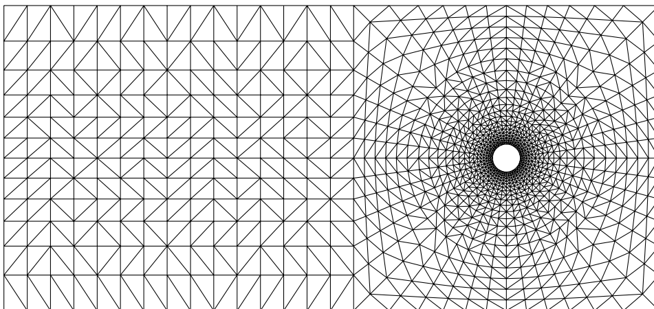
図 2.13: 要素分割図
