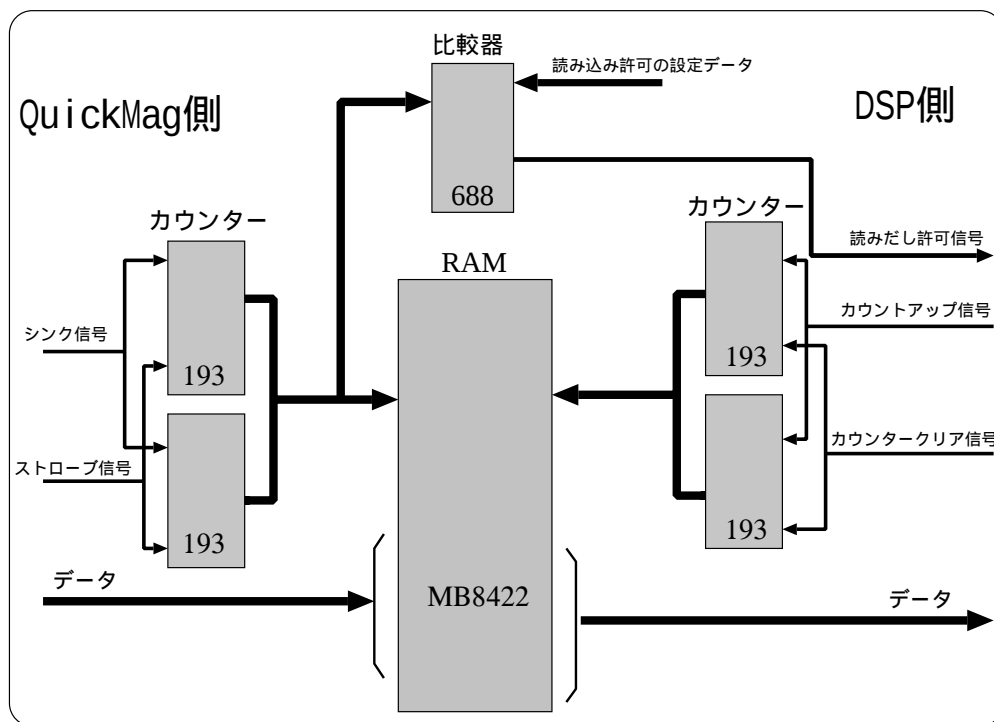
図 5.3: バッファボード
