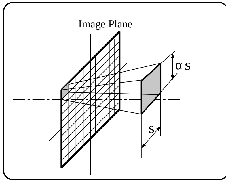
図 5.1: 画像面での縦横比
