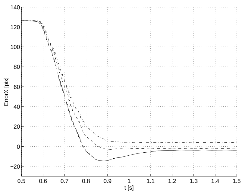
図 5.10: \xi_x の偏差 k_p = 9e - 4
