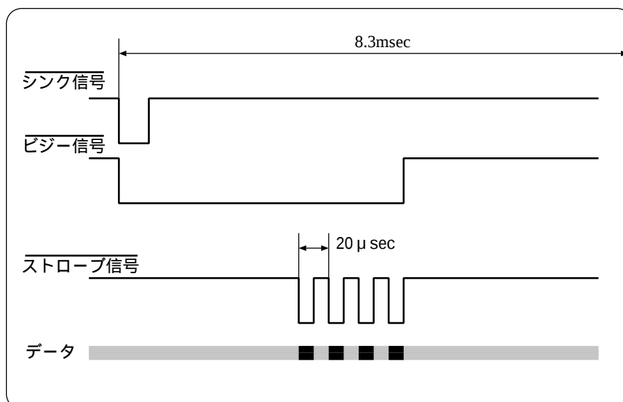
図 5.4: イメージプロセッサの出力信号
