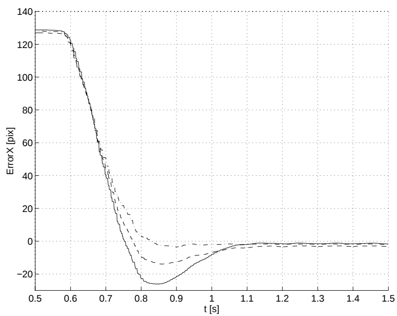
図 5.11: \xi_x の偏差 k_p = 11e - 4
