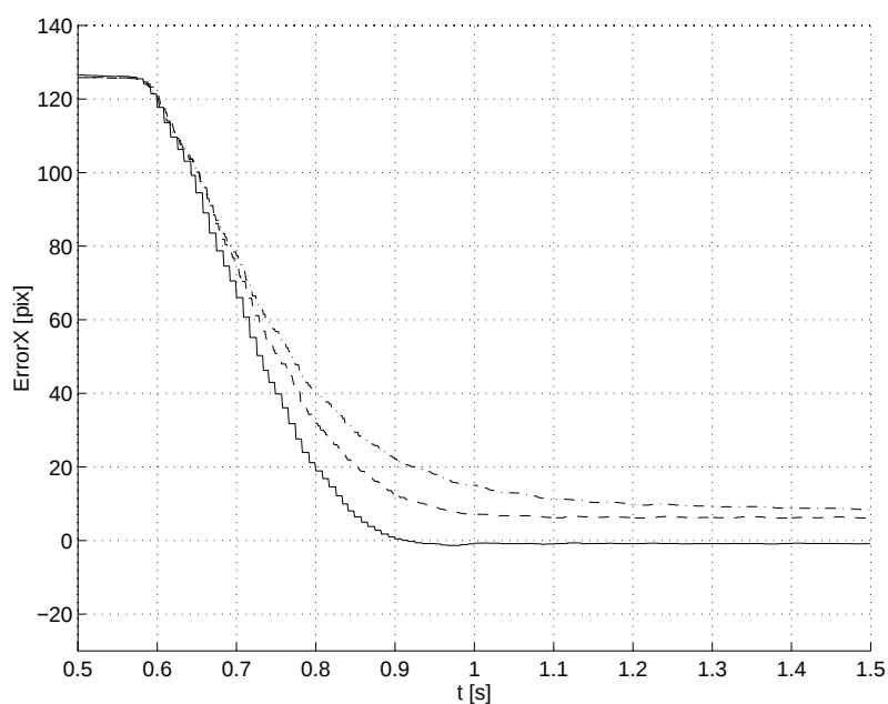
図 5.9: \xi_x の偏差 k_p = 7e-4
