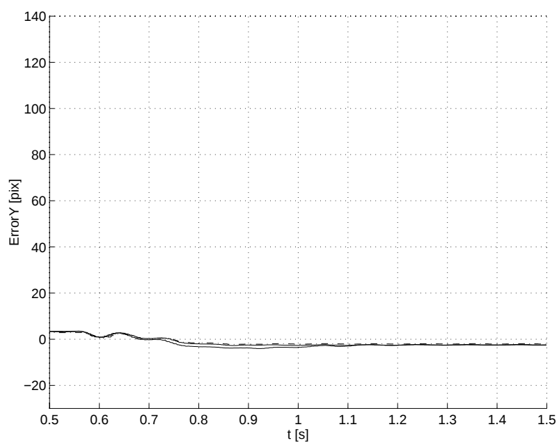
図 5.13: \xi_y の偏差 k_p = 9e - 4
