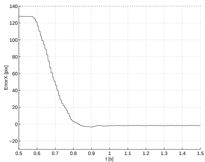
図 5.7: 実験結果 \xi_x K_p = 11e - 3, k_p = 55
