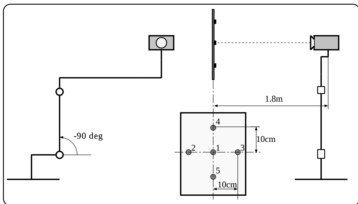
図 5.6: 実験での初期姿勢と対象物
