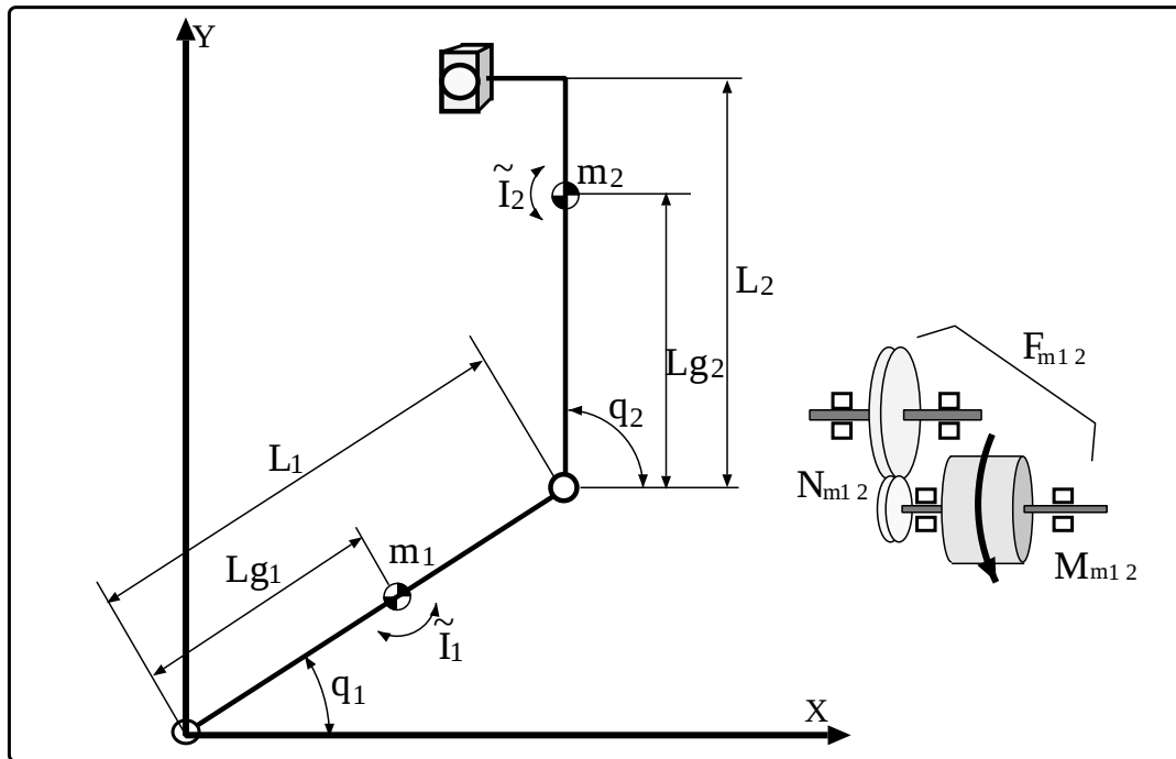
図 3.4: SC-15 の物理モデル
