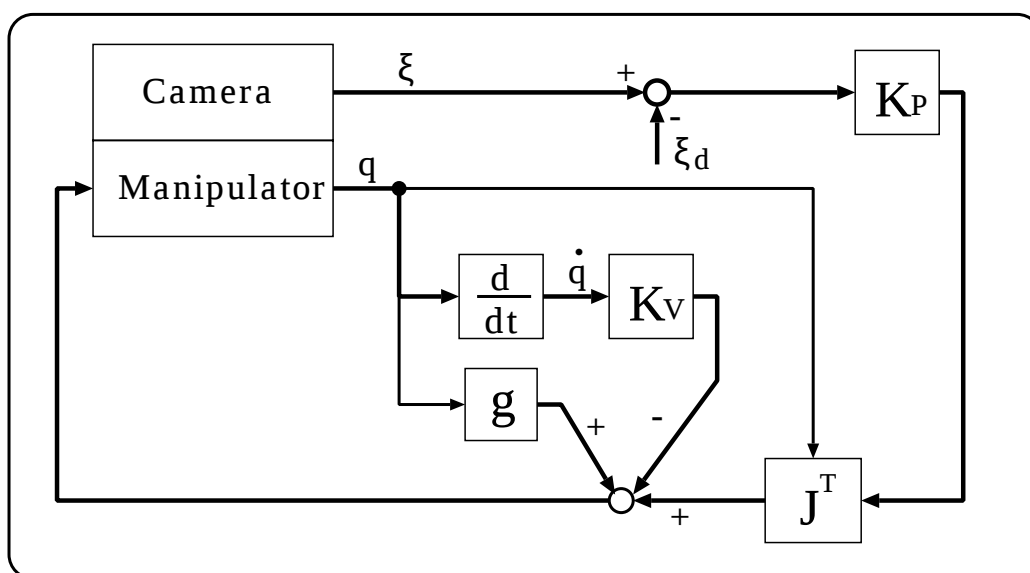
図 5. 5: PD 制御系
