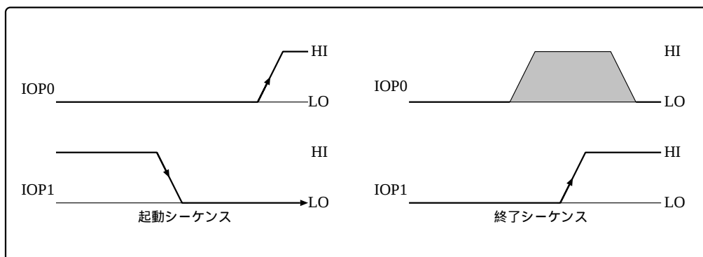
図 2. 2: アーム#1 の起動シーケンスと終了シーケンス
