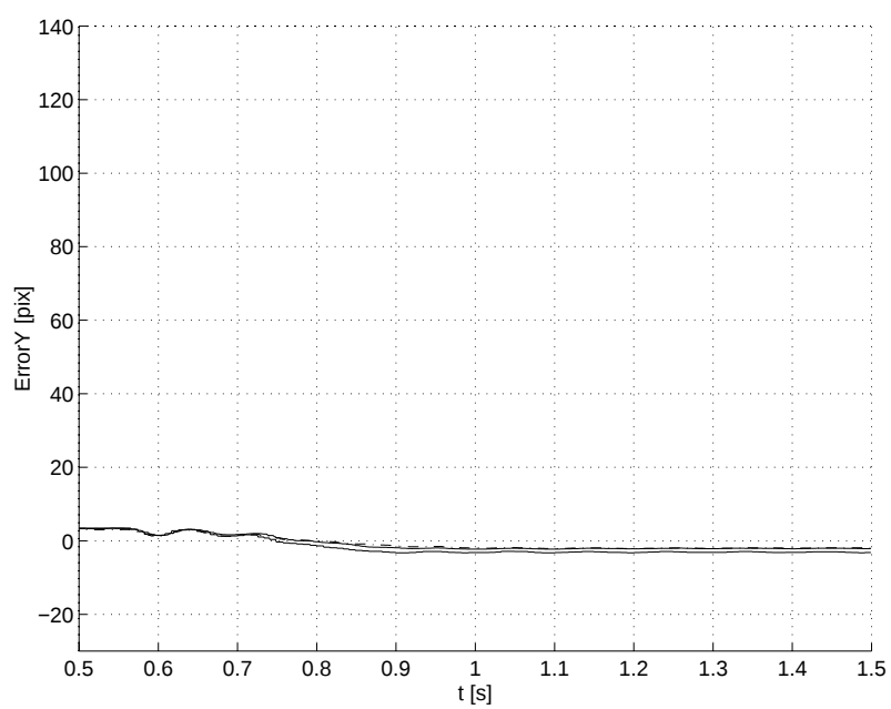
図 5.12: \xi_y の偏差 k_p = 7e - 4
