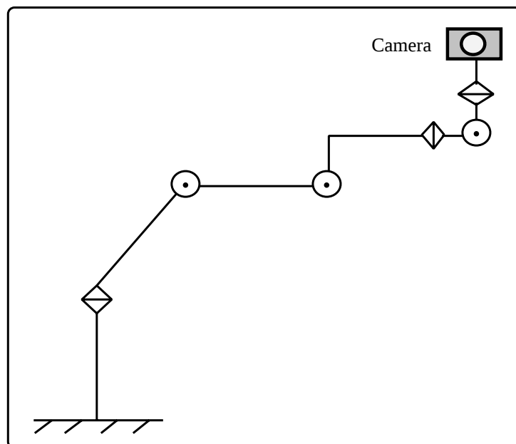
図 3.1: SC-15 の機構モデル
