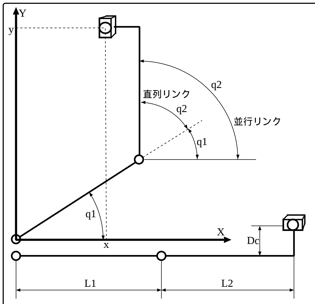
図 3.3: 直列リンク機構での関節角と並列リンク機構での関節角
