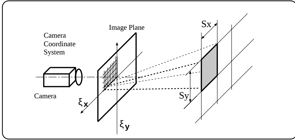
図 3.6: カメラのピクセル長
