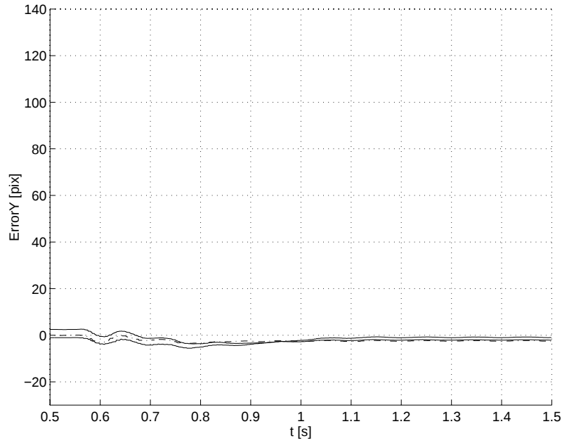
図 5.14: \xi_y の偏差 k_p = 11e - 4
