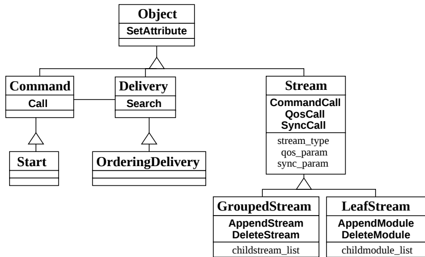
図 5.9: Start 命令呼び出しで使用するオブジェクトのクラス
