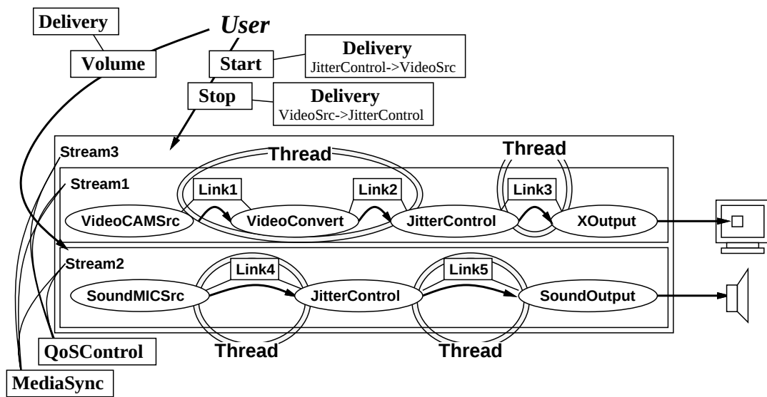
図 6.2: ビデオカンファレンスシステム
