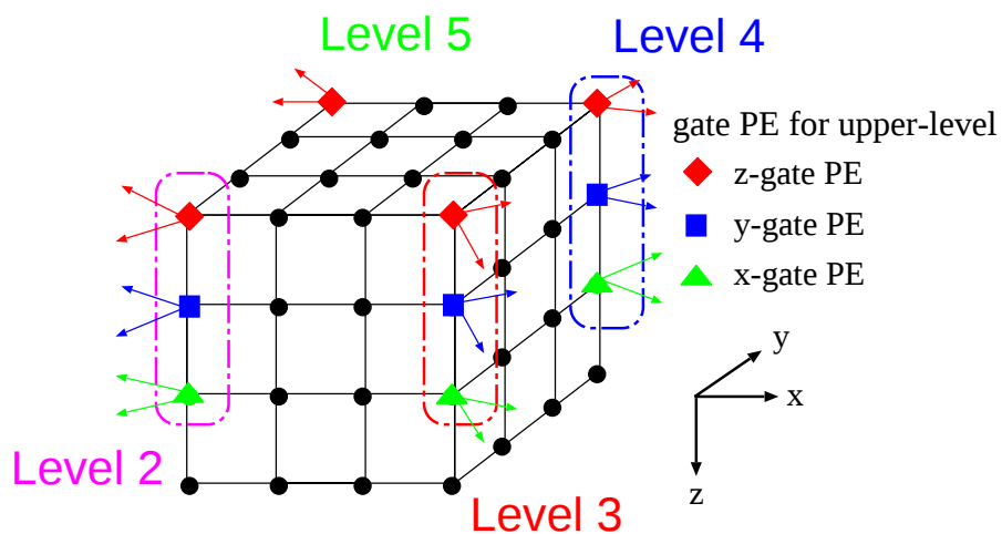
図 3.1: 3D 階層型トーラスの基本モジュール
