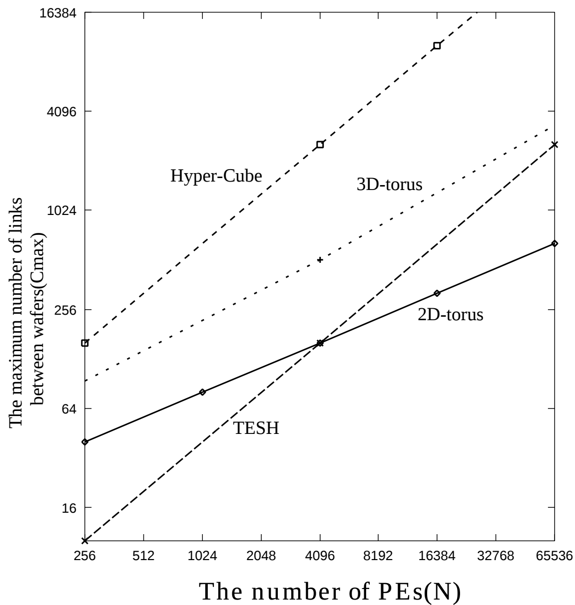
図 2.22: ウェーハ間最大結線数 ( C_{max} )
