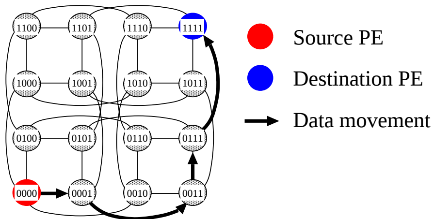
図 2.12: ハイパーキューブのルーティング (N=16)
