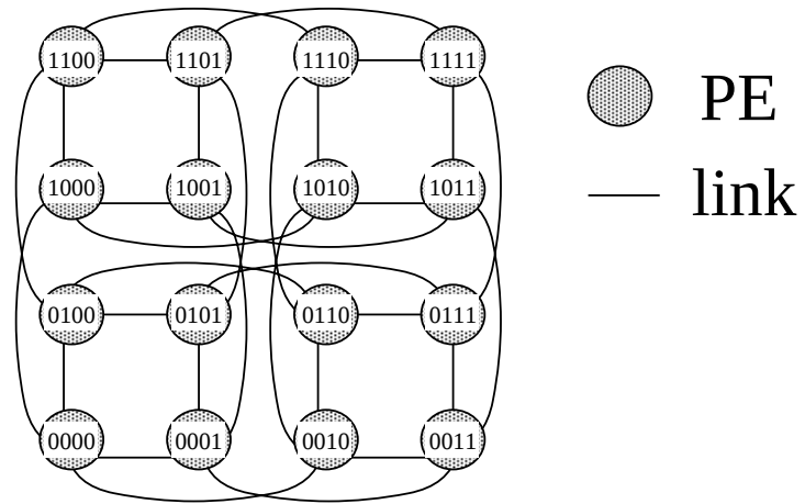
図 2.11: ハイパーキューブ (N=16)
