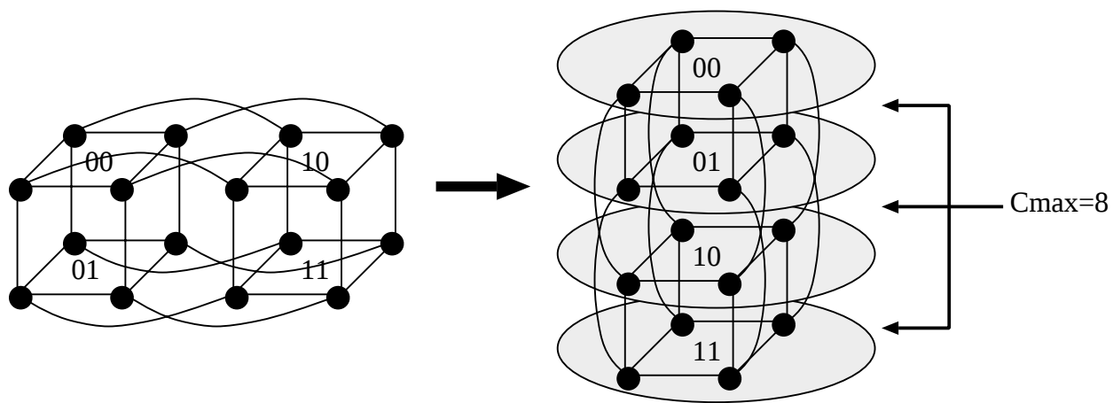
図 2.13: ハイパーキューブのウェーハ間最大結線数 C_{max}(N=16, m=4)
