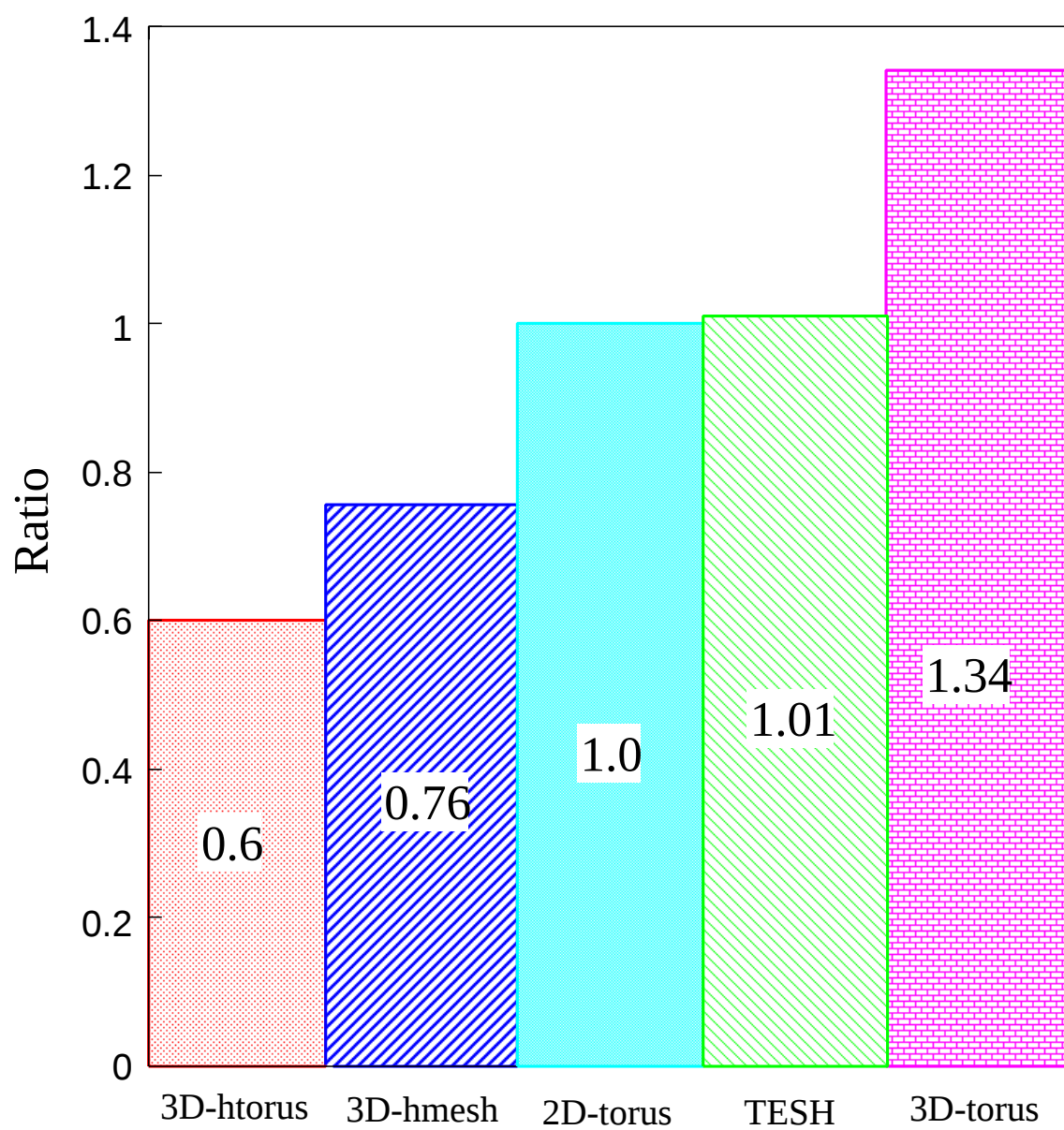
図 3.9: レイアウト面積 A(N=4096)
