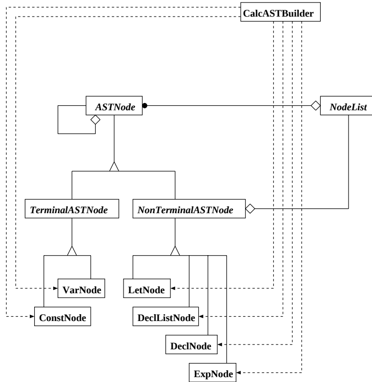
図 5.4: 抽象構文木
