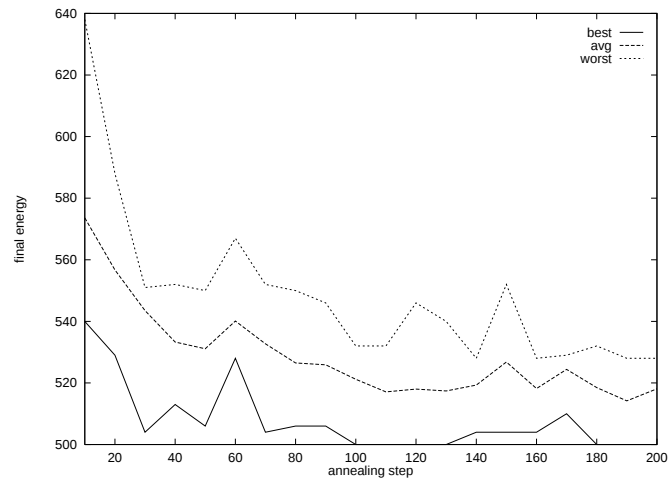
図 4.5: 固定モジュールのみの最良, 平均, 最悪値の推移 (ランダム)
