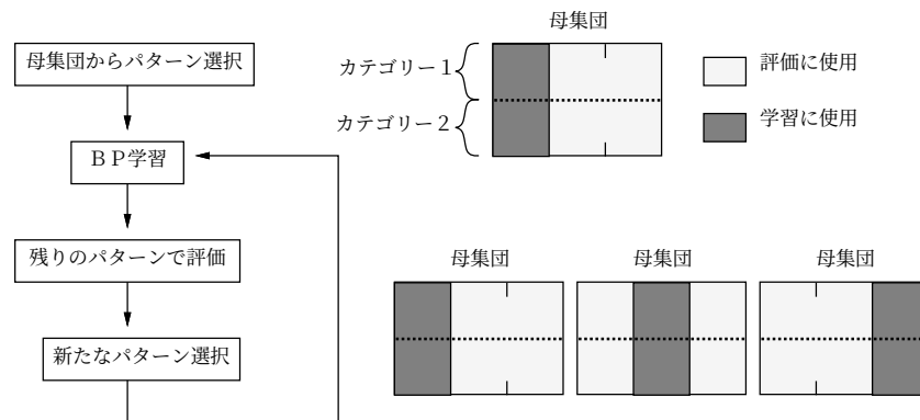
図 3.7: 汎化能力の評価手順
