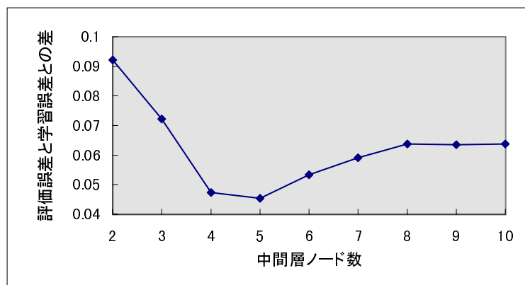
図 3.14: 中間層素子数を変化させた時のクロスバリデーションにおいて取り得る範囲
