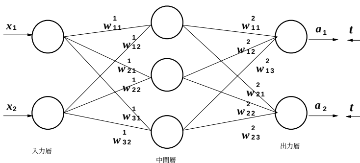
図 2.3: 階層型ネットワークの例
