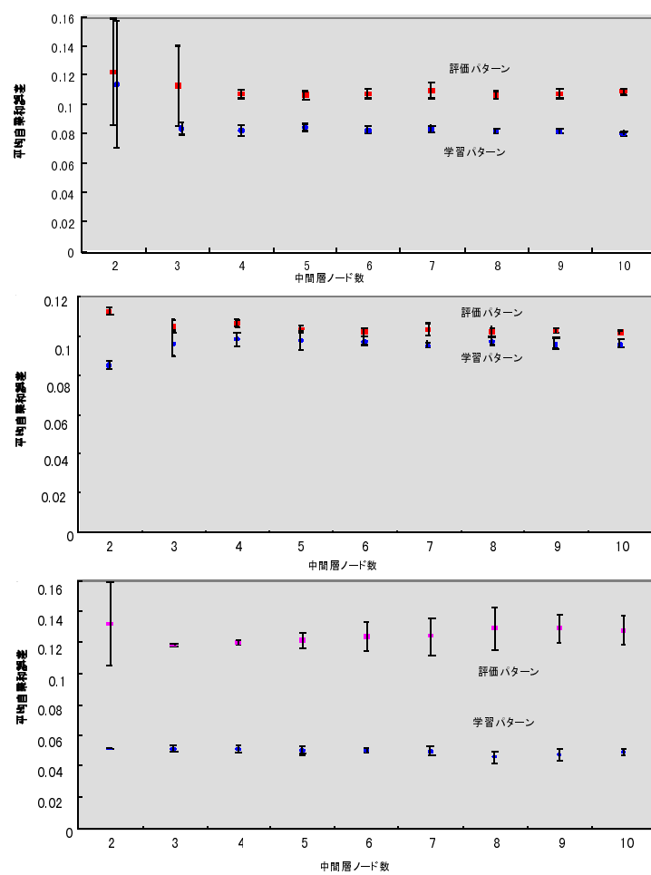
図 3.12: 中間層素子を変化させた時のテストパターンによる汎化能力
