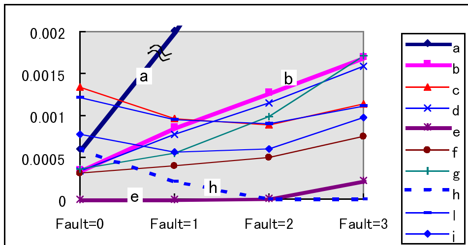
図 4.10: 多重故障（最良NNとの差）
