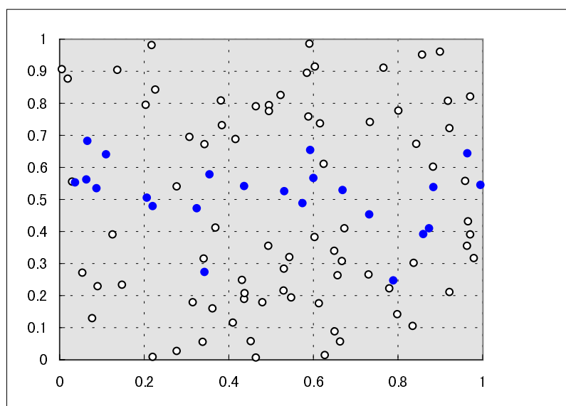
図 2.6: 帯状パターン問題の離散値サンプリング
