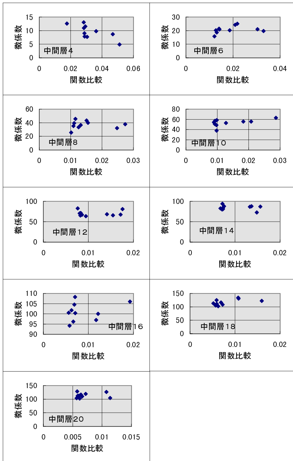
図 6.79: FTBP で帯状パターン連続を学習した時の関数比較に対する中間層の微係数
