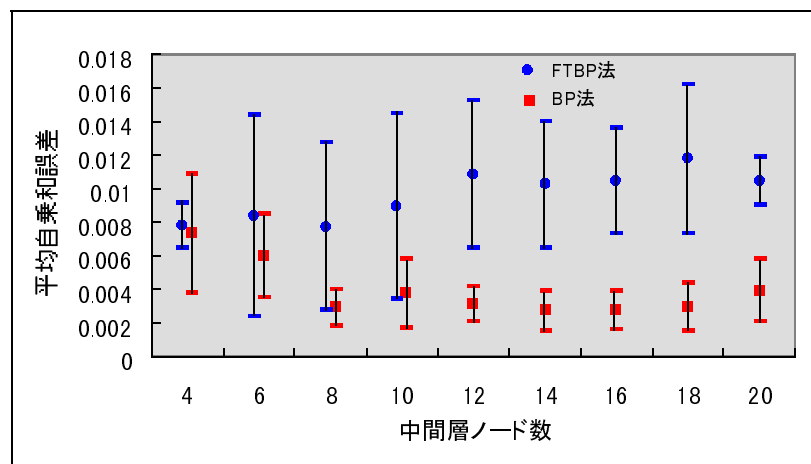
図 5.6: BP 法と FTBP 法の補間能力の比較（帯状パターン連続）
