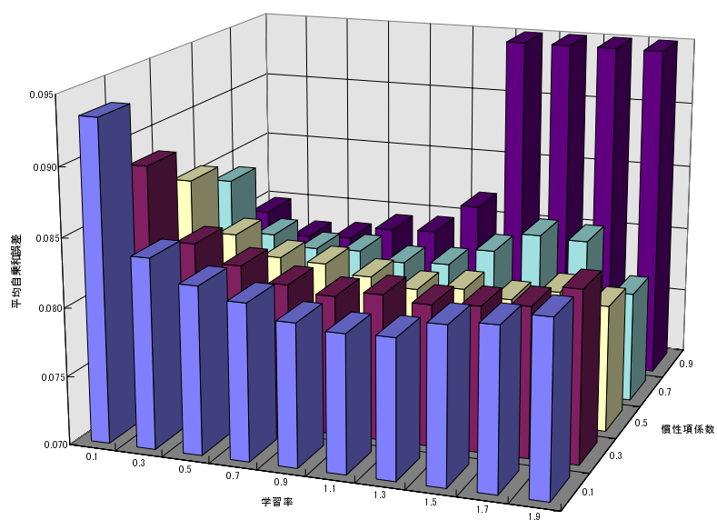
図 4.5: FTBP で帯状パターン離散を学習した時の学習率と慣性項係数
