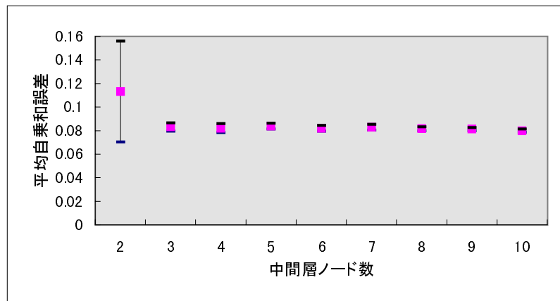
図 3.11: BP で帯状パターン離散を学習した時の平均・標準偏差
