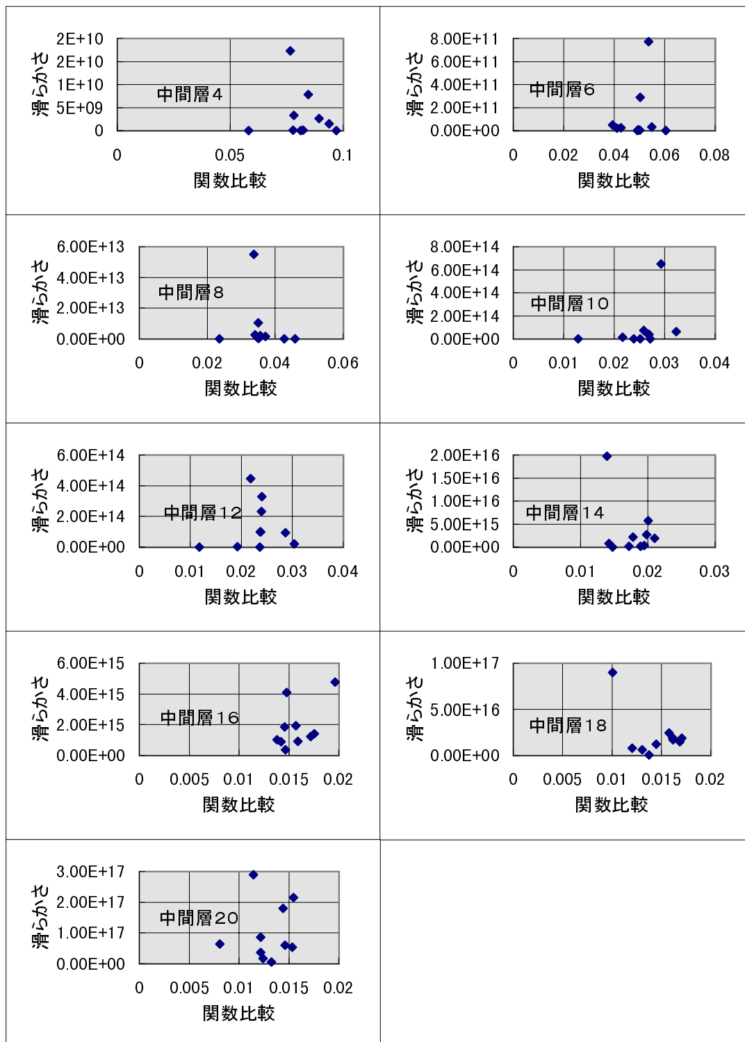
図 6.82: BP で帯状パターン離散を学習した時の関数比較に対する関数の滑らかさ
