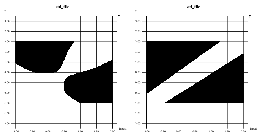
図 3.6: 中間層素子による出力分布
