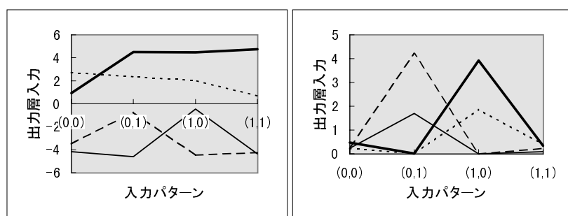
図 3.2: 出力層素子への入力
