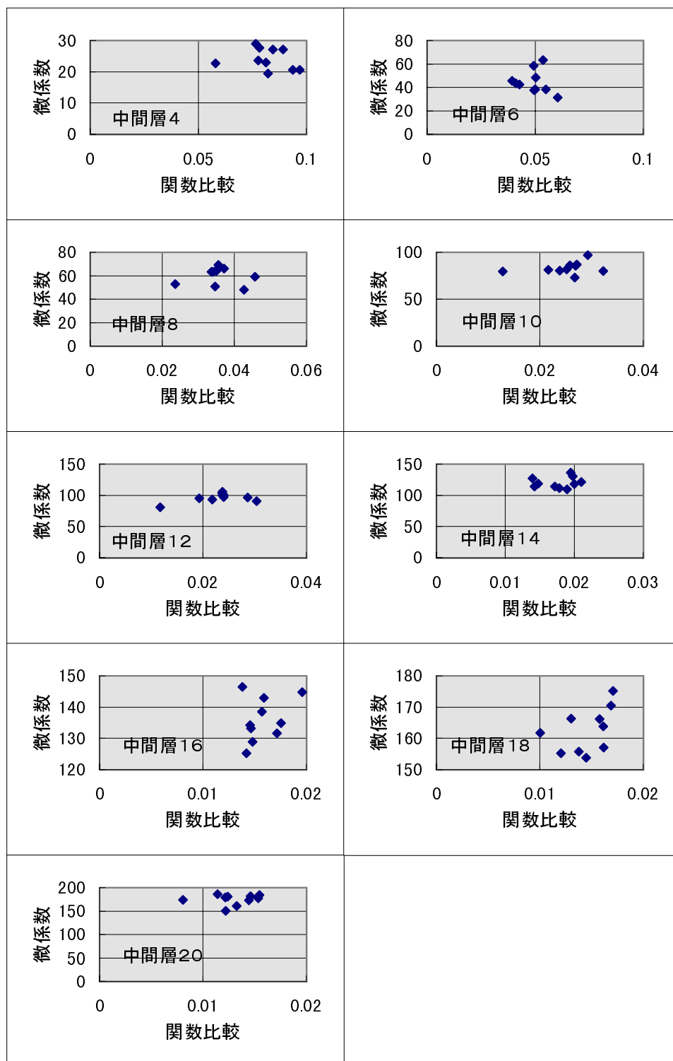
図 6.78: BP で帯状パターン離散を学習した時の関数比較に対する中間層の微係数
