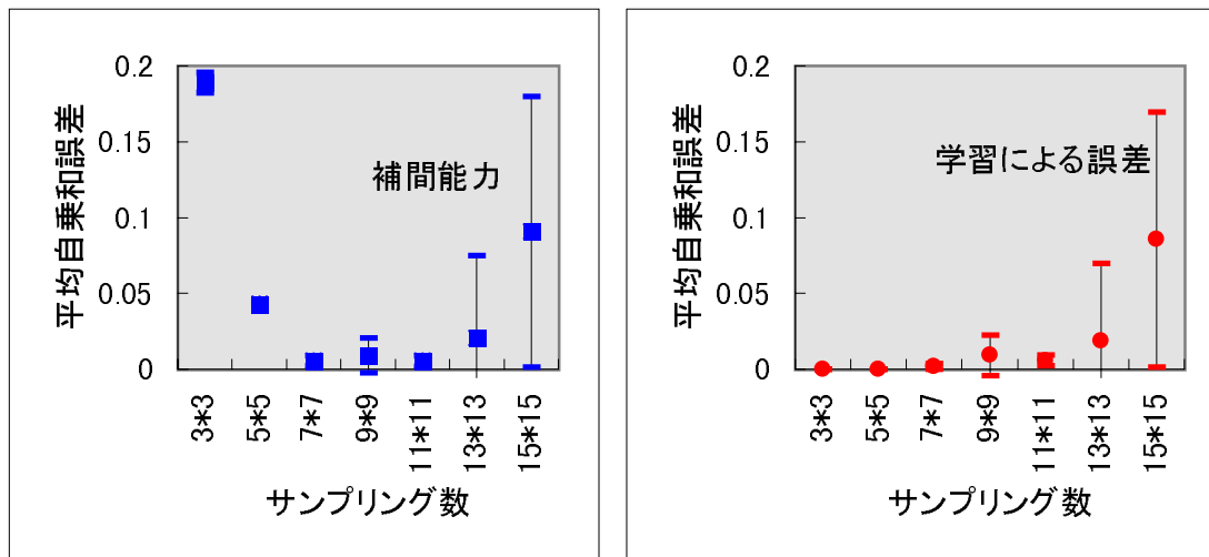
図 3.16: 帯状分布連続のサンプル数に対する補間能力の違い
