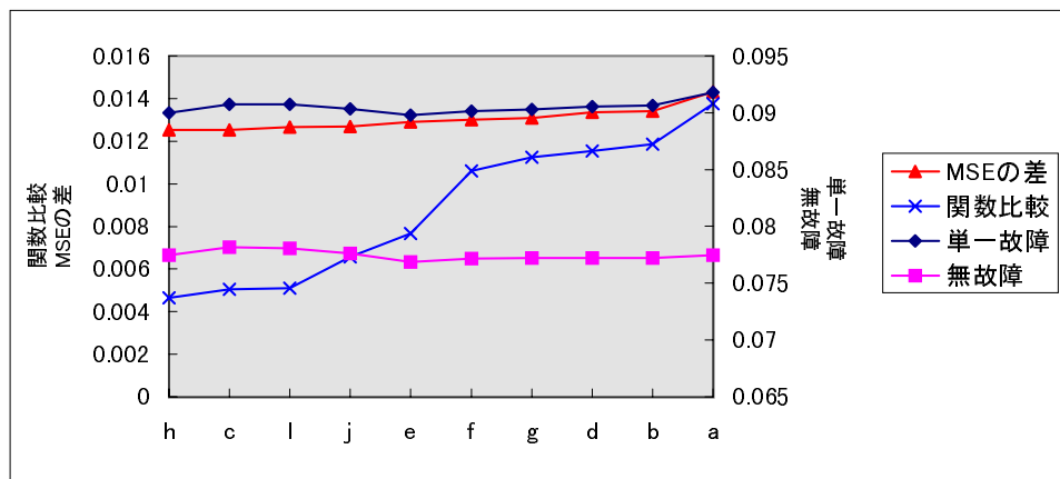
図 4.7: 中間層ノード数 16 の性能評価
