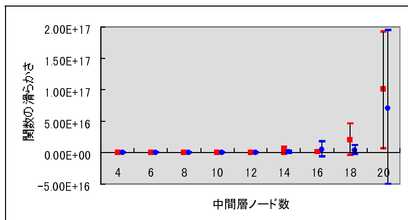
図 5.10: 帯状分布離散を学習した BP と FTBP の関数の滑らかさ
