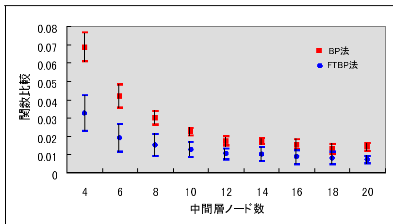
図 5.1: 中間層ノード数を変化させた時の BP と FTBP の関数比較（帯状パターン連続）
