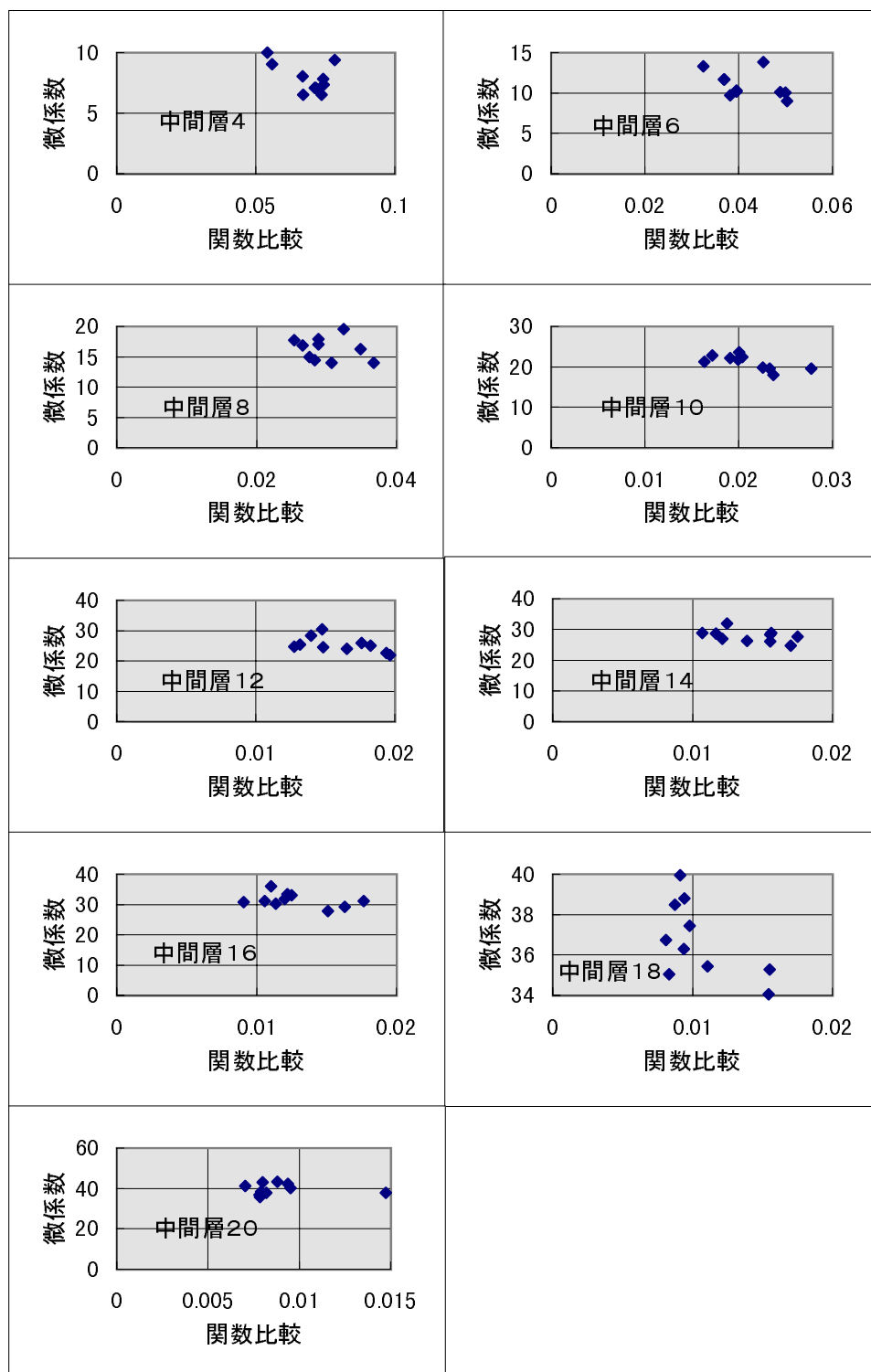
図 6.77: BP で帯状パターン連続を学習した時の関数比較に対する中間層の微係数
