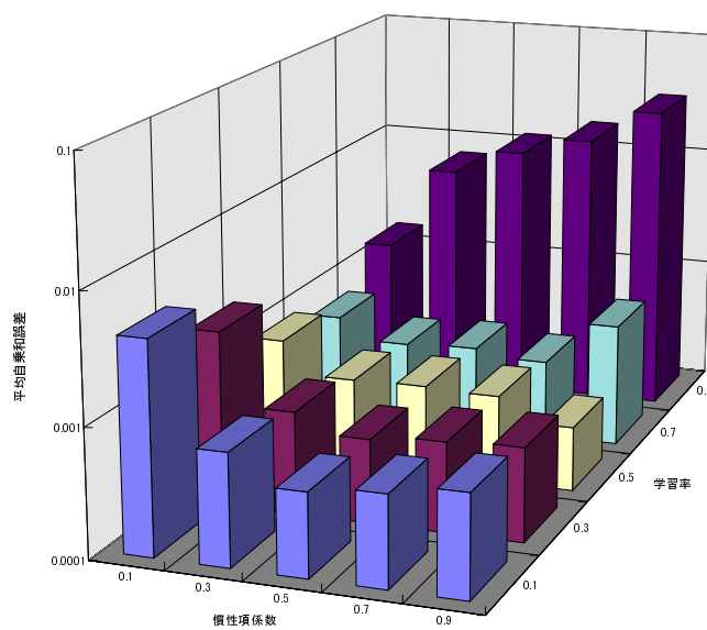
図 4.6: FTBP で帯状パターン連続を学習した時の学習率と慣性項係数
