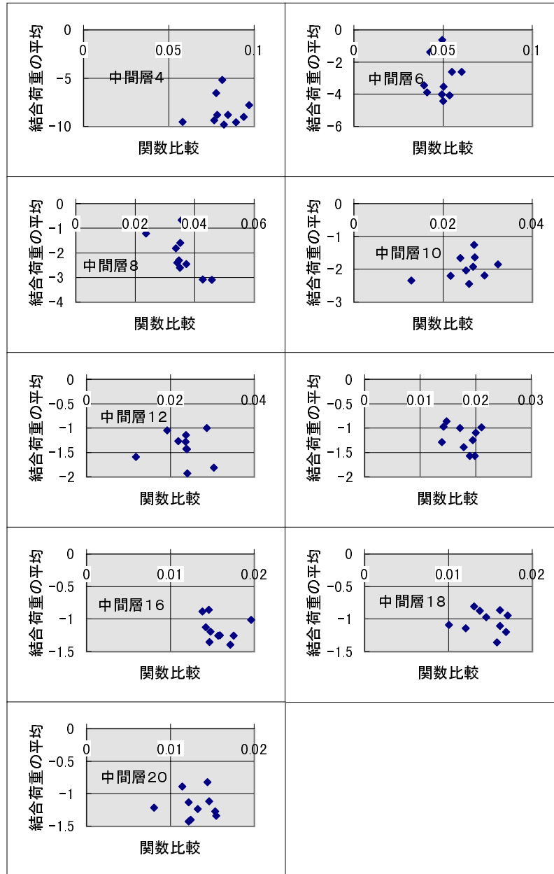
図 6.75: BP で帯状パターン連続を学習した時の関数比較に対する結合荷重
