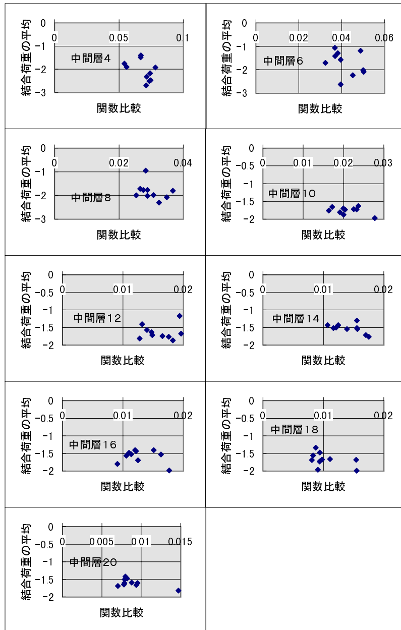
図 6.73: BP で帯状パターン連続を学習した時の関数比較に対する結合荷重
