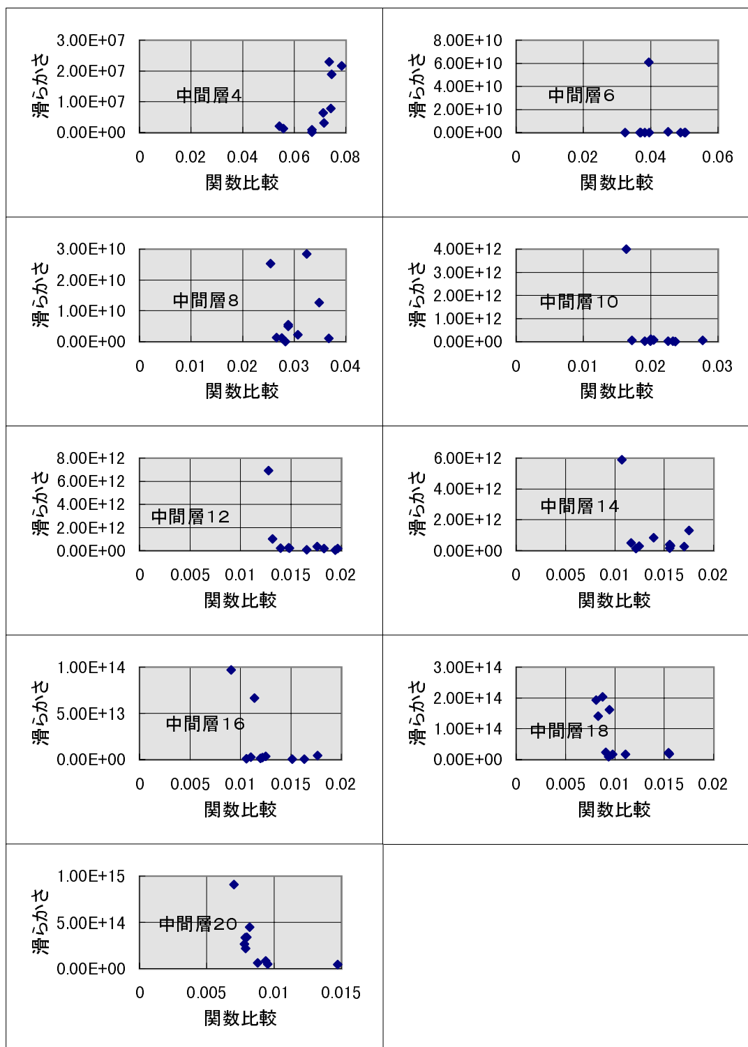
図 6.81: BP で帯状パターン連続を学習した時の関数比較に対する関数の滑らかさ
