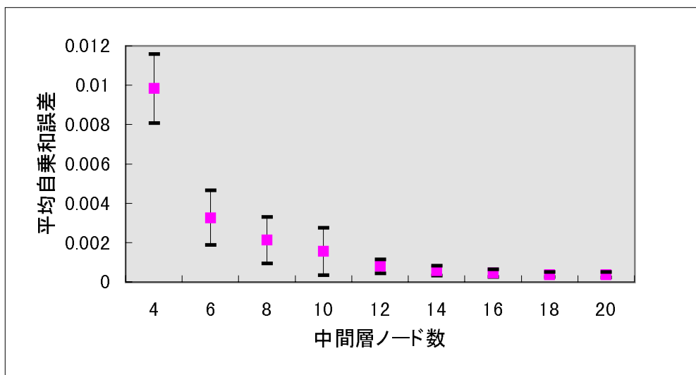
図 4.3: 中間層素子数を変化させて FTBP で帯状パターン連続を学習した時の平均・標準偏差
