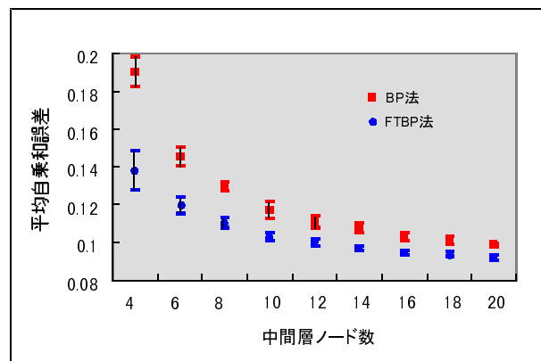
図 5.4: 単一断線故障を発生させた時の BP と FTBP の自乗和誤差（帯状パターン離散）
