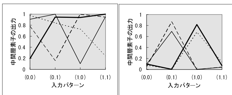
図 3.1: 中間層素子の出力
