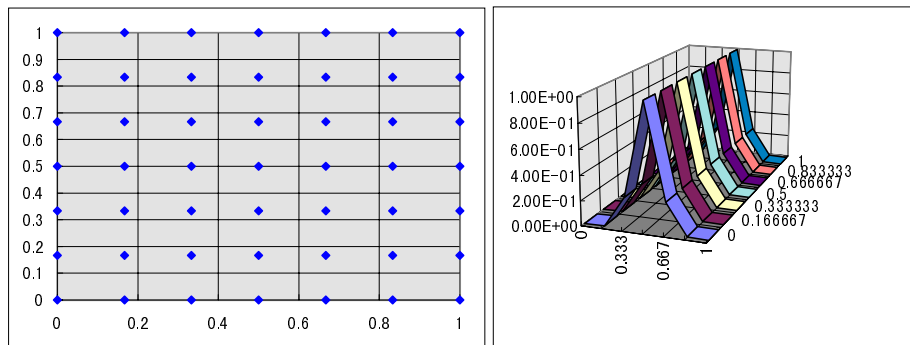
図 2.5: 帯状パターン問題の連続値サンプリング
