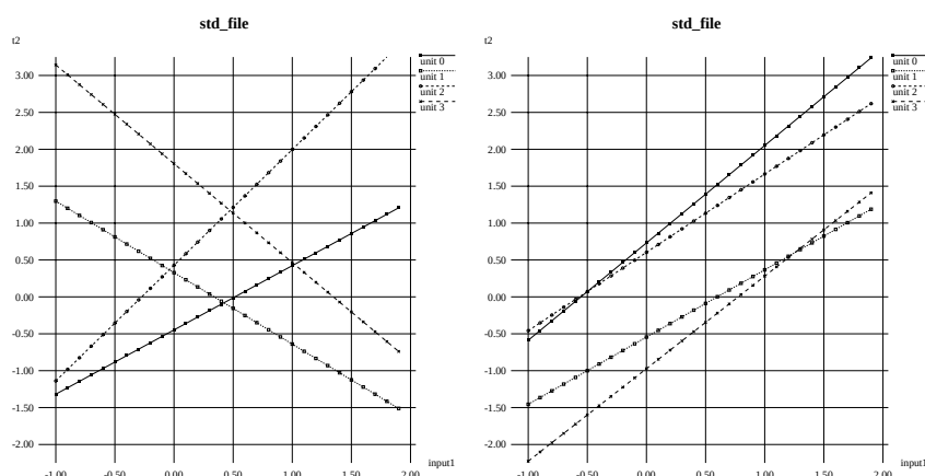
図 3.5: 中間層素子による分離直線
