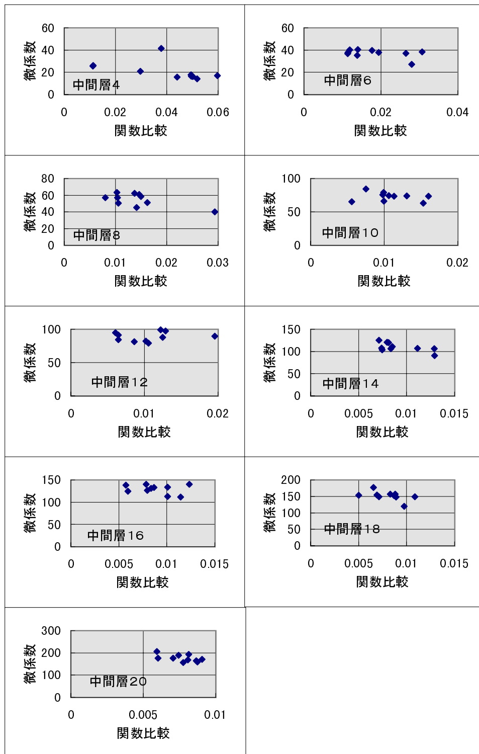
図 6.80: FTBP で帯状パターン離散を学習した時の関数比較に対する中間層の微係数
