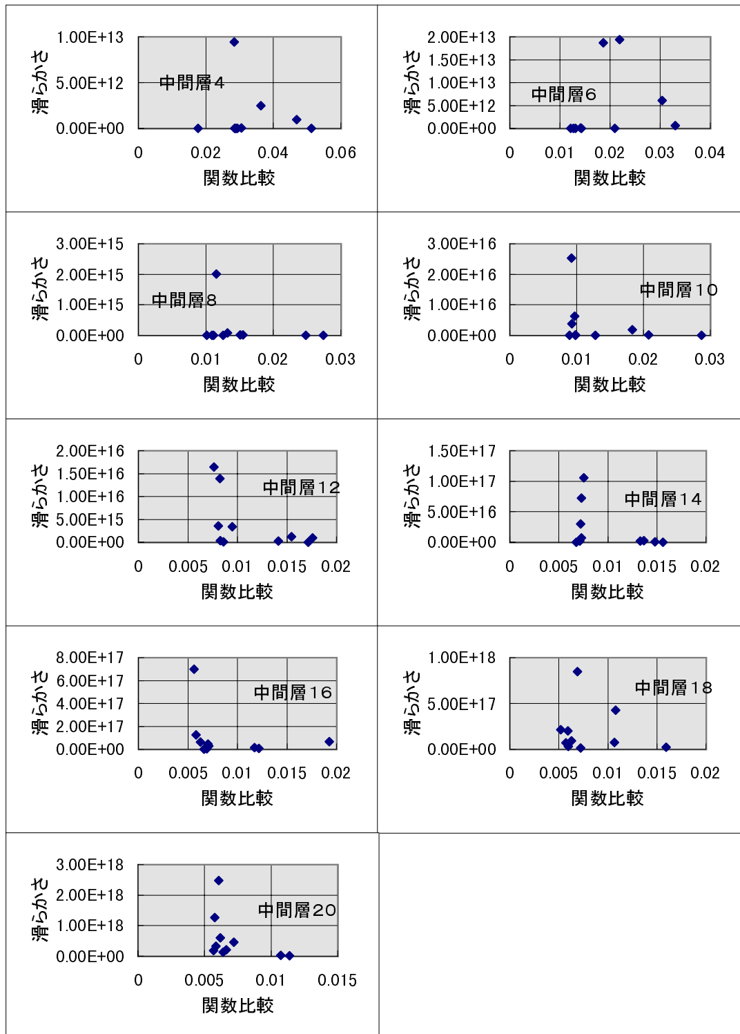
図 6.83: FTBP で帯状パターン連続を学習した時の関数比較に対する関数の滑らかさ
