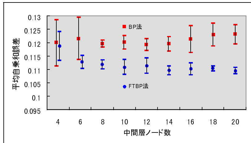
図 5.5: BP 法と FTBP 法の汎化能力の比較（帯状パターン離散）
