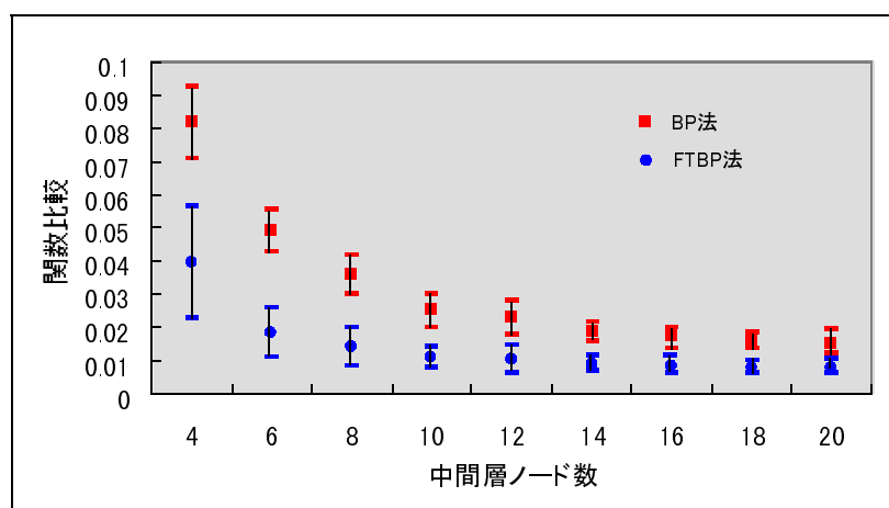
図 5.2: 中間層ノード数を変化させた時の BP と FTBP の関数比較（帯状パターン離散）
