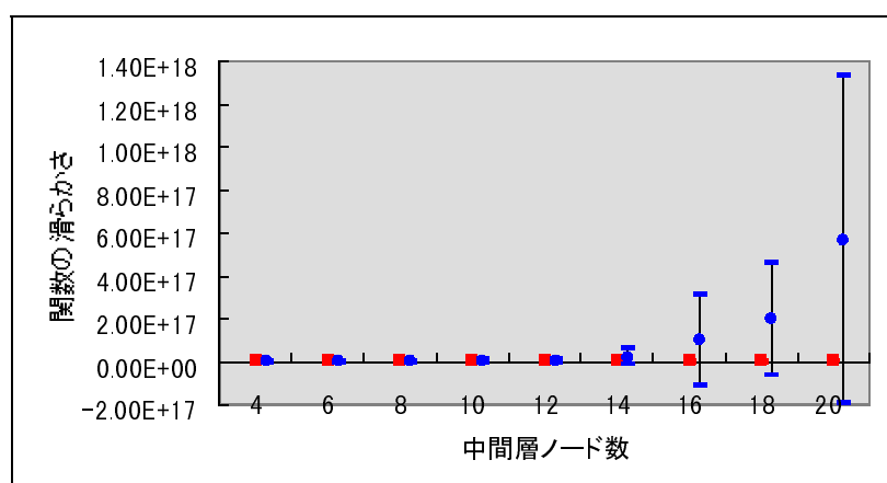
図 5.11: 帯状分布連続を学習した BP と FTBP の関数の滑らかさ
