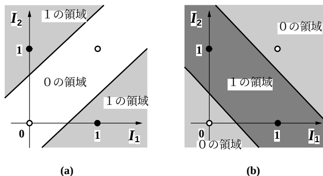
図 3.4: XOR の分離直線
