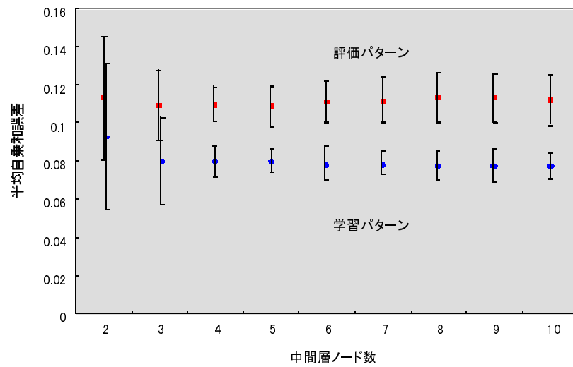
図 3.13: 中間層素子を変化させた時のクロスバリデーションによる汎化能力
