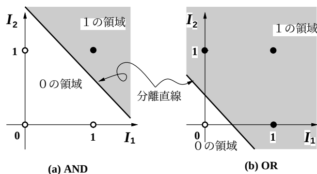
図 3.3: 中間層素子出力による分離直線の例
