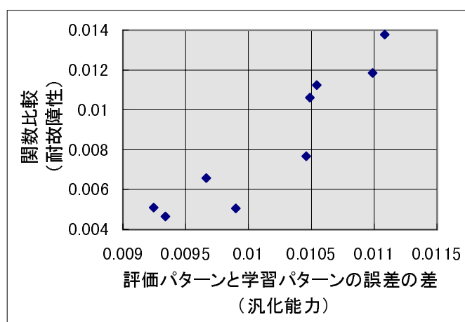
図 5.7: 同じ中間層を持つネットワークの耐故障性と汎化能力
