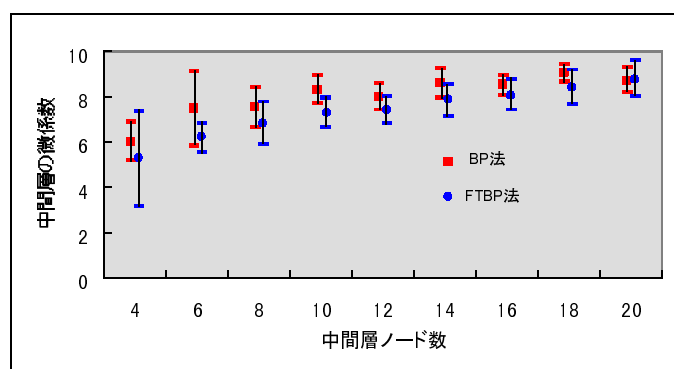
図 5.8: 帯状分布離散を学習した BP と FTBP の中間層素子の微係数
