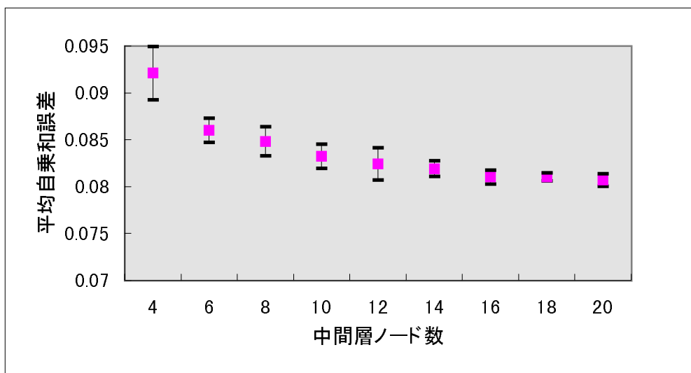
図 4.4: 中間層素子数を変化させて FTBP で帯状パターン離散を学習した時の平均・標準偏差
