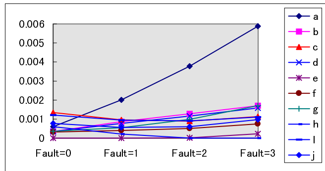
図 4.9: 多重故障（最良NNとの差）
