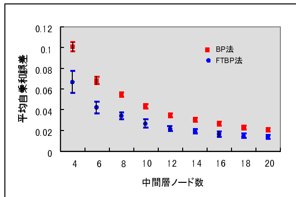
図 5.3: 単一断線故障を発生させた時の BP と FTBP の自乗和誤差（帯状パターン連続）
