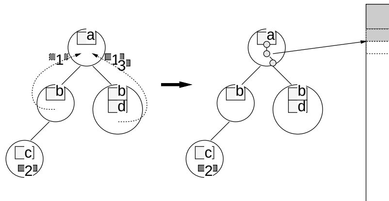
図 5.7: 分岐コードの生成
