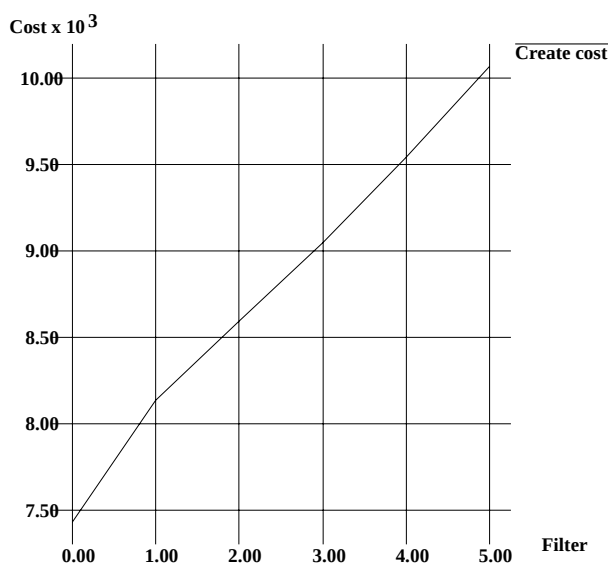
図 6.6: フィルタ数に対するモジュール生成コスト
