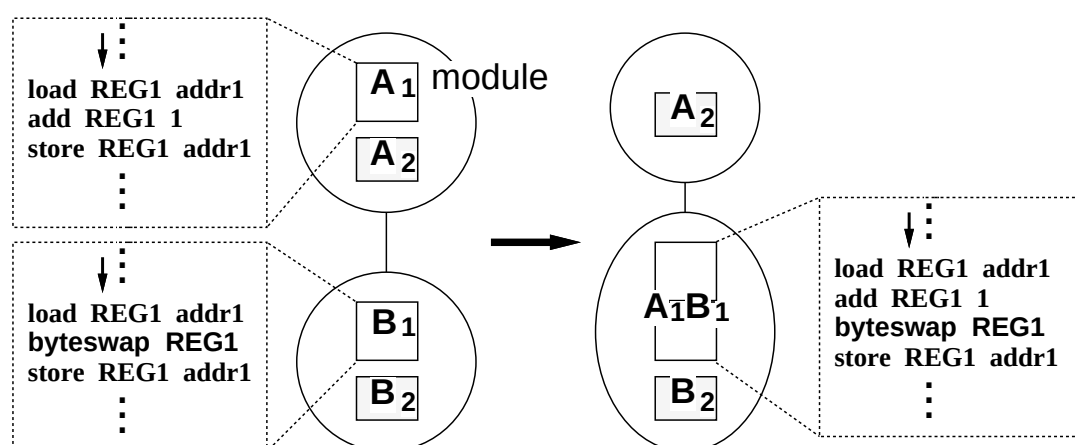
図 4.1: load/store の削減
