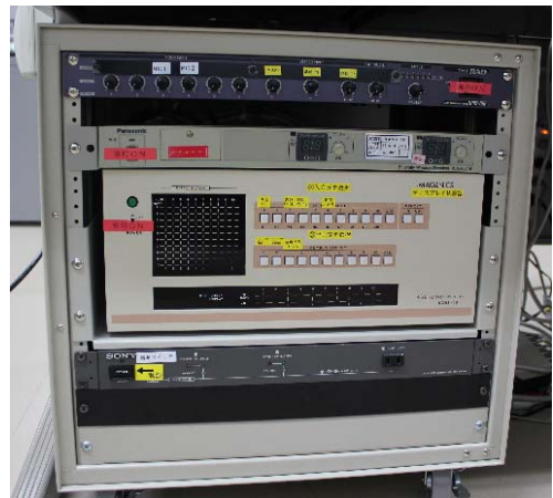
図 5. マイク受信機を設置したラック
