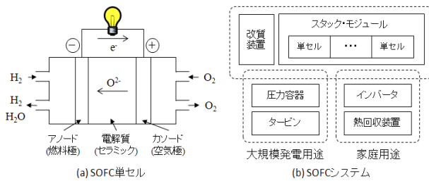
図 6 SOFC 概念図
