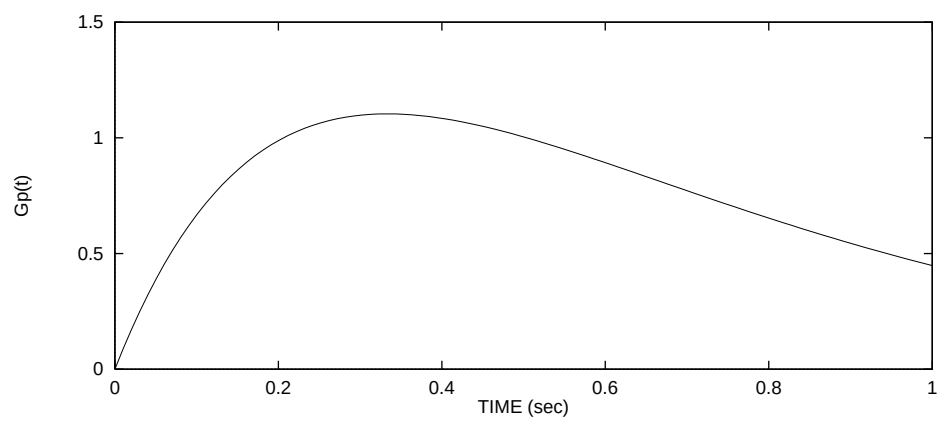
(a) フレーズ成分 G_p(t) ( \alpha = 3.0 \text{ s}^{-1} )
