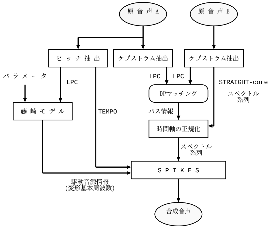
図 2.1: 音声合成系
