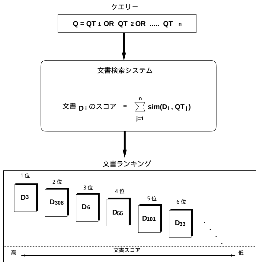
図 2.2: 文書検索システムの概観
