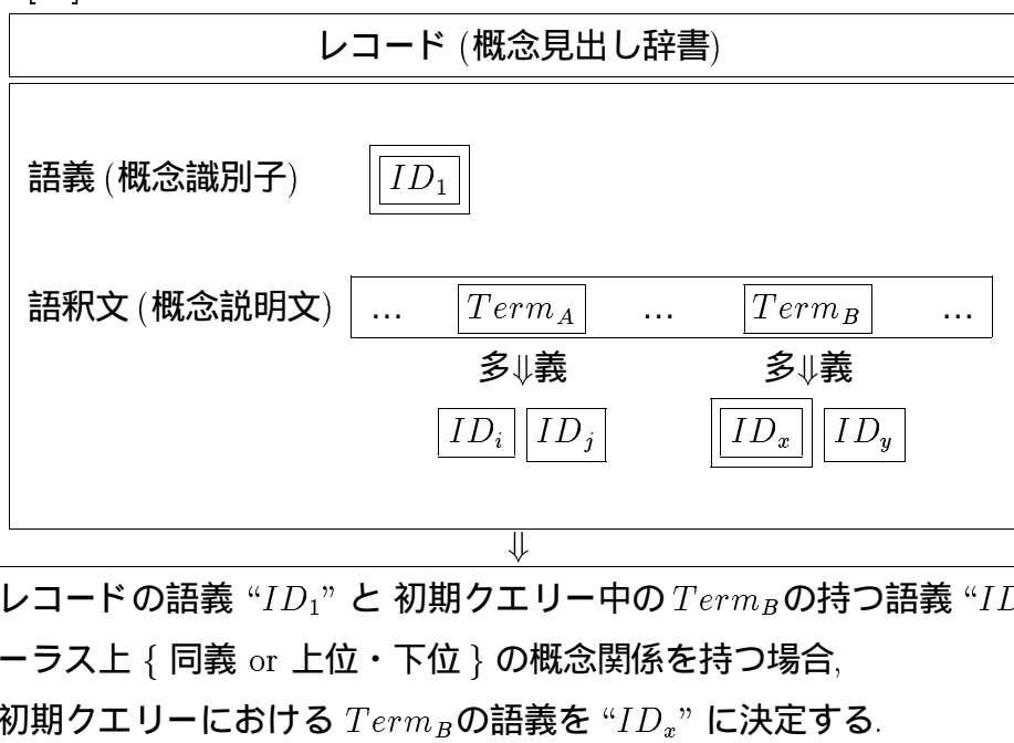
図 5.2: 語釈文とシソーラスを利用した語義の曖昧性の解消方法
