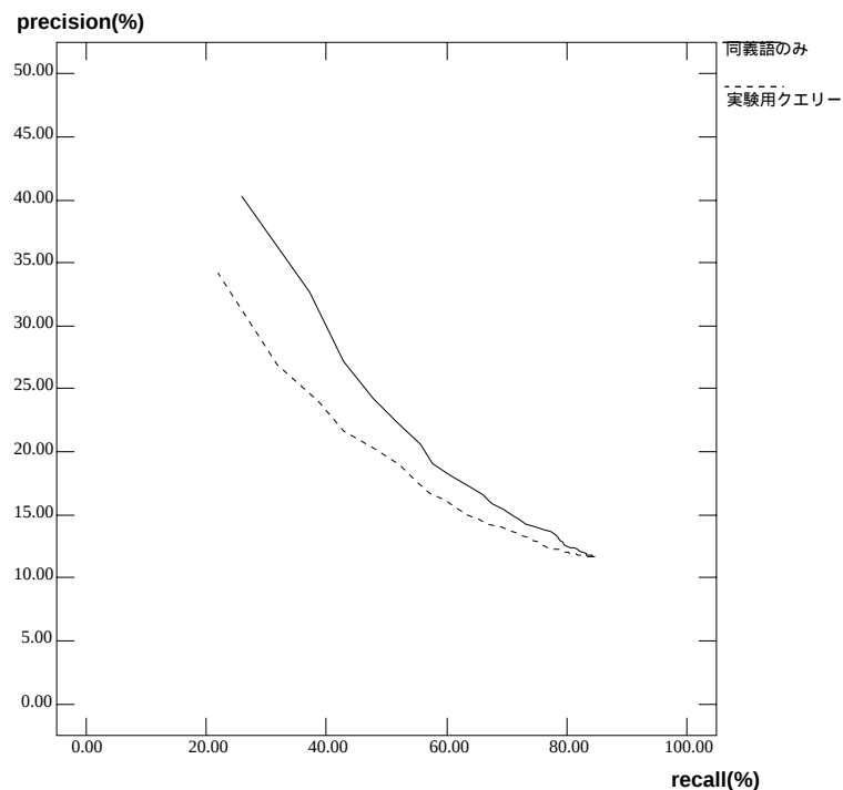
図 6.2: 実験 (1) の結果 (クエリーセット “B”)
