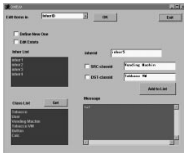
図 5.9: 継承関係編集 GUI
