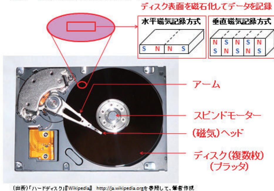
図1 垂直磁気記録方式ディスクの開発
