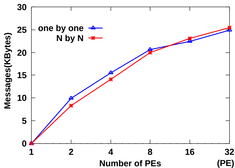
図 4.18: マスタスレーブ型における総メッセージ通信データ量
