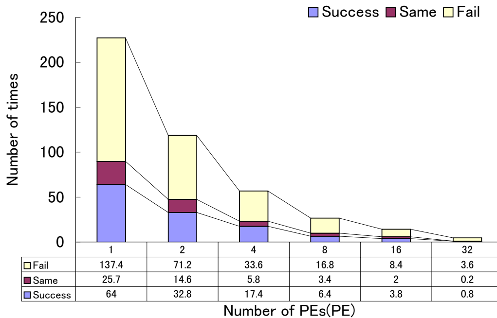
図 4.19: マスタスレーブ型における TSP の実行回数 (one by one)
