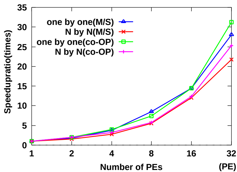
図 4.29: マスタースレーブ型と協調型の速度向上比
