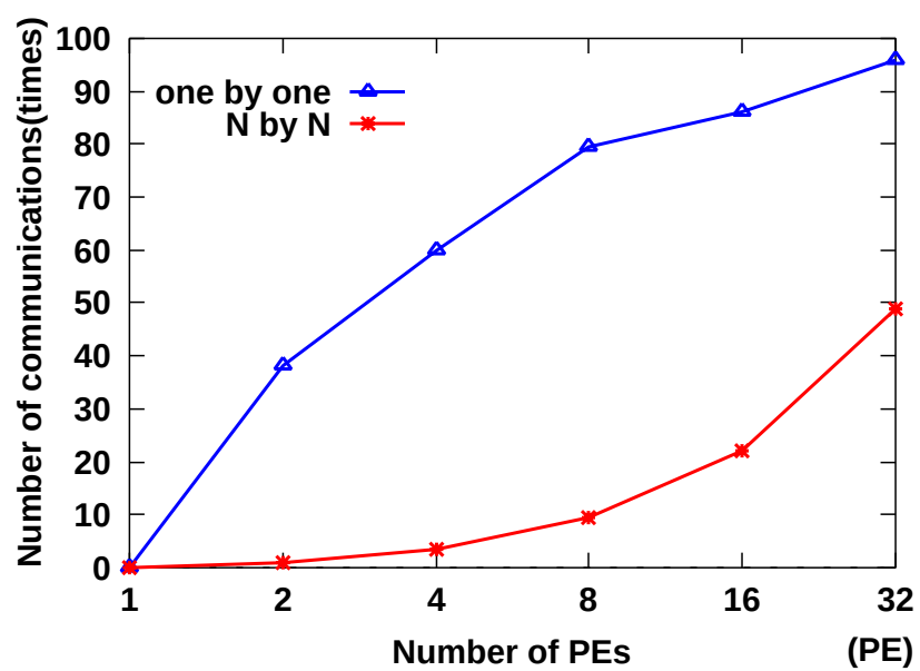
図 4.17: マスタースレーブ型における総メッセージ通信回数
