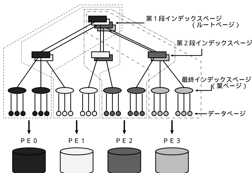
図 1: Fat-Btree 構造
