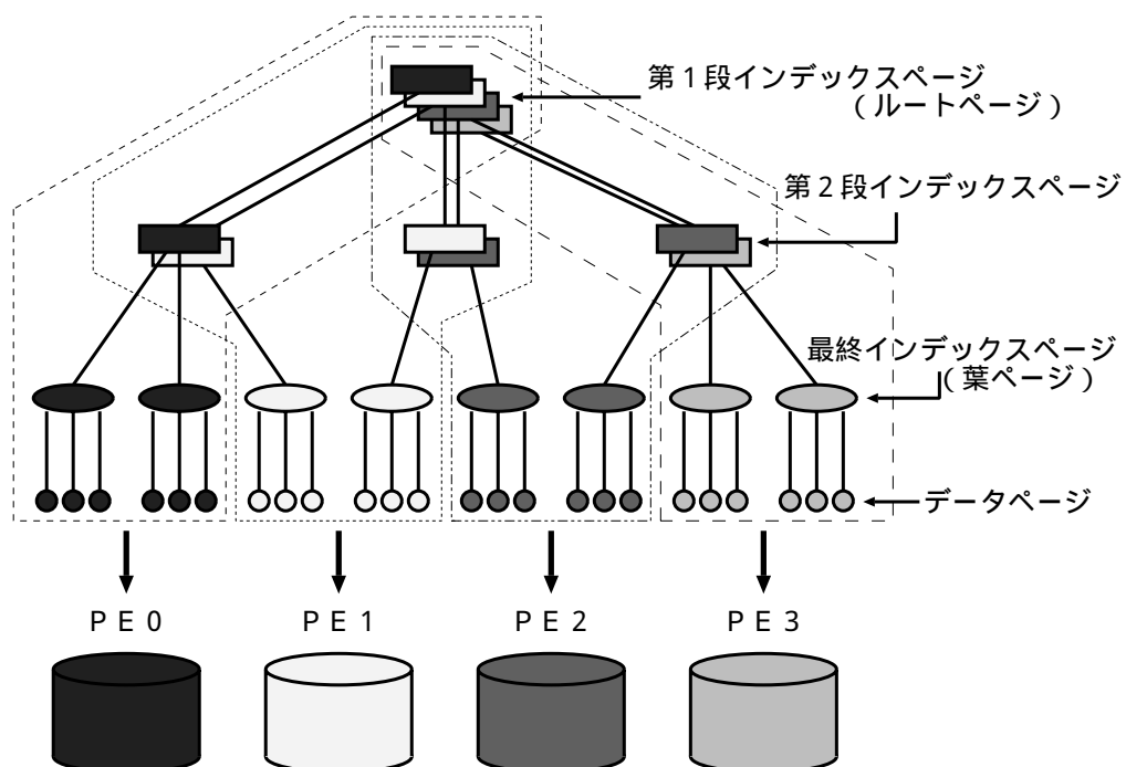
図 3.1: Fat-Btree 構造
