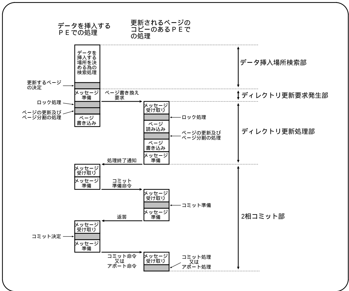
図 A.1: WRITE 処理の流れ ( Inv = 1 の場合)
