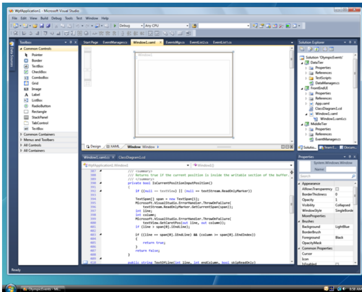
図 6 Visual Studio
