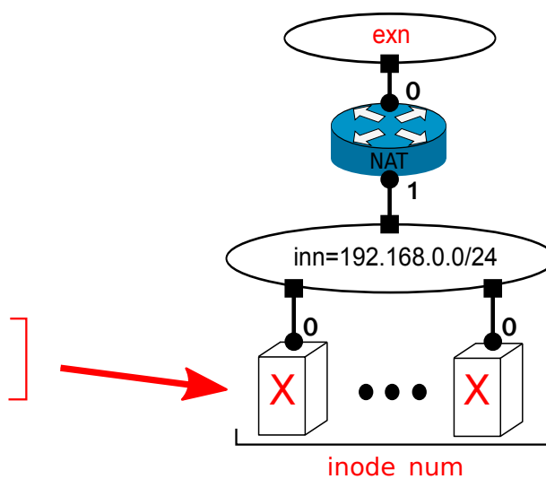
図 4.11: Abstract_NAT Dodule script
