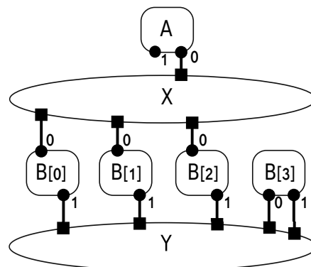
図 4.7: ネットワーク記述と構成
