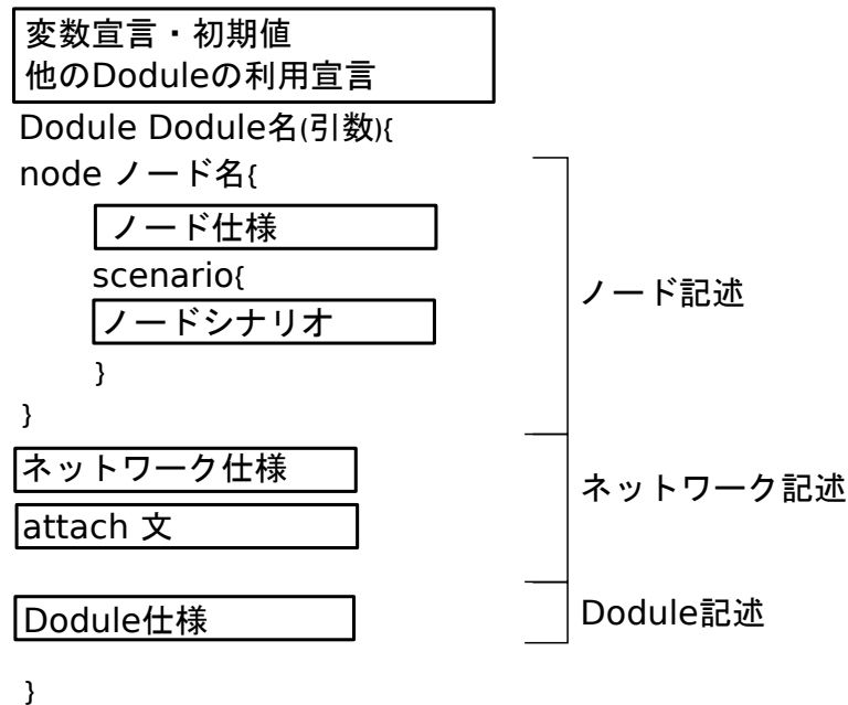
図 4.8: Dodule script
