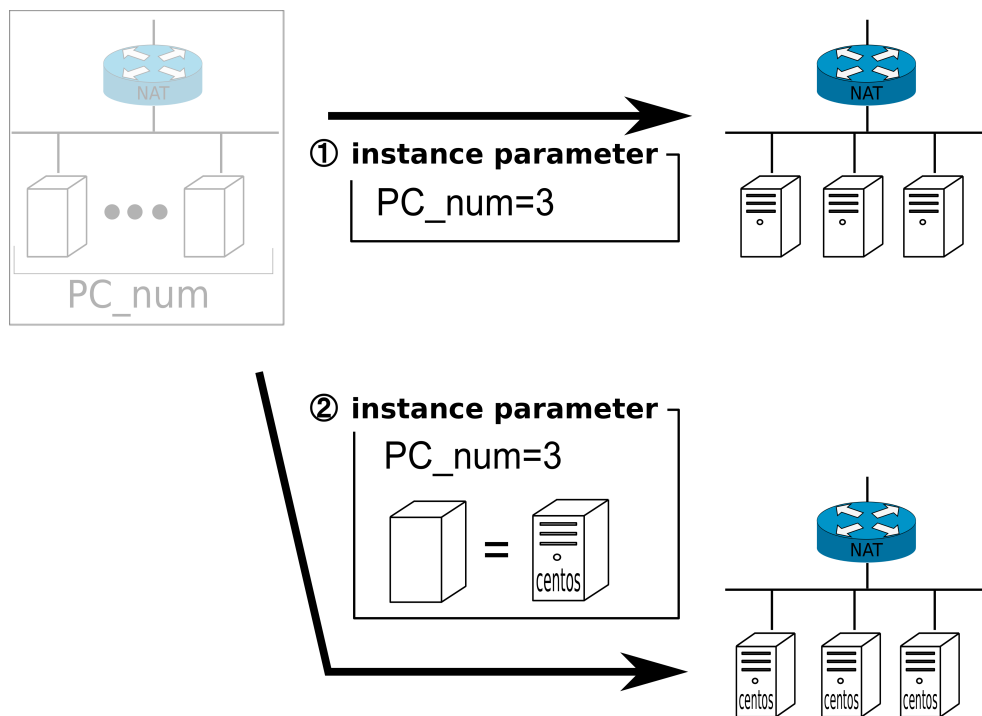
図 4.4: コンストラクタによる初期値
