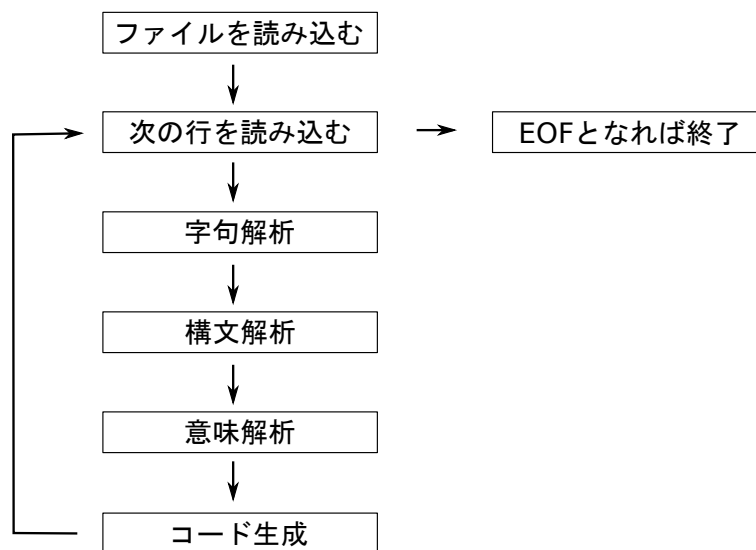
図 4.14: MKt の処理の流れ
