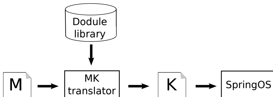
図 4.13: 本システムの構成
