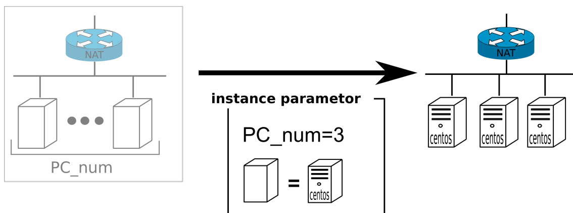
図 4.3: Module のパラメータ
