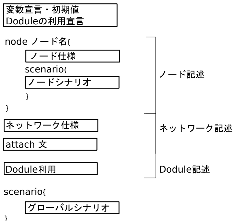
図 4.6: スクリプトの骨組み
