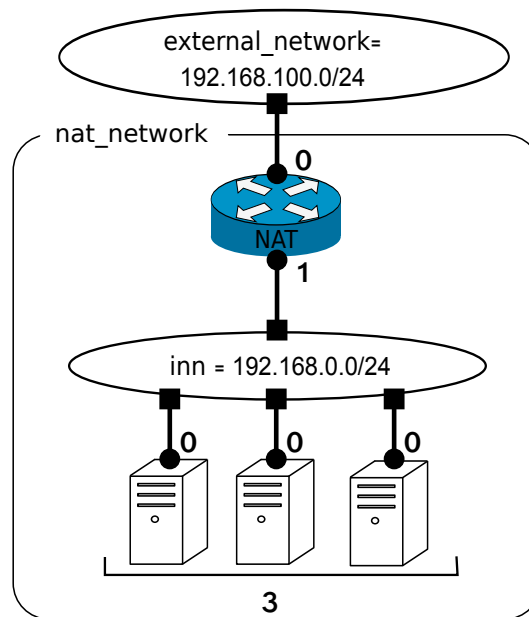
図 4.10: Standard_NAT のインスタンス化の例
