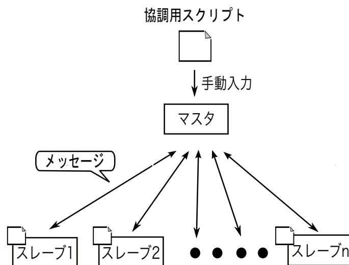
図 2.2: マスタ・スレイブ間のメッセージ交換
