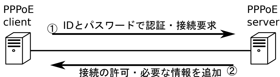
図 5.3: PPPoE の流れ
