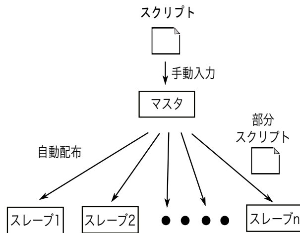
図 2.1: マスタ・スレイブモデル
