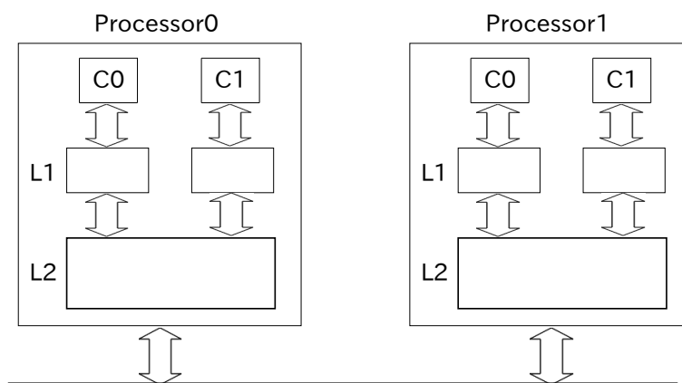
図 4.1: 2 コア・2 プロセッサ構成
