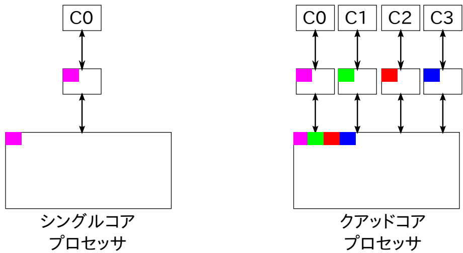
図 3.1: Inclusion Property 方式
