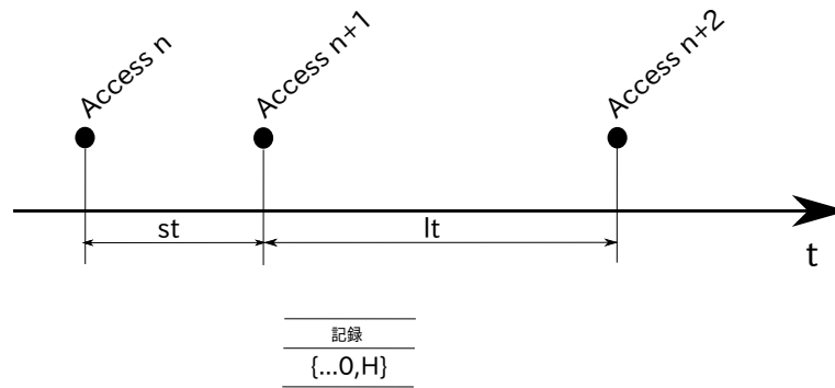
図 2.4: L1 Long term access の記録の例
