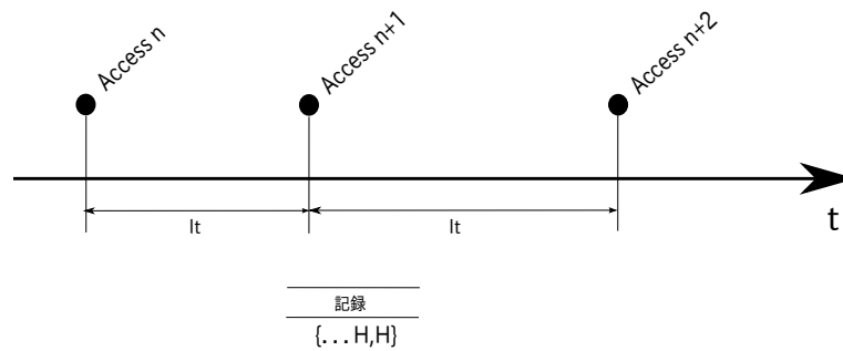
図 2.2: L1 Long term access の記録の例
