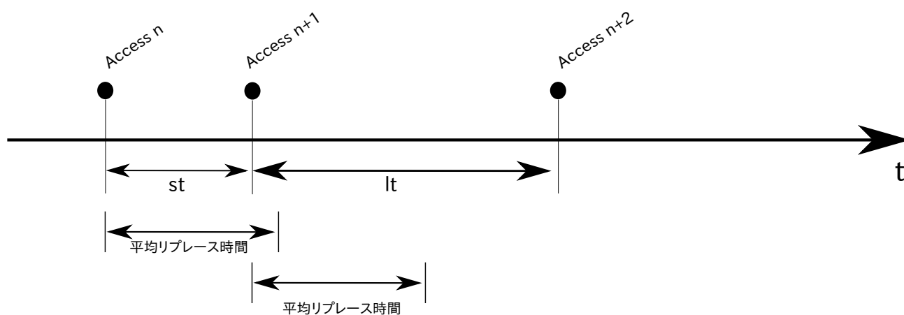
図 3.3: メモリアクセス間隔との比較による問題
