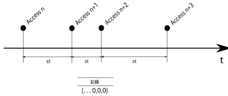
図 2.1: L1 Short term access の記録の例
