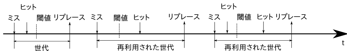
図 3.7: ステップ 2 のブロック
