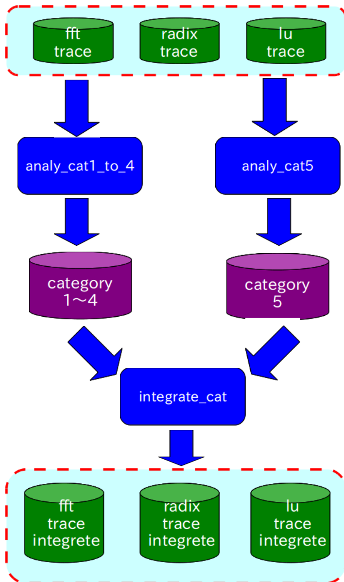
図 4.6: カテゴリファイル出力
