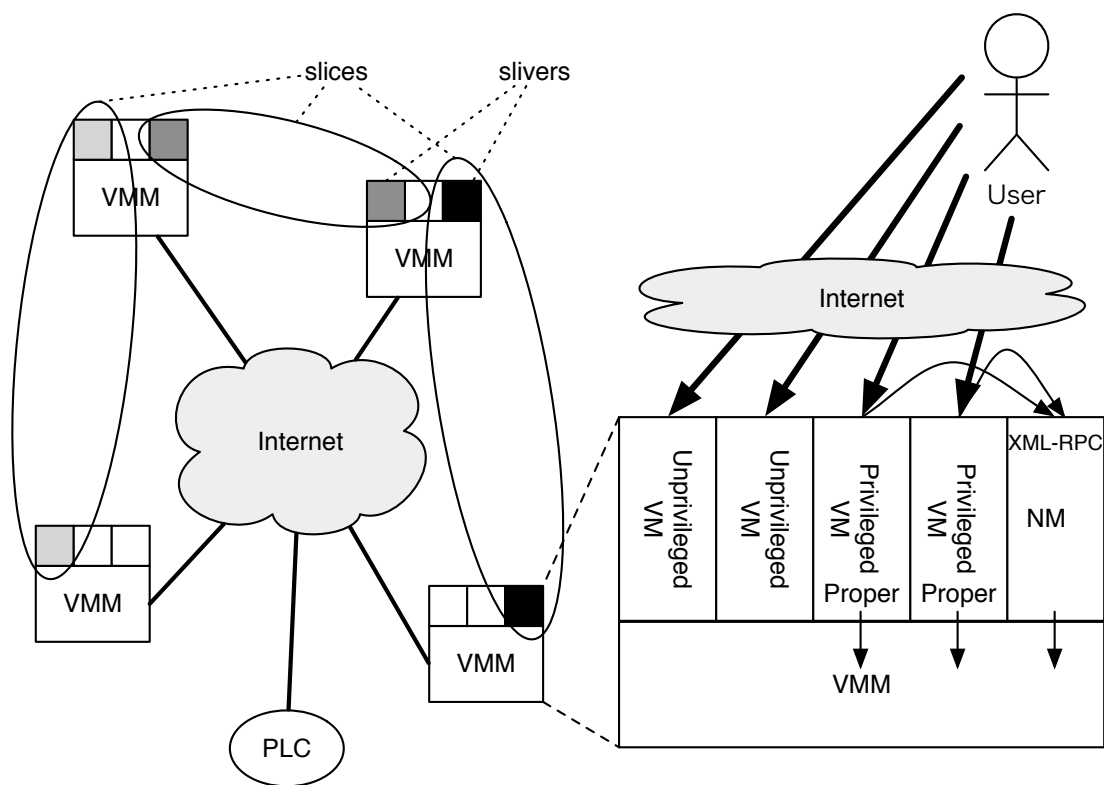
図 2.2: planetlab の概要
