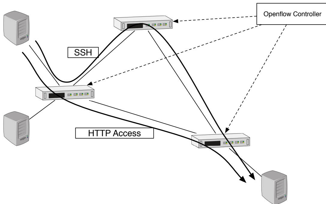
図 5.4: OpenFlow の動作
