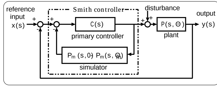
図 3.2: MIMO Smith method.
