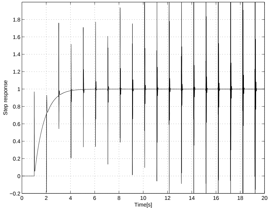
図 4.2: u=0.01 の場合のシステム
