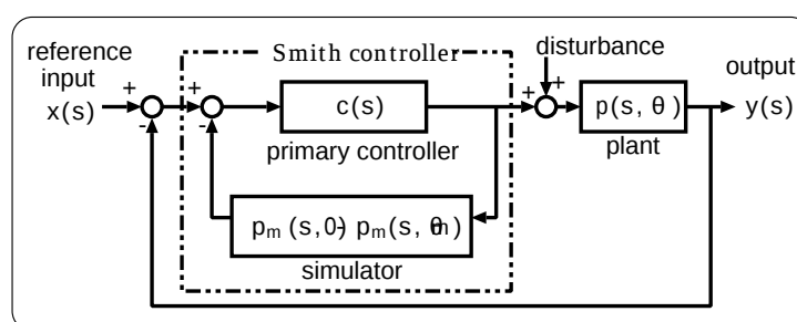
図 3.1: SISO Smith method.
