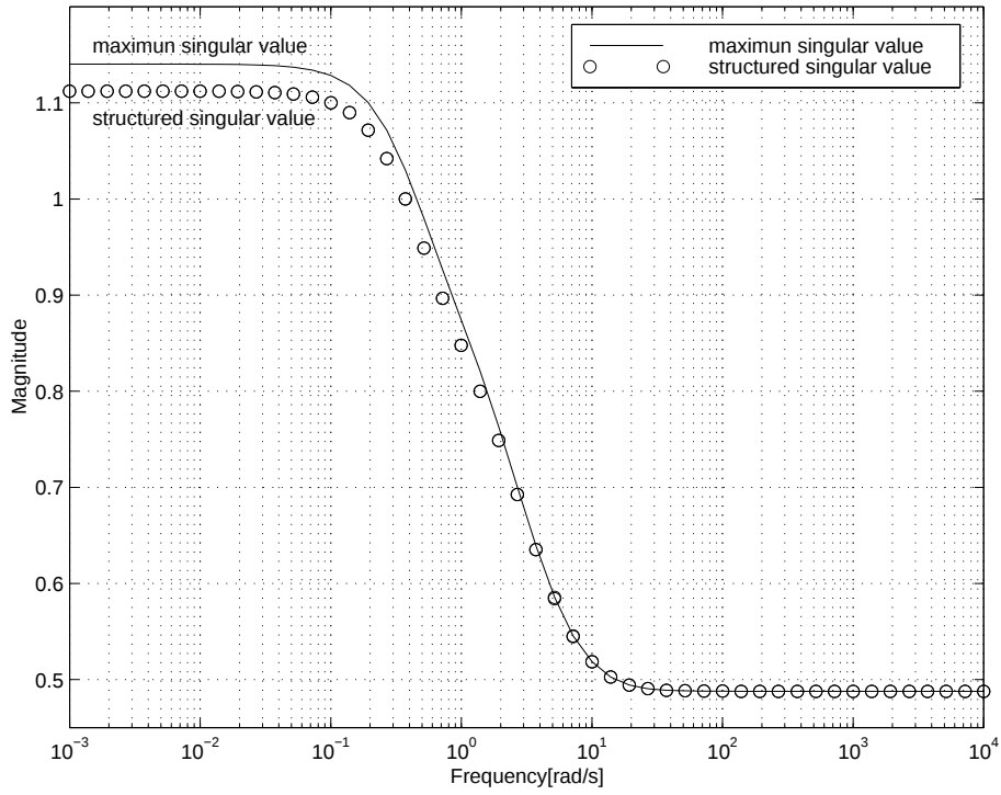
図 6.2: \mu_{\Delta}(M(j\omega)) and \bar{\sigma}(M(j\omega)) .
