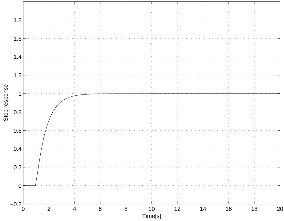
図 4.1: u=0 の場合のノミナルシステム
