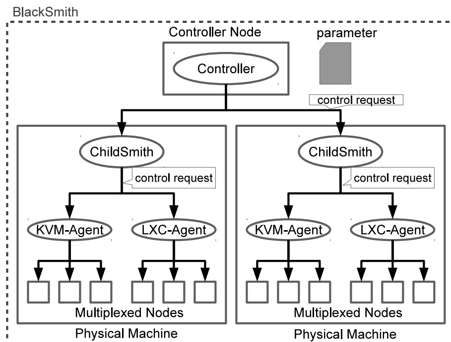
図 5.2: BlackSmith の全体構成
