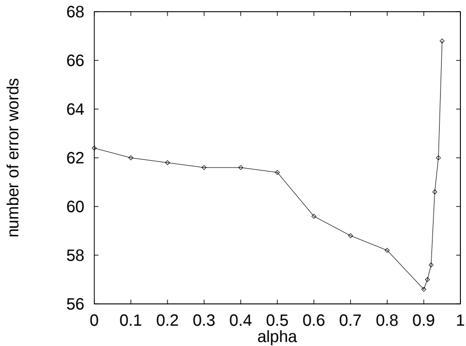
図 4.5: 評価データ 5 話者 (m116 ~ m120) の平均誤認識単語数の変化による結合係数 \alpha の決定 ( \text{SNR}_{45\text{dB}} )
