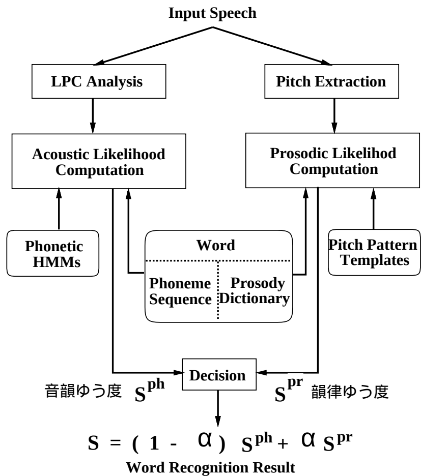
図 2.1: 韻律情報を用いた認識システムの構成
