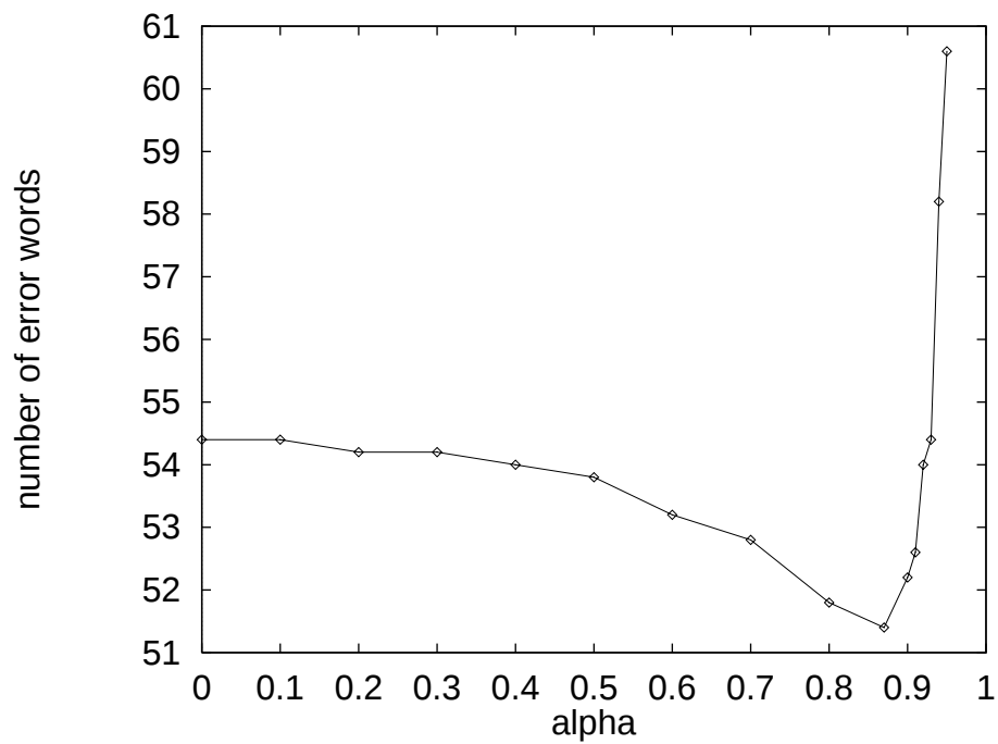
図 4.4: 評価データ 5 話者 (m116 ~ m120) の平均誤認識単語数の変化による結合係数 \alpha の決定 ( \text{SNR}_{\infty} )
