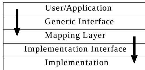
図 3.1: トレードオフを記述するためのフレームワーク
