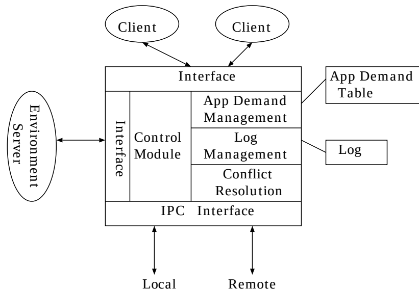
図 4.2: DOマネージャの構成
