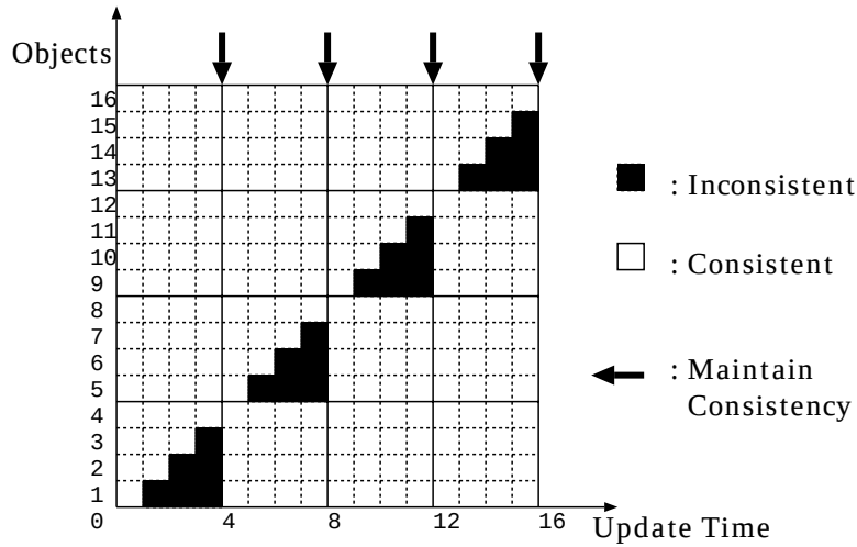
図 6.1: 一貫性維持度の算出方法
