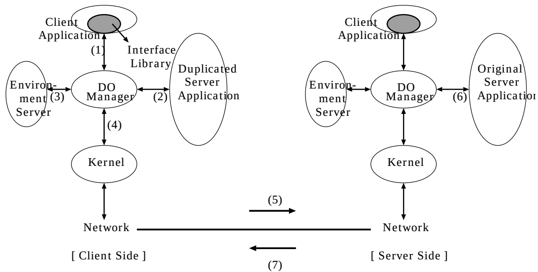
図 4.1: ツールキットの構成
