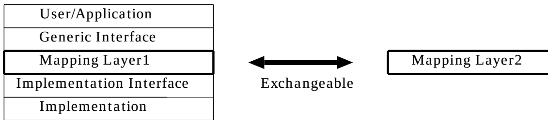
図 3.5: 交換可能なマッピングレイヤー
