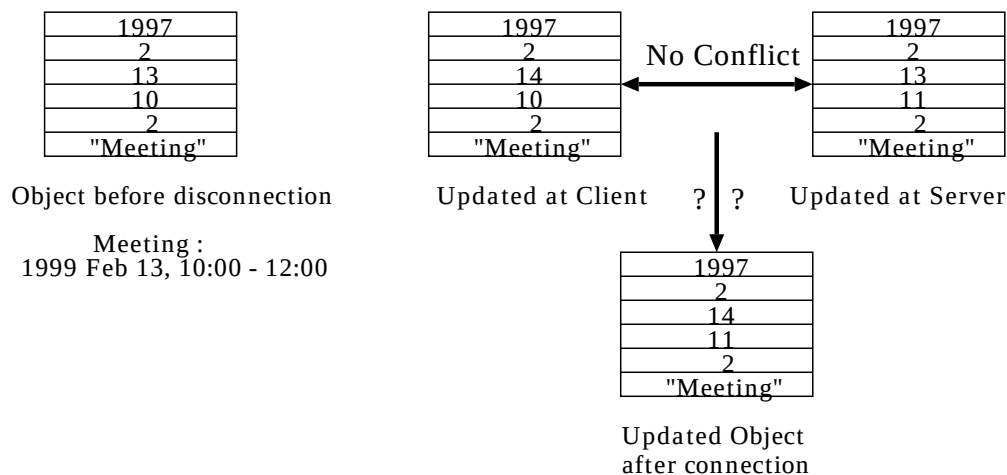
図 4.7: 同一オブジェクト内の競合
