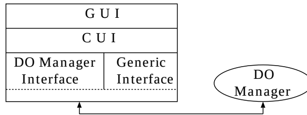
図 4.4: クライアントアプリケーションの構成
