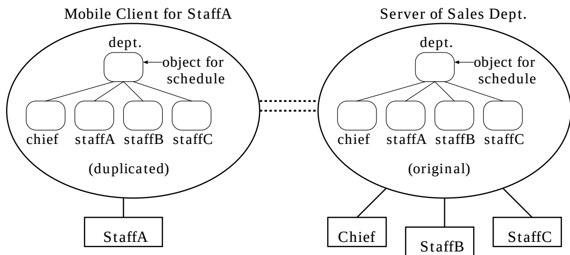
図 5.1: グループスケジューラの構成
