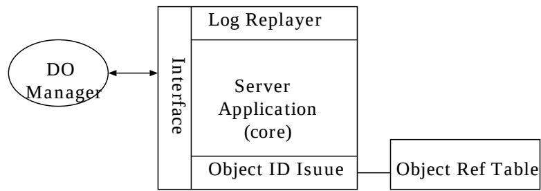
図 4.3: サーバアプリケーションの構成
