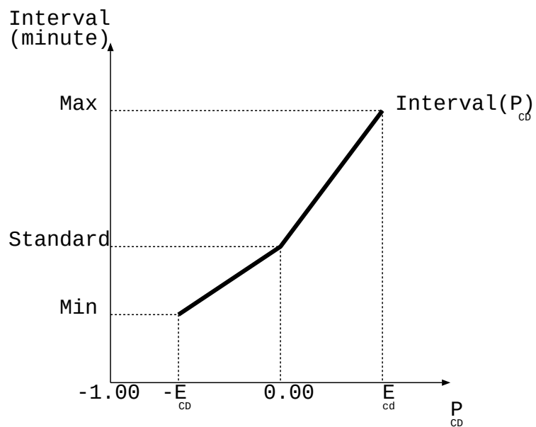
図 3.4: 接続間隔時間決定関数
