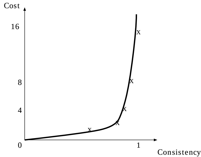
図 6.2: 通信コストと一貫性維持度の相関関係
