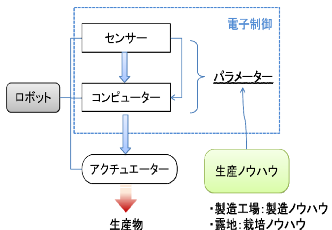
図1 植物工場等のロボット化
