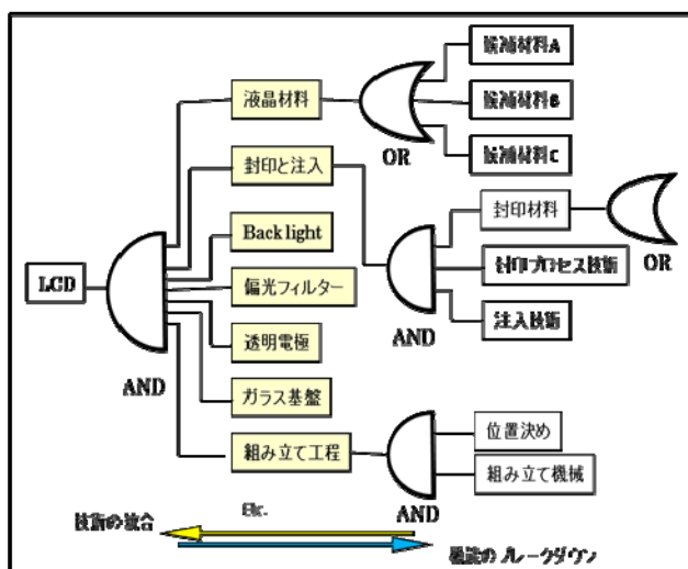
図4. 技術アーキテクチャ図LCD技術のブレイクダウン
