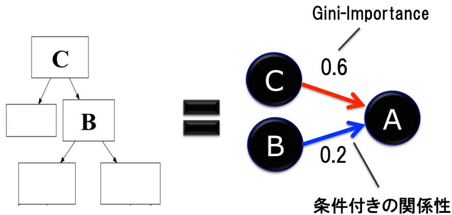
図 3.9: 決定木構造とグラフ構造
