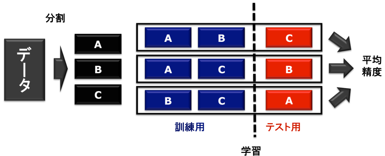
図 3.2: k-fold-CrossValidation
