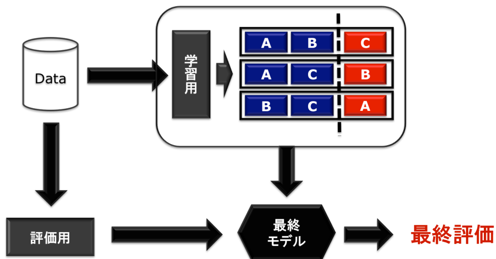
図 4.2: 学習過程
