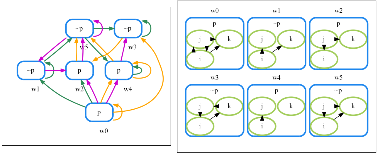
図 4.23 生成されたモデル \mathfrak{M}_2^{\text{add.ch}_j^{C_{ik}}} の画像とチャネル関係図
