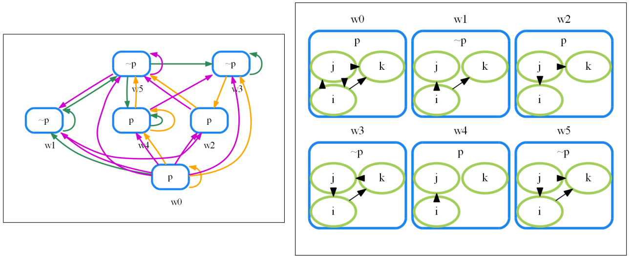
図 4.28 モデル \mathfrak{M}_5 の画像とチャネル関係図
