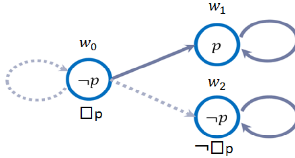
図 3.1 [\text{com } p] による信念変化
