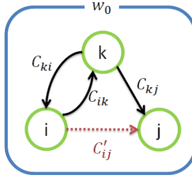
図 3.4 告知によるチャンネルの追加
