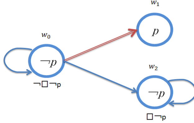
図 3.3 [\text{per } p] による信念変化
