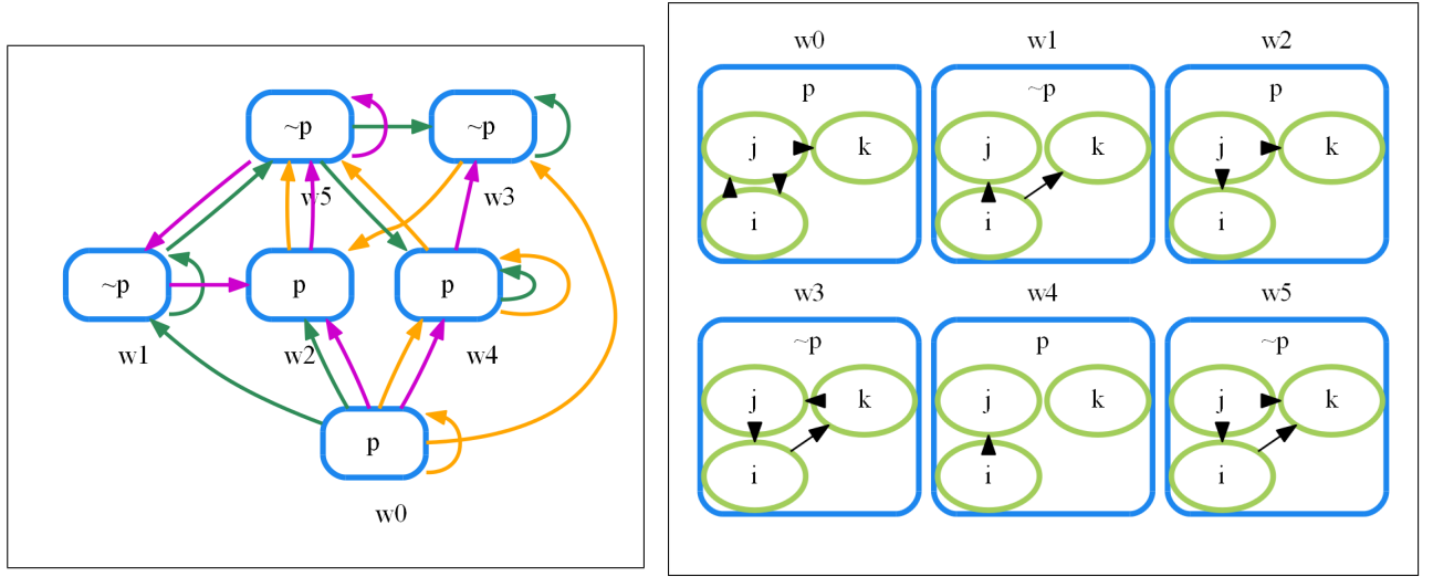
図 4.17 生成されたモデル \mathfrak{M}_2 の画像とチャネル関係図
