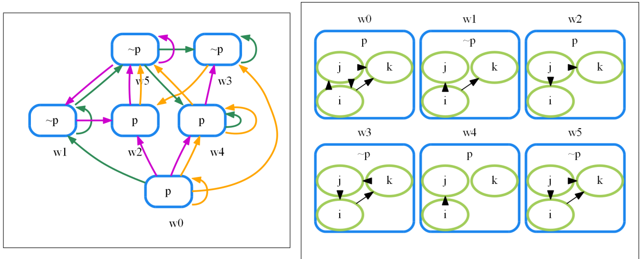
図 4.27 モデル \mathfrak{M}_4 の画像とチャネル関係図
