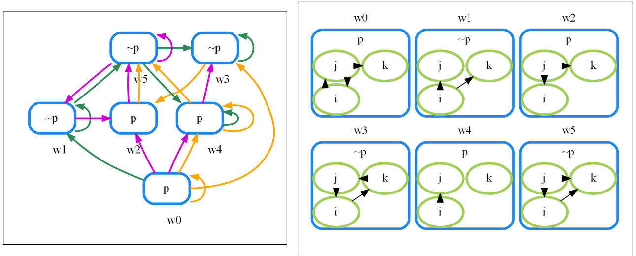
図 4.26 モデル \mathfrak{M}_3 の画像とチャネル関係図
