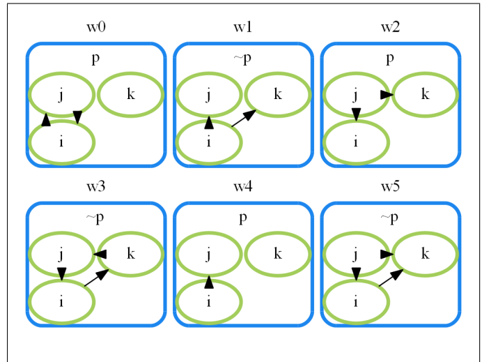
図 4.22 生成されたモデル \mathfrak{M}_2^{\text{del.ch } C_{jk}} の画像とチャネル関係図
