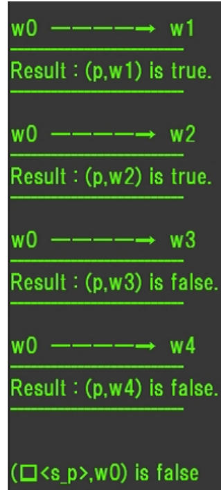
図 4.6 計算処理
