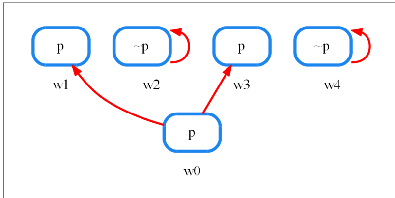
図 4.12 告知により更新されたモデル \mathfrak{M}_1^{\text{com}^{\downarrow_s} p}
