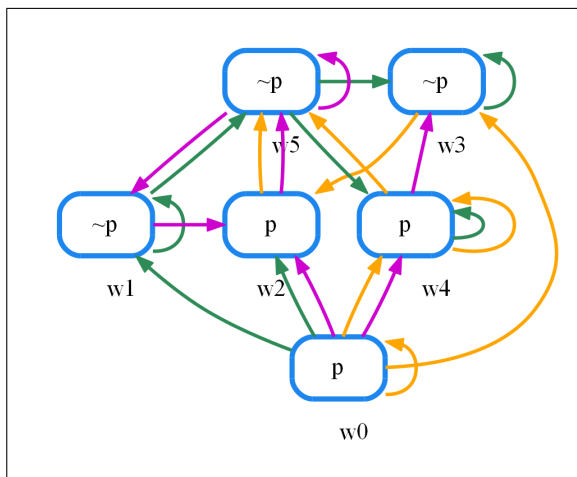
図 4.22 生成されたモデル \mathfrak{M}_2^{\text{del.ch } C_{jk}} の画像とチャネル関係図
