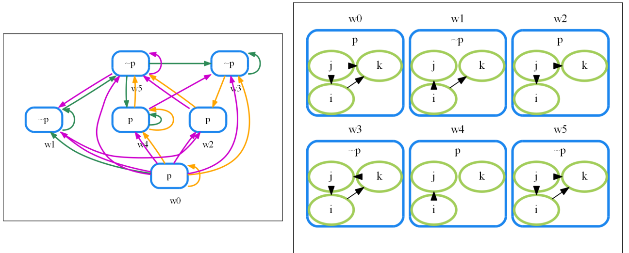
図 4.29 モデル \mathfrak{M}_6 の画像とチャネル関係図
