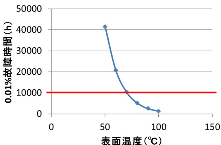
図 2.2: 動作温度と寿命
