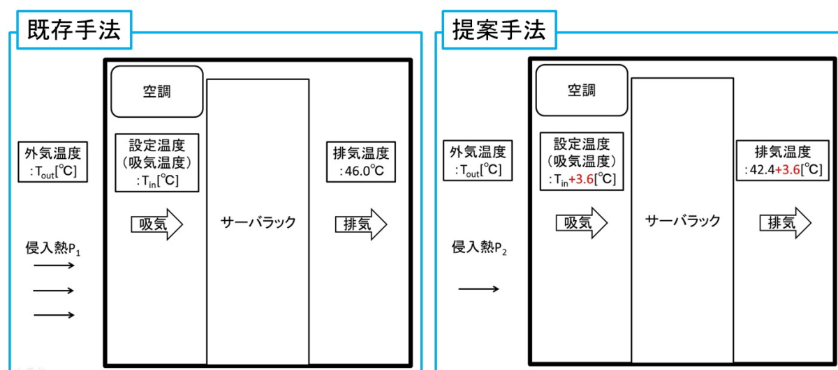
図 2.3: 侵入熱にかかる空調電力削減手法
