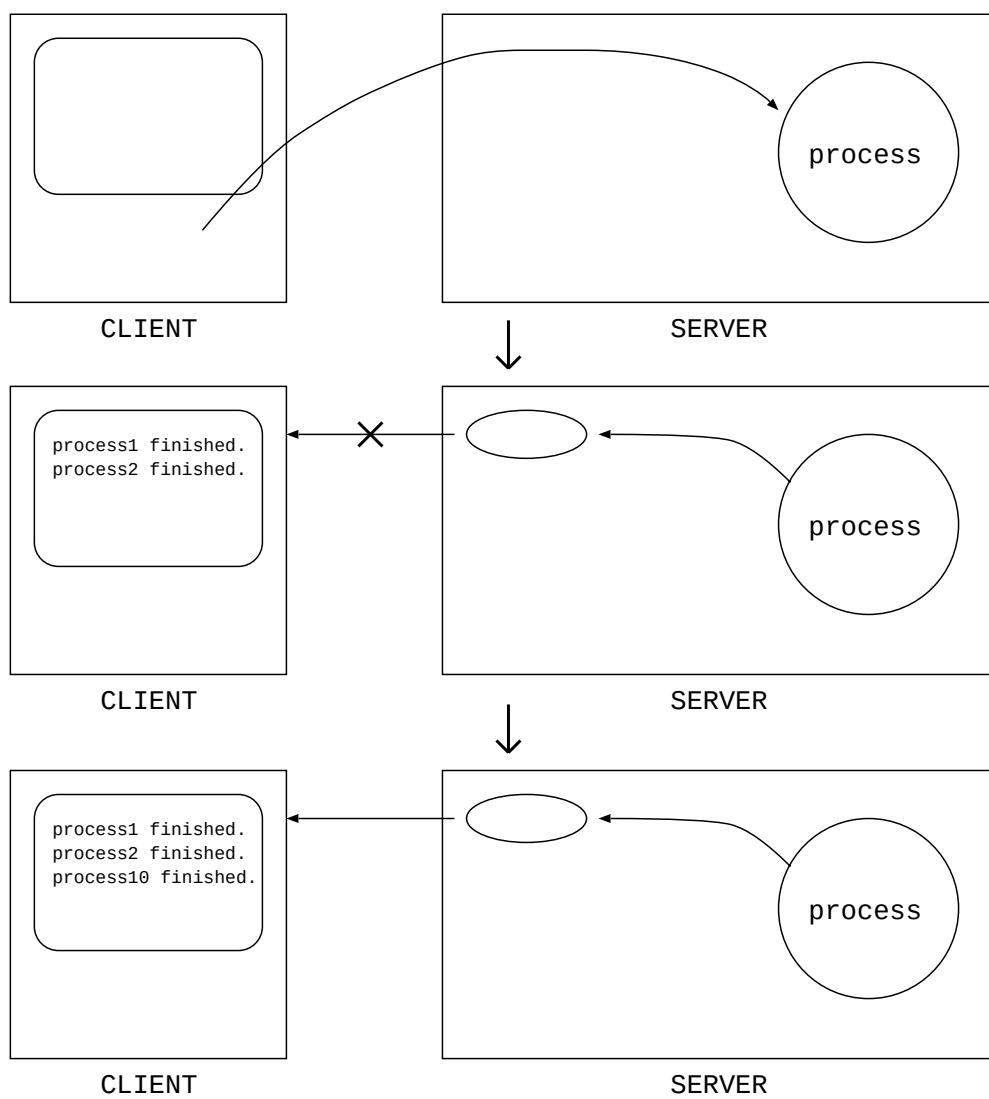
図 5.1: 作業状況を返す場合の切断時操作
