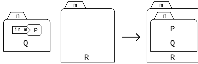
図 4.2: 侵入リダクション
