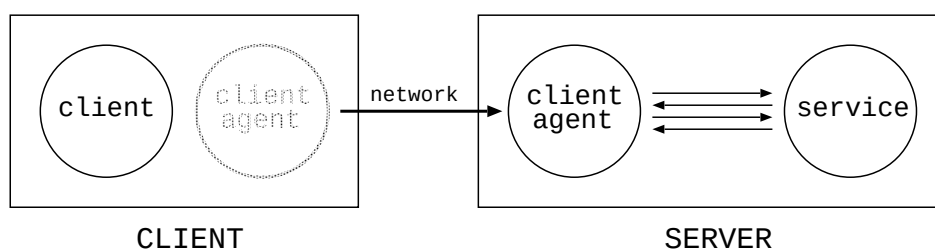
図 2.1: 移動エージェント
