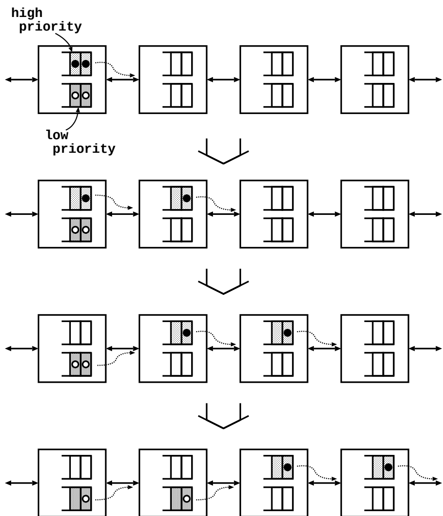
図 3.4: 占有法による空白の抑制
