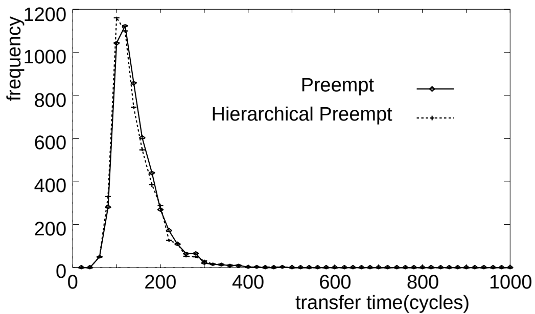
図 6.10: TESH におけるランダム通信の転送時間分布（チャンネル数 8、パケット生成率 1.0 \times 10^{-3} ）
