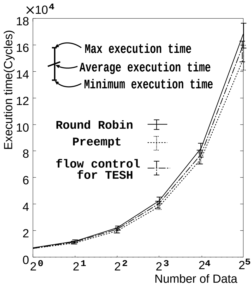
図 6.13: FFT の実行時間の比較
