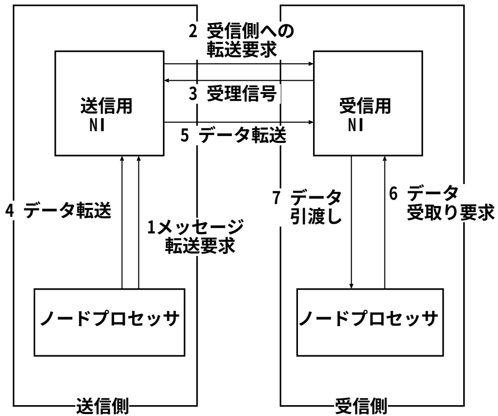
図 4.2: 通信の手順
