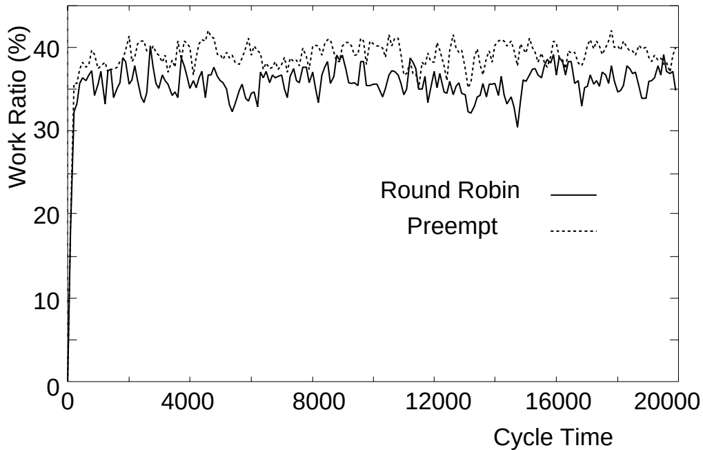
図 5.10: リンクの稼働率
