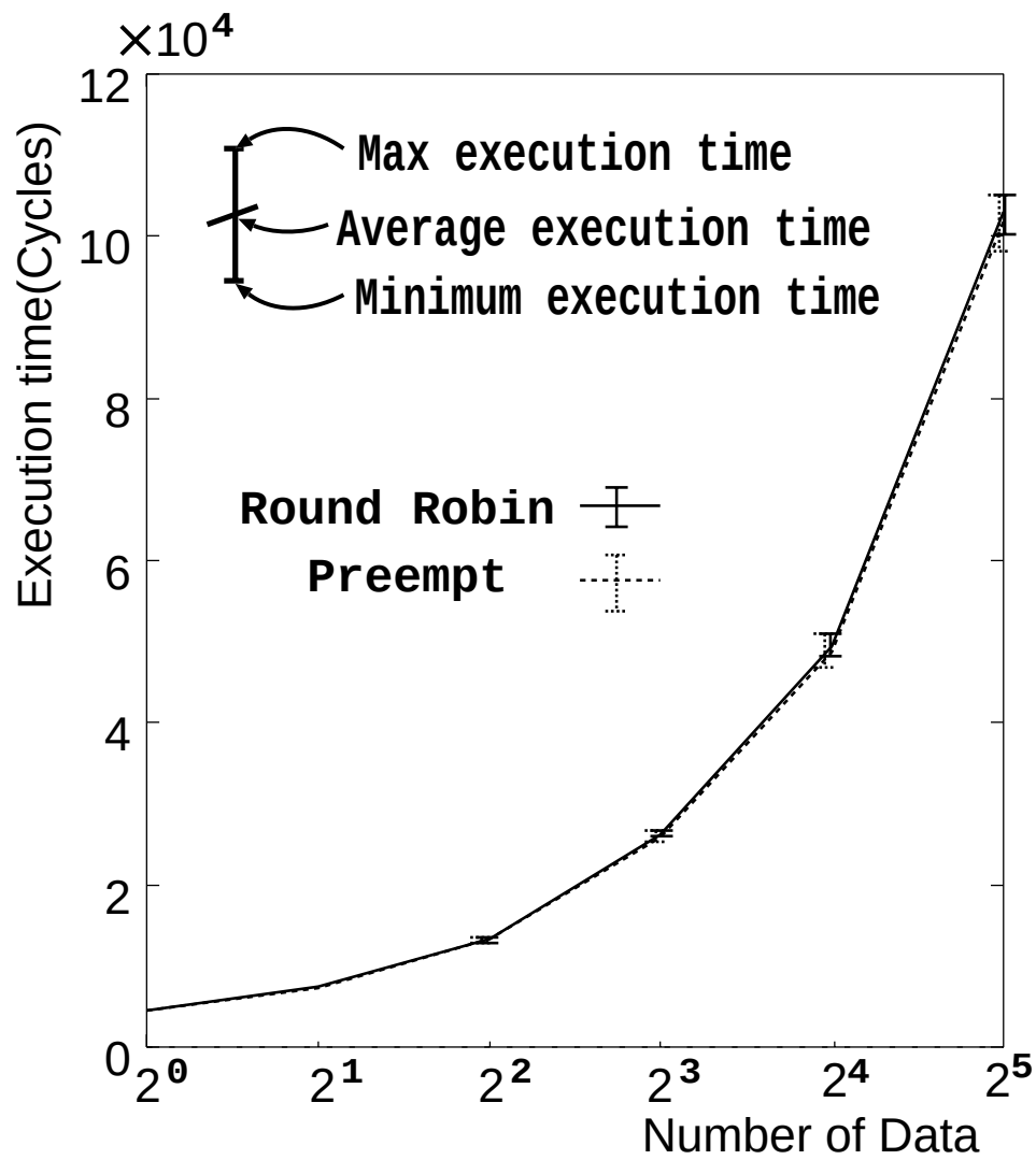
図 5.17: FFT の実行時間
