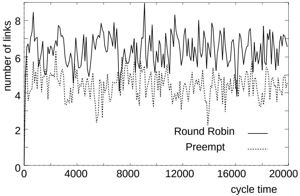
図 6.7: フリット間に空白があるために転送が行えないリンクの数
