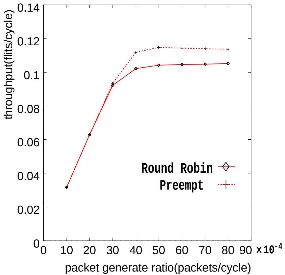
図 5.6: ランダム通信の平均スループット (パケット長 32)
