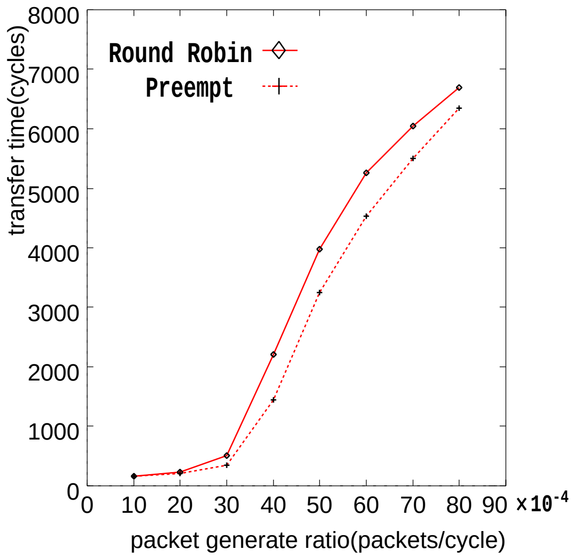
図 5.5: ランダム通信の平均転送時間 (パケット長 32)
