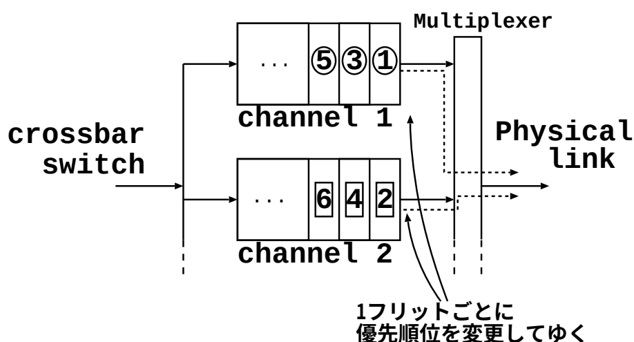
図 2.8: ラウンドロビンのフロー制御
