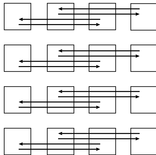
図 5.15: FFT の通信パターン
