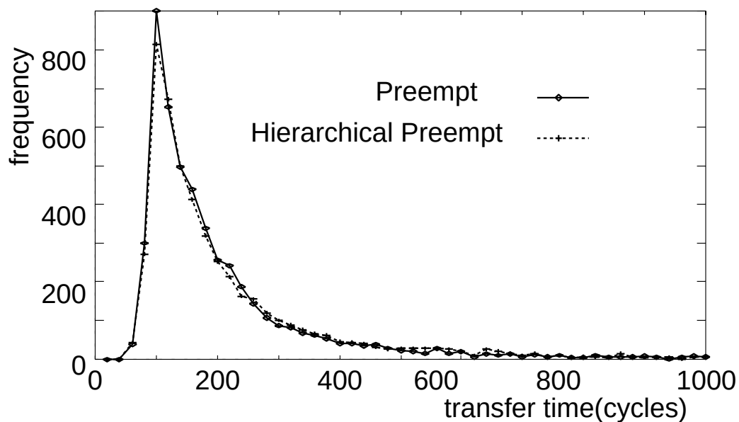
図 6.9: TESH におけるランダム通信の転送時間分布（チャネル数 4）
