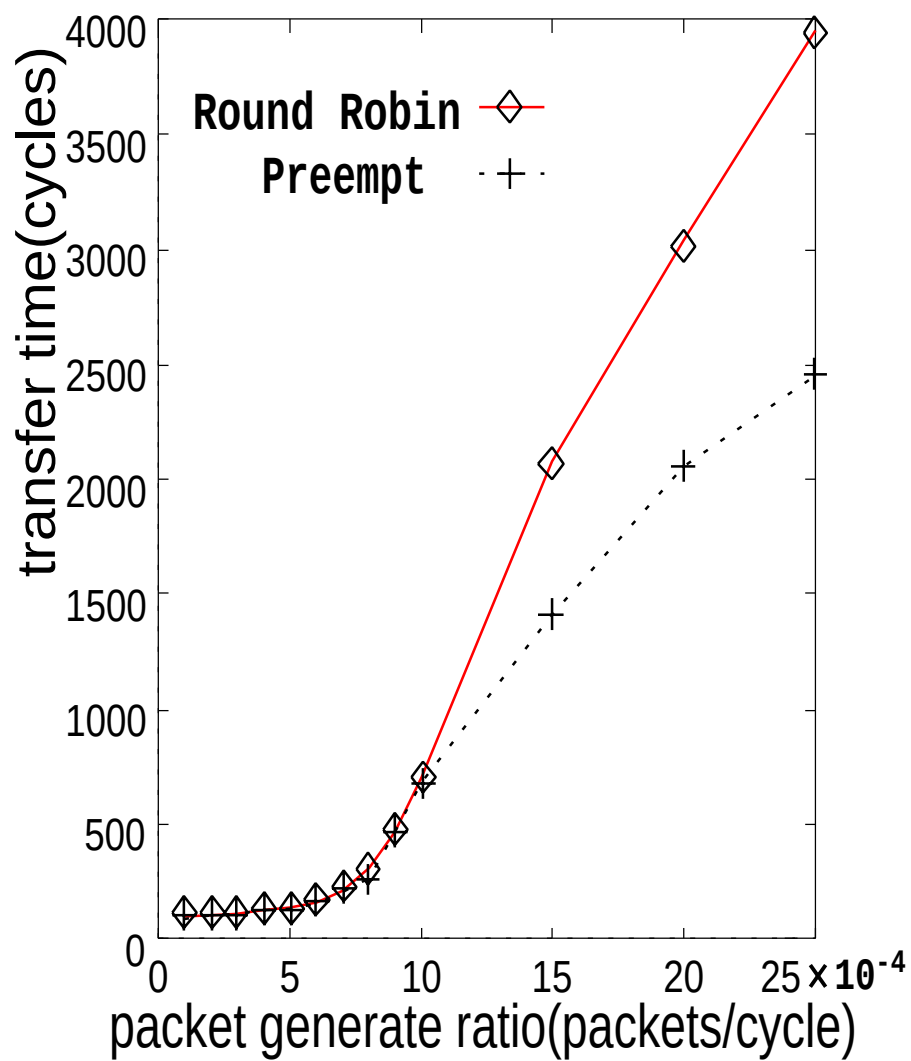
図 5.9: 転送先が集中した通信の平均転送時間
