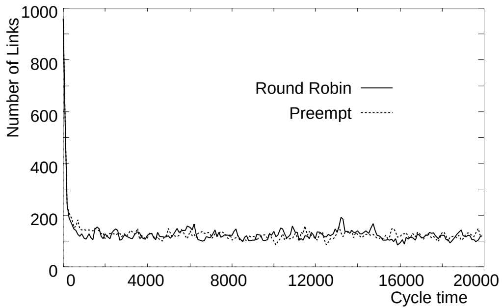
図 5.12: パケットが存在しないために転送を行なわないリンクの数
