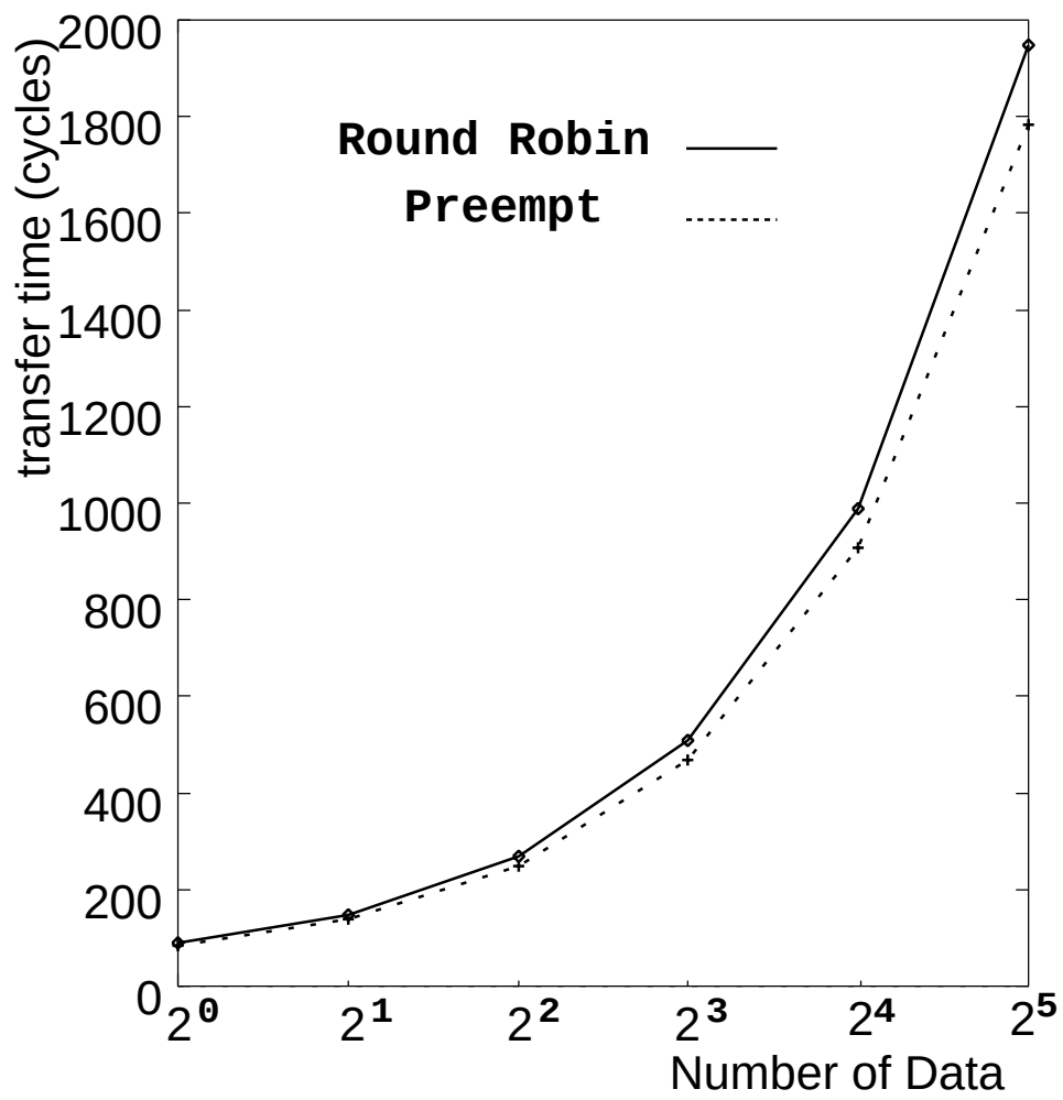
図 5.16: FFT における各手法の平均通信時間
