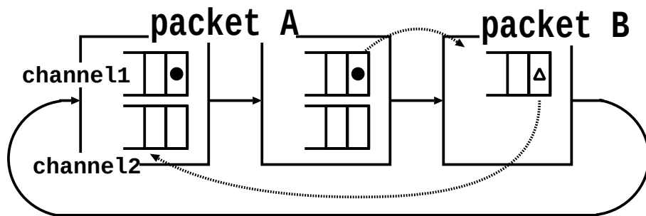
図 2.6: 仮想チャネルによるデッドロックの回避
