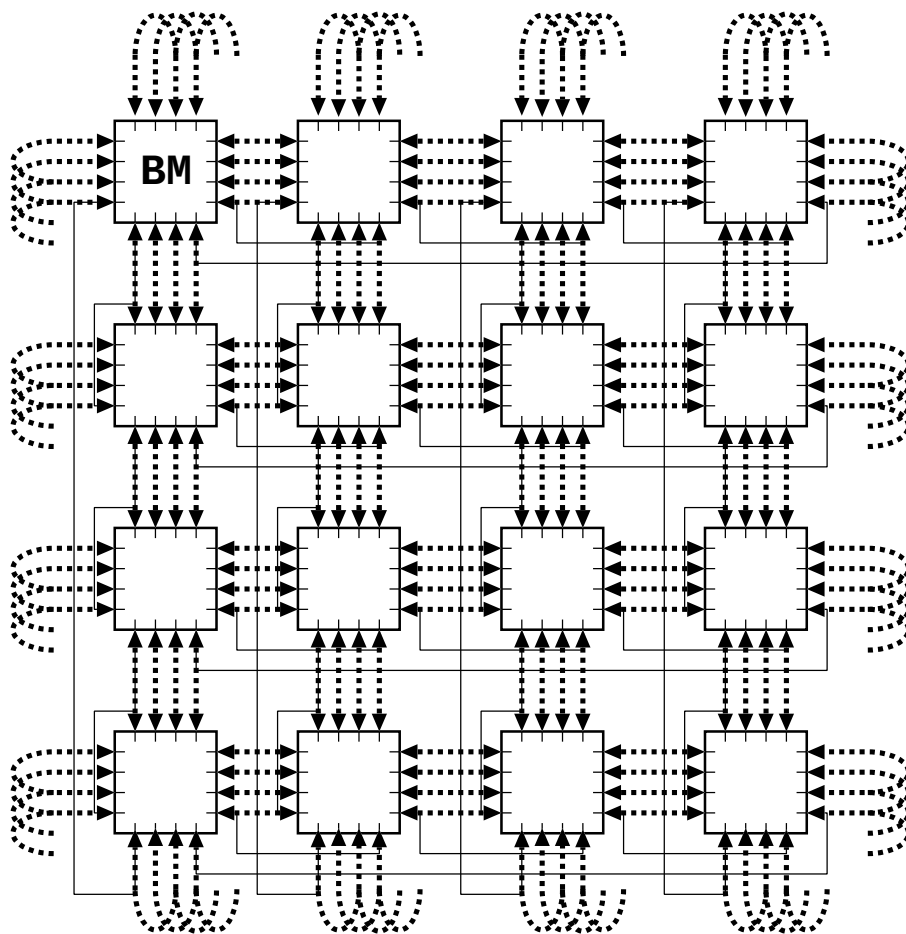
図 6.14: 四方向通信の BM 間通信
