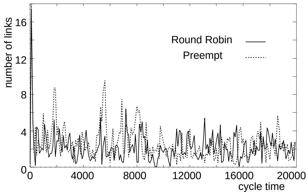
図 6.6: パケットが存在しないために転送を行わないリンクの数
