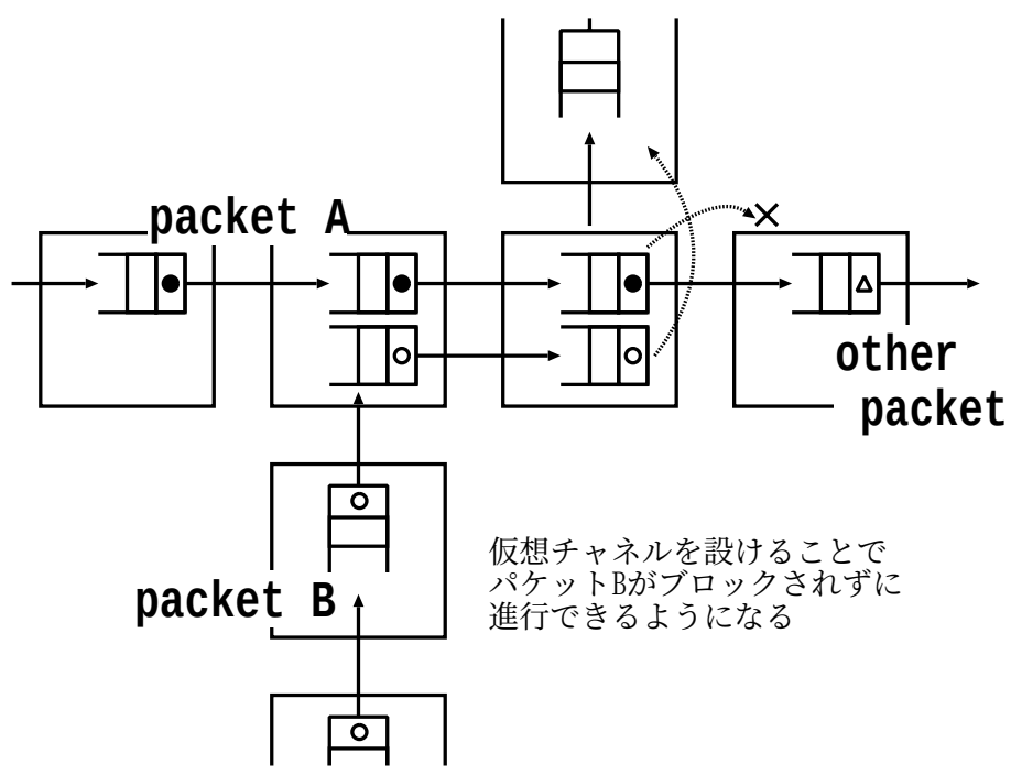
図 2.4: 仮想チャネルの利用によるブロックの回避
