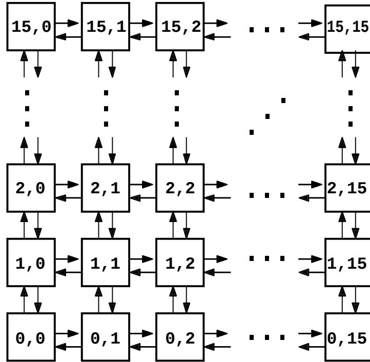
図 5.2: 実験に用いる二次元メッシュ
