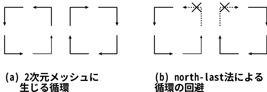
図 5.18: Turn モデル
