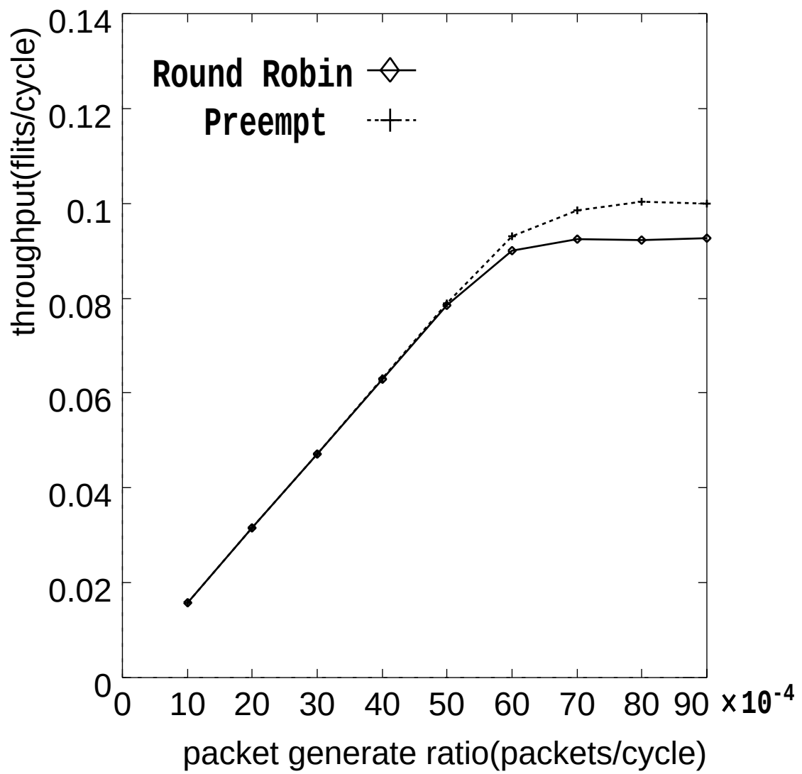
図 5.4: ランダム通信の平均スループット (パケット長 16)
