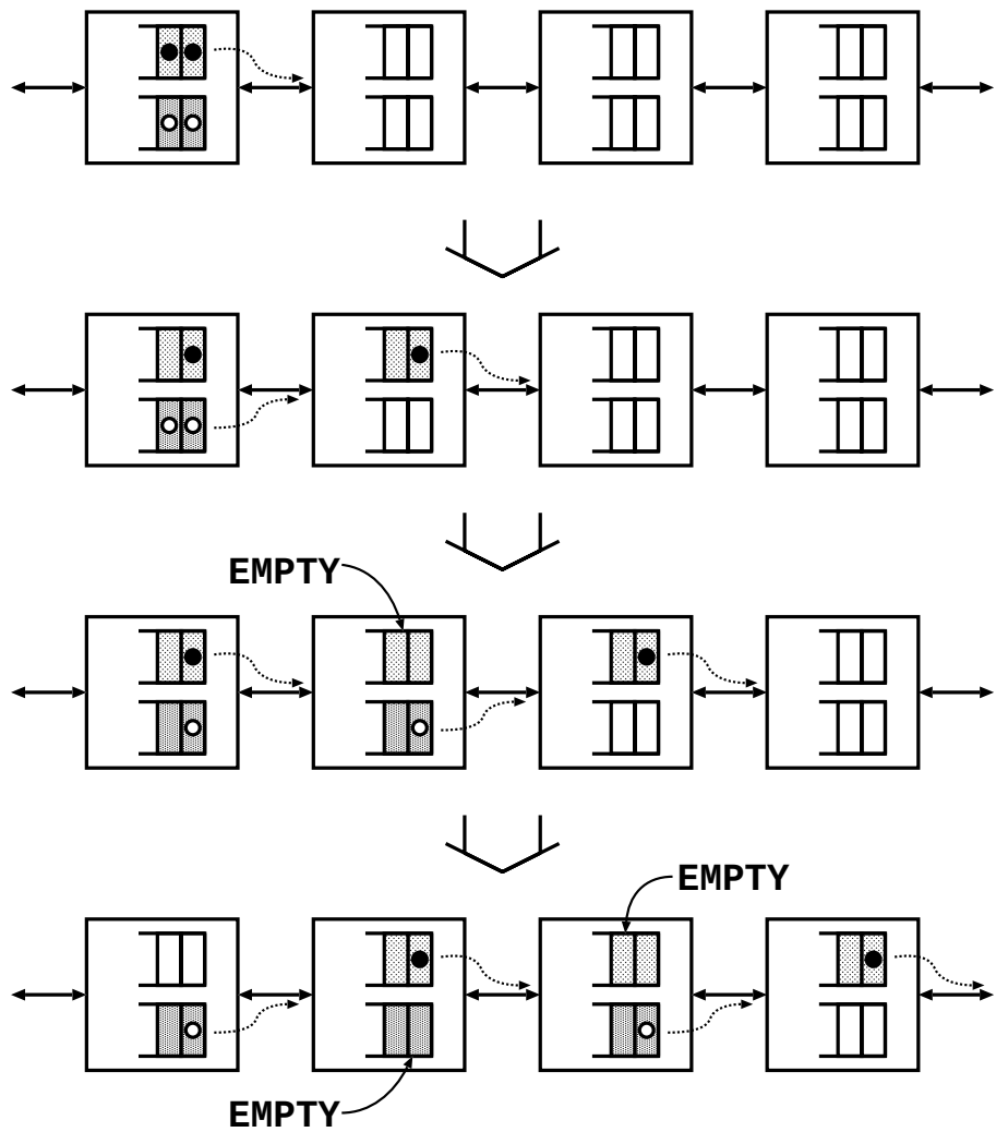
図 3.2: ラウンドロビンにより発生する空白
