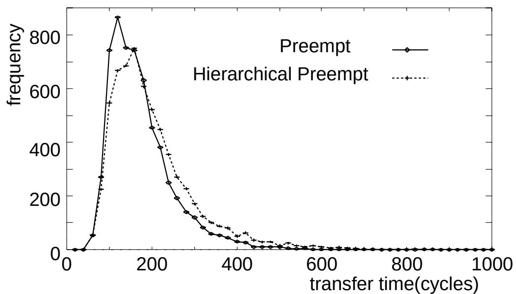
図 6.11: TESH におけるランダム通信の転送時間分布（チャンネル数 8、パケット生成率 1.2 \times 10^{-3} ）
