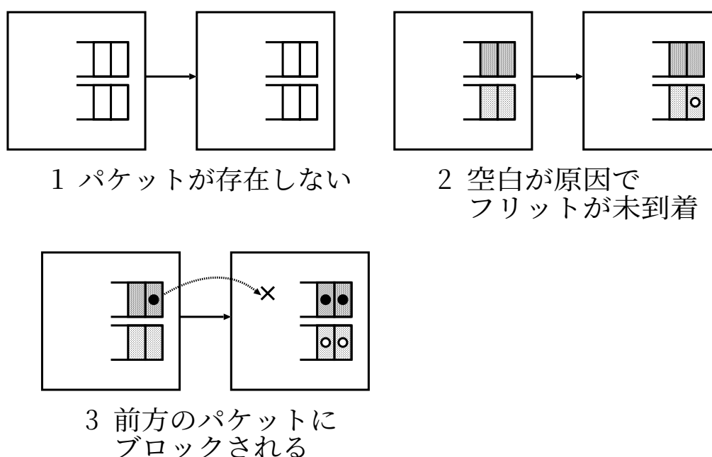
図 5.11: フリットが転送されない原因
