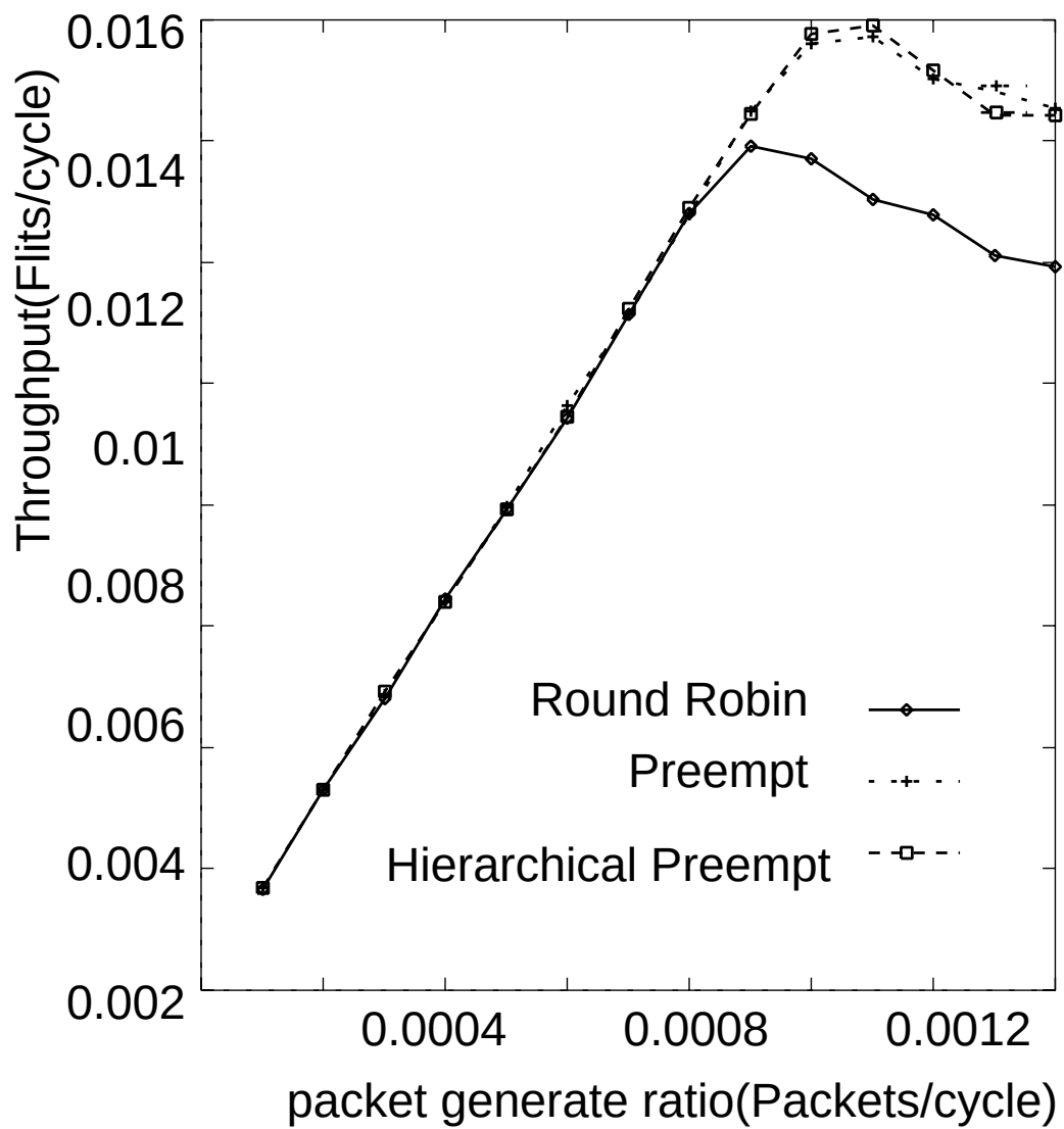
図 6.4: TESH におけるランダム通信の平均スループット
