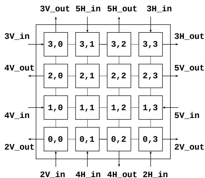
図 6.1: 基本モジュールの構成
