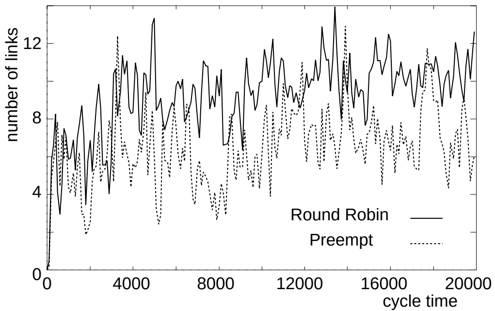
図 6.8: 前方のパケットにブロックされるために転送が行えないリンクの数
