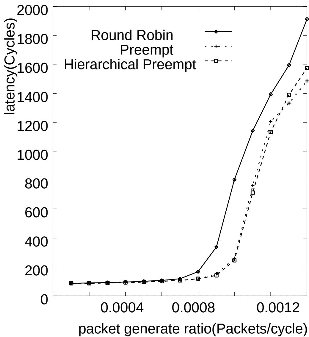
図 6.3: TESH におけるランダム通信の平均転送時間
