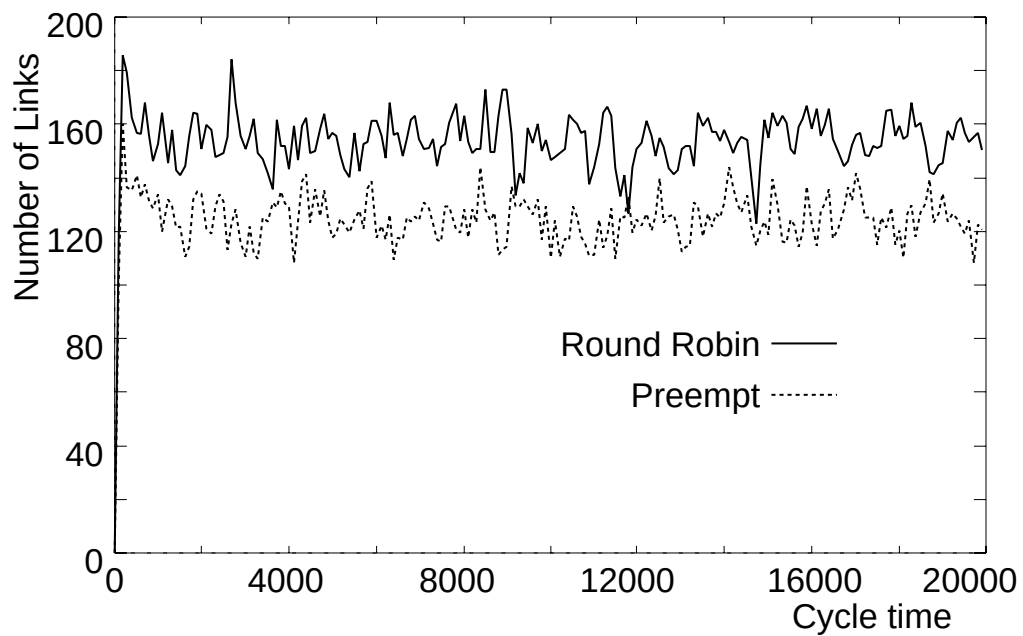
図 5.13: フリット間に空白があるために転送が行えないリンクの数
