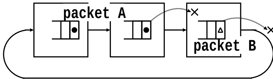
図 2.5: デッドロックの例
