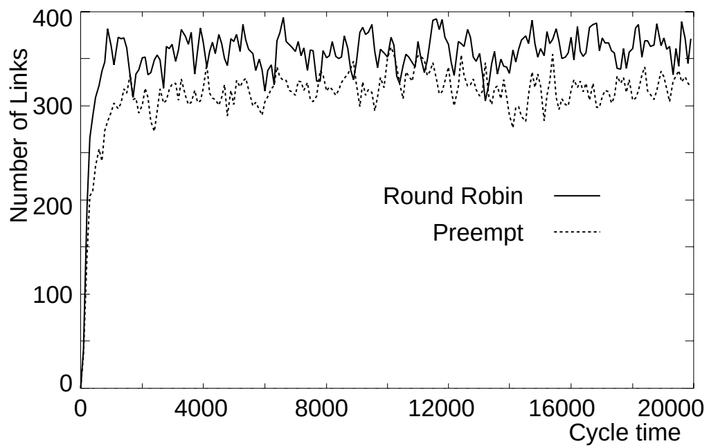
図 5.14: 前方のパケットにブロックされるために転送が行えないリンクの数
