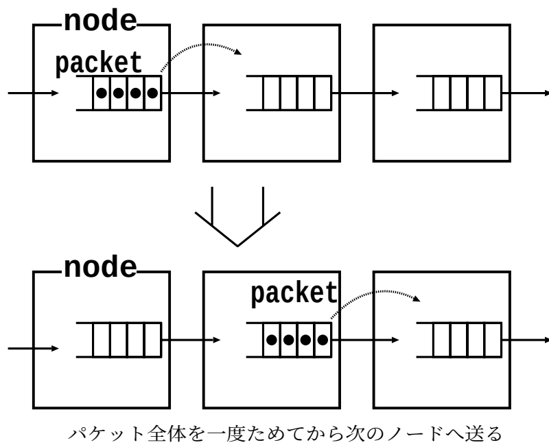
図 2.1: ストアアンドフォワード
