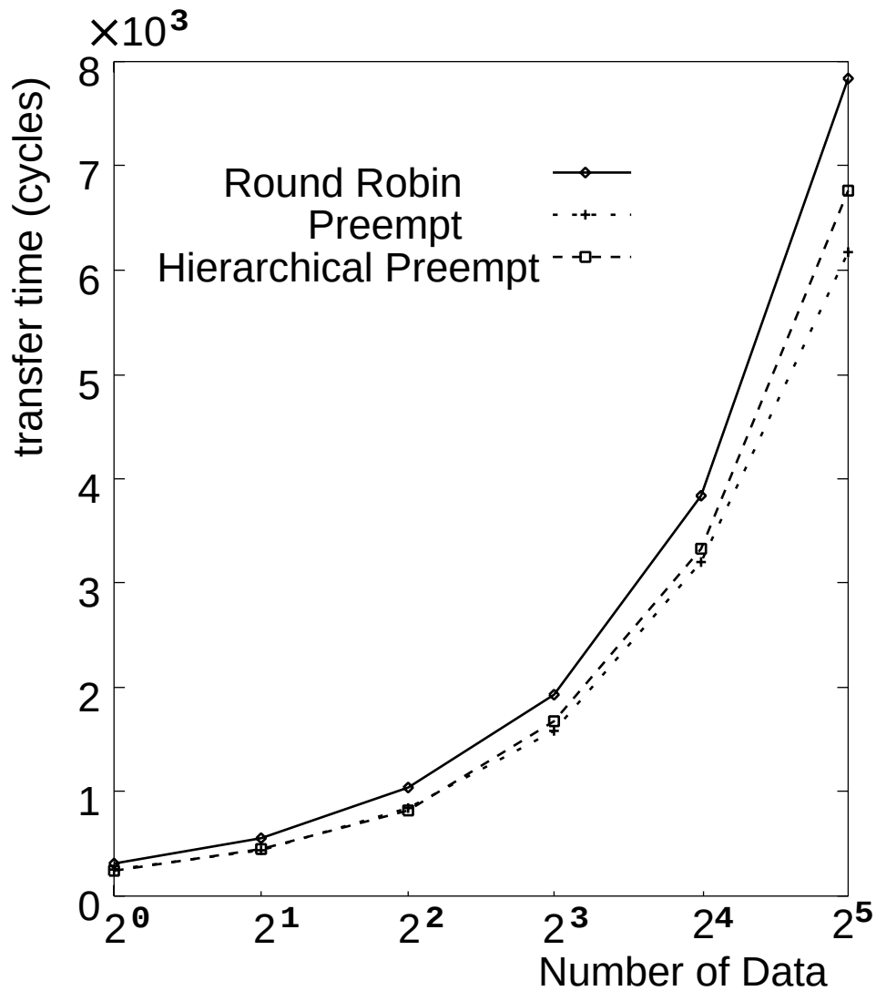
図 6.12: FFT における各手法の平均通信時間
