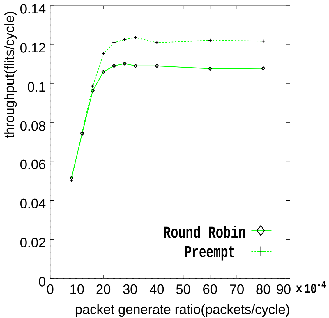
図 5.8: ランダム通信の平均スループット (パケット長 64)
