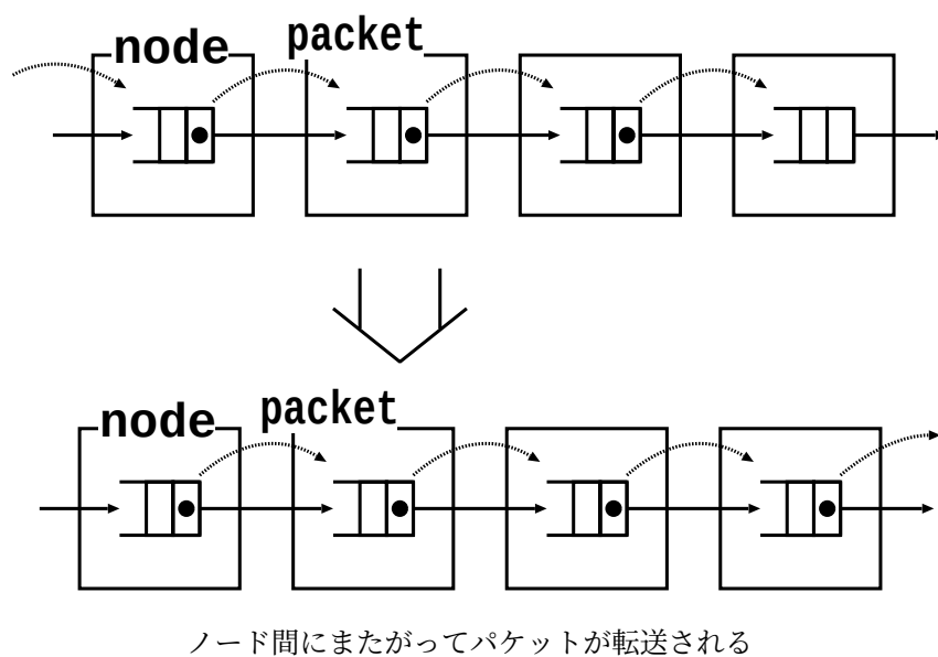
図 2.2: ワームホールルーティング
