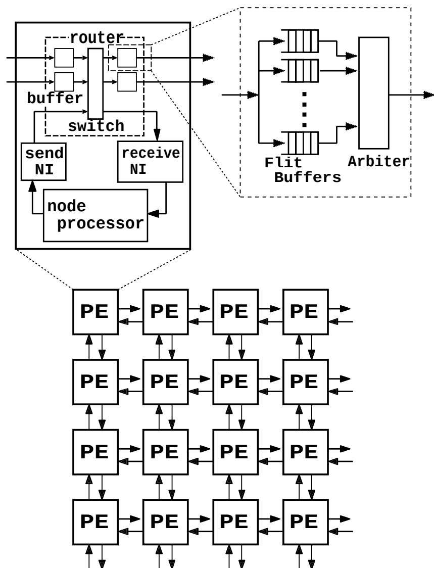
図 4.1: システム構成
