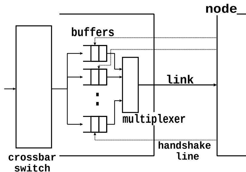
図 2.7: 仮想チャネルの物理的構成
