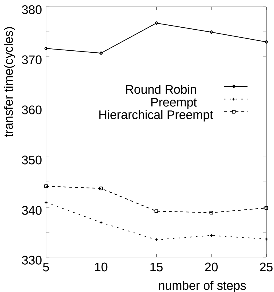
図 6.15: 四方向通信の平均通信時間
