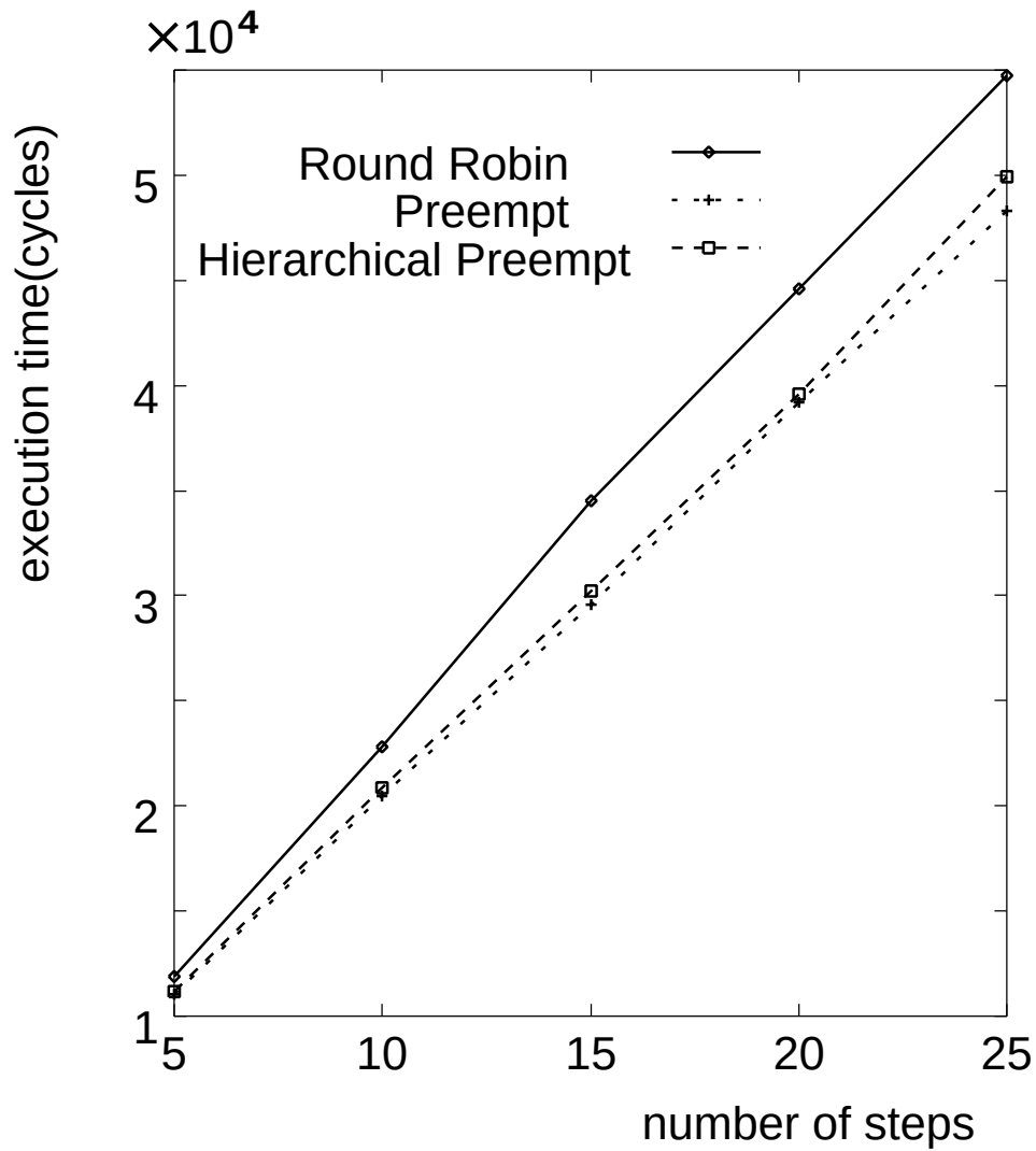
図 6.16: 四方向通信の実行時間
