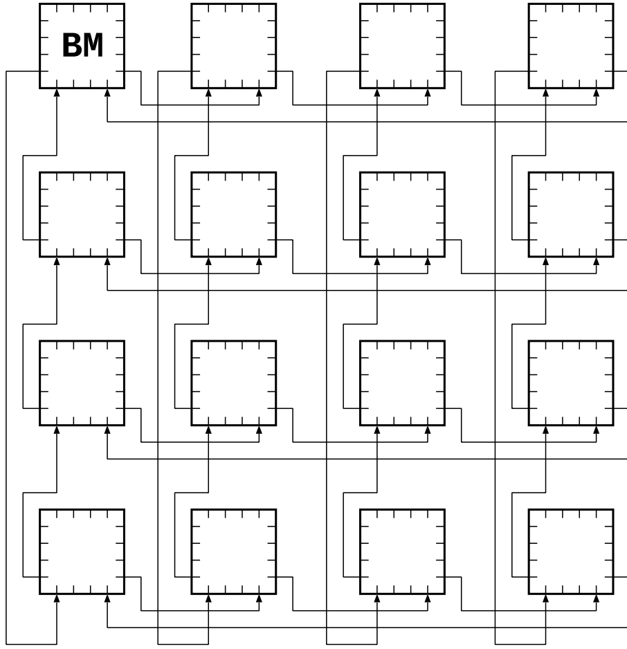
図 6.2: TESH(2,2,0) の構成
