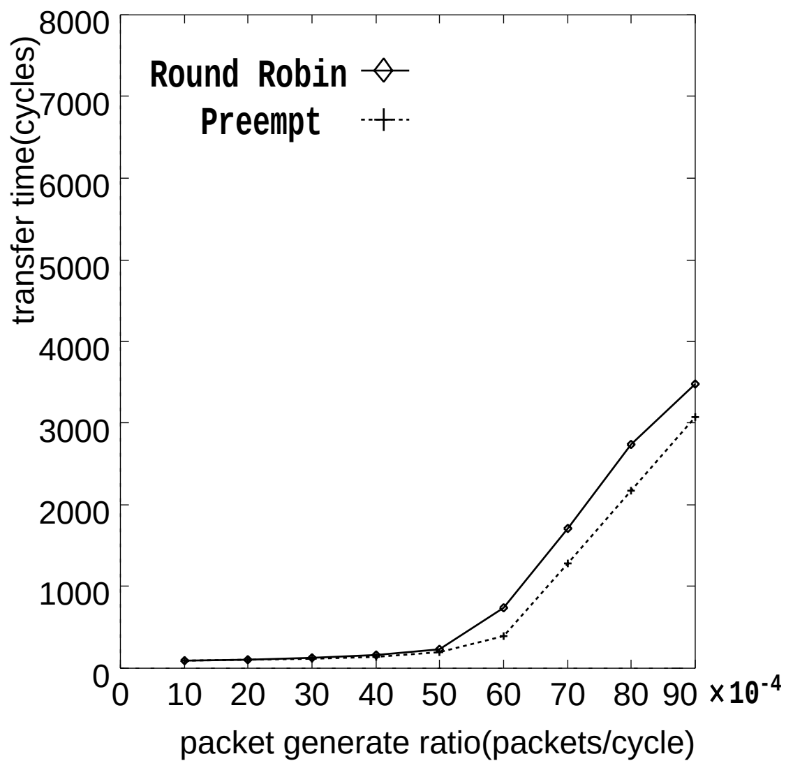
図 5.3: ランダム通信の平均転送時間 (パケット長 16)
