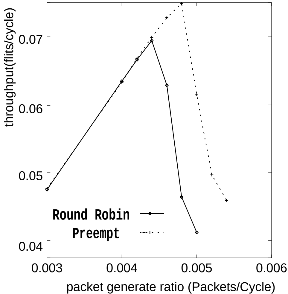
図 5.20: north last 法によるランダム通信の平均スループット
