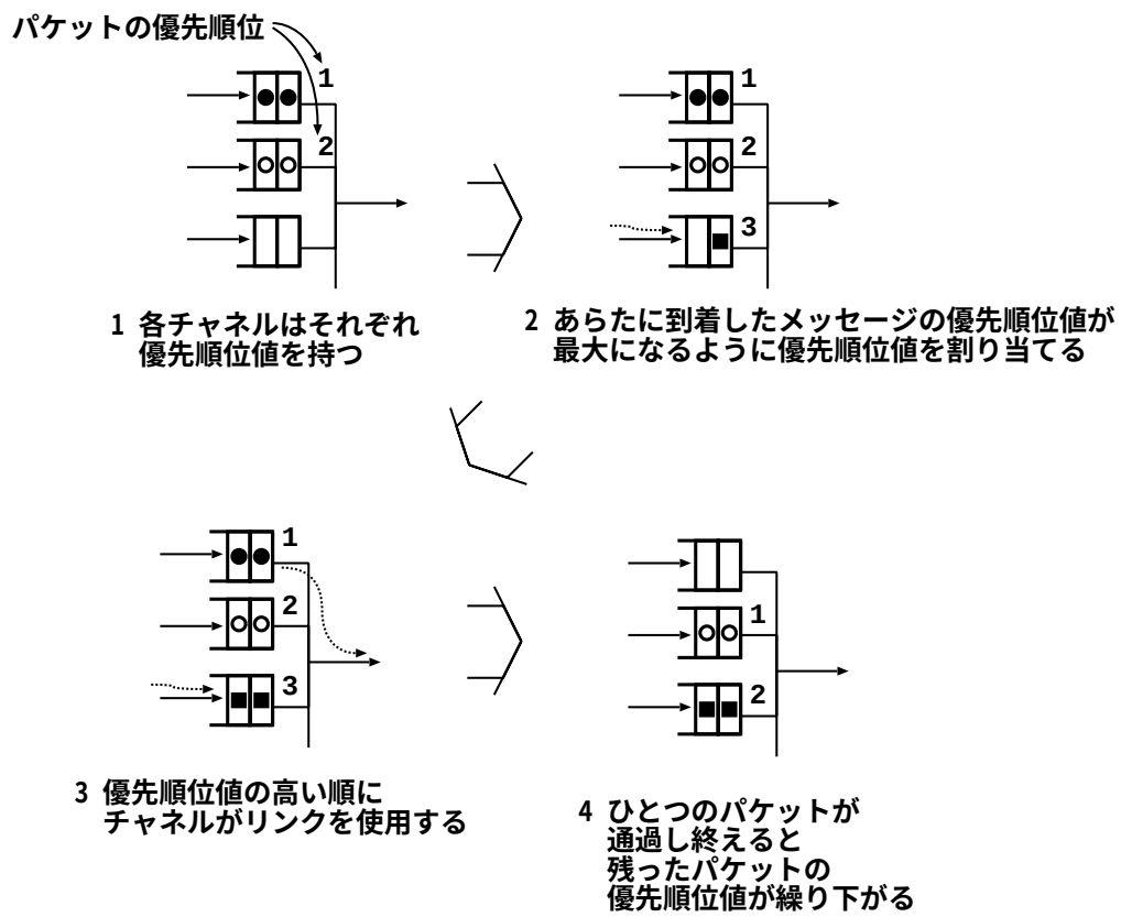
図 3.3: 占有法のフロー制御
