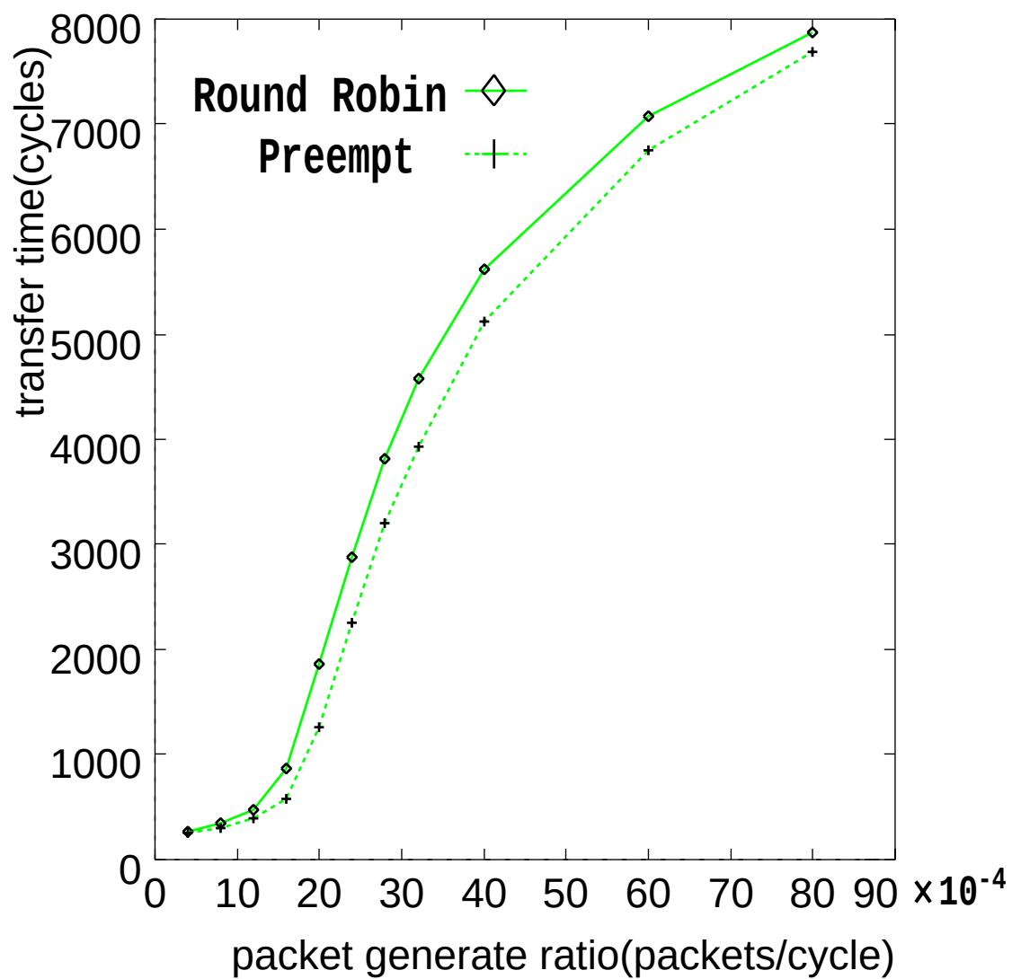
図 5.7: ランダム通信の平均転送時間 (パケット長 64)
