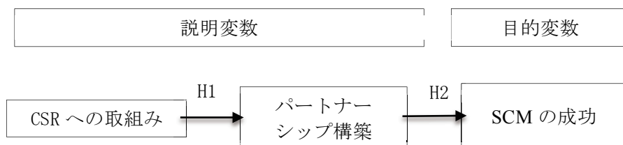
図 1 仮説モデル
