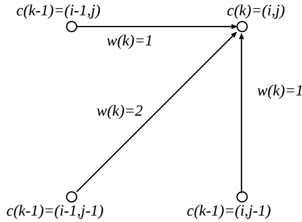
図 4.2: DP マッチングの傾斜制限
