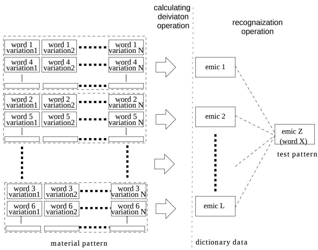
図 4.6: 単語から音韻抽出認識のための辞書作成
