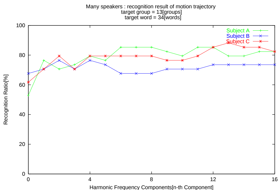
図 5.12: 34 単語に対する複数話者の運動軌跡認識結果
