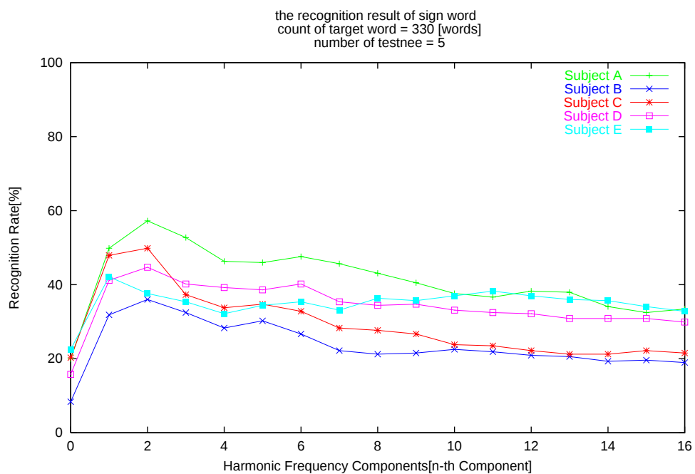
図 5.9: 5 人を対象にした複数話者認識の結果
