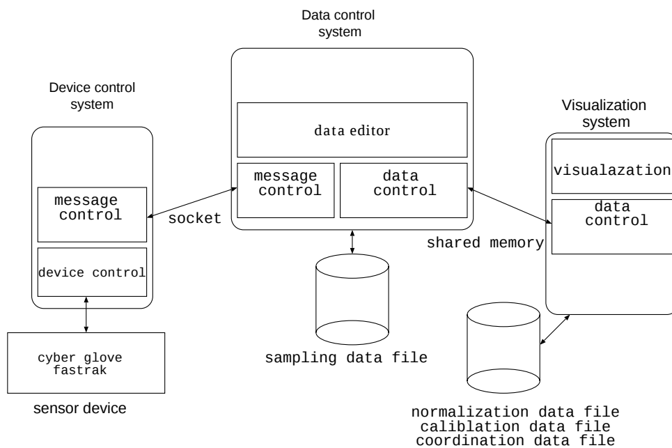
図 3.2: システムモデル
