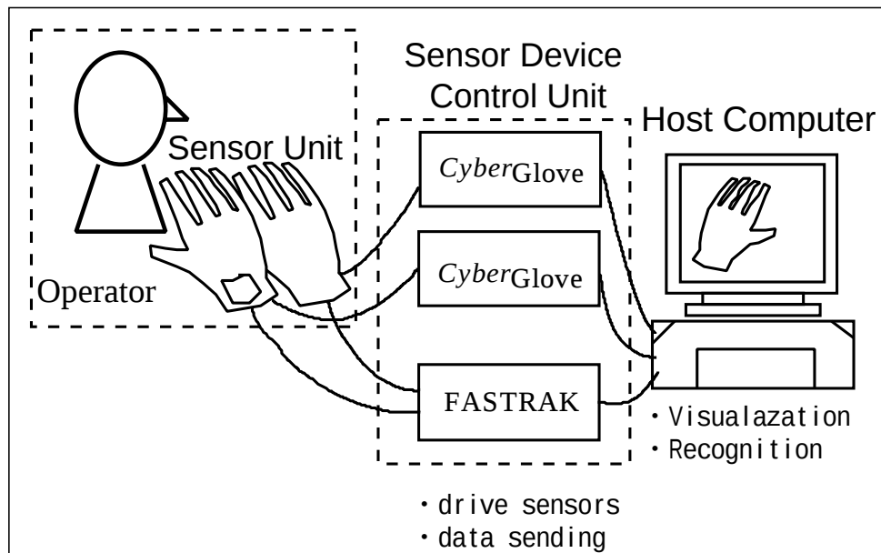
図 3.1: 単語データ入力システム
