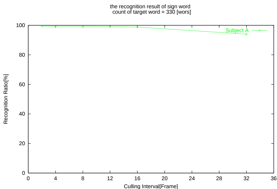
図 5.2: DP マッチングを用いた特定話者認識結果
