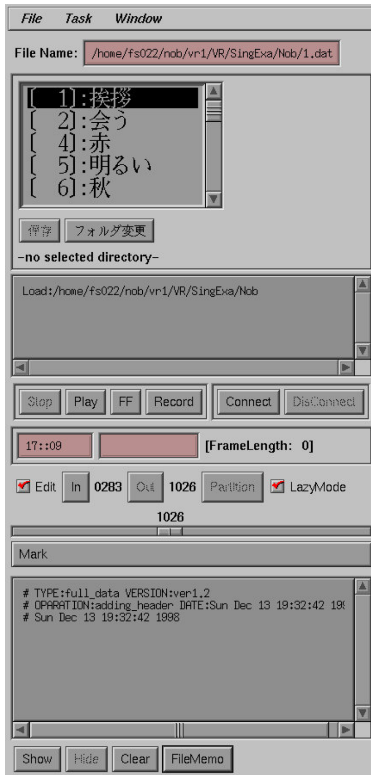
図 3.15: 手話単語採取インターフェイス
