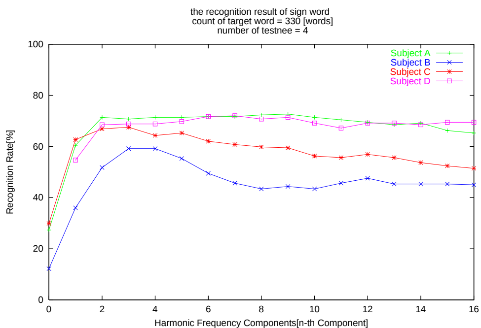
図 5.8: 4 人を対象にした複数話者認識の結果
