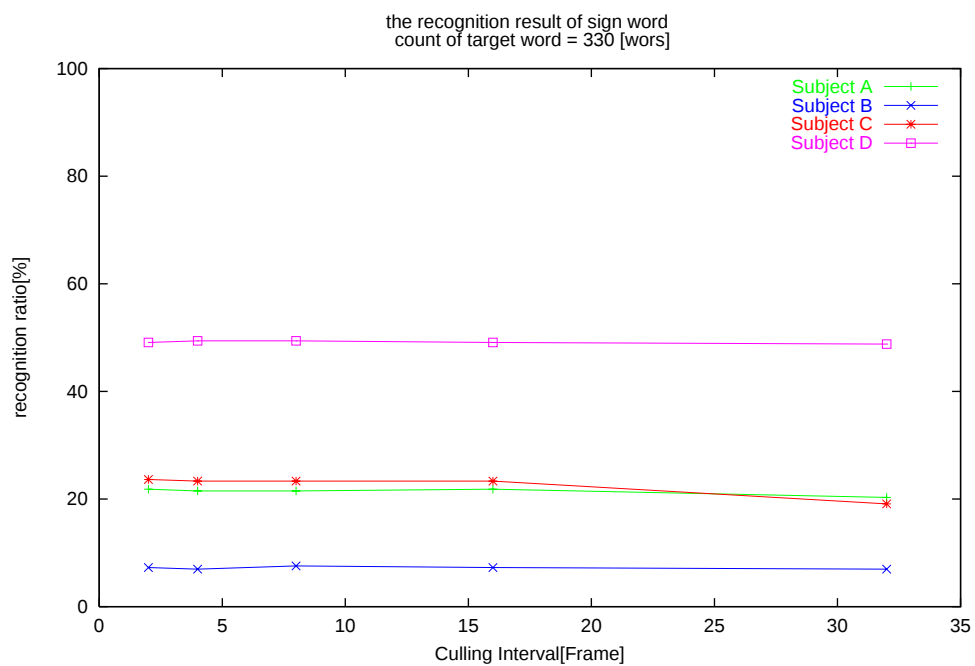
図 5.3: DP マッチングを用いた複数話者認識結果
