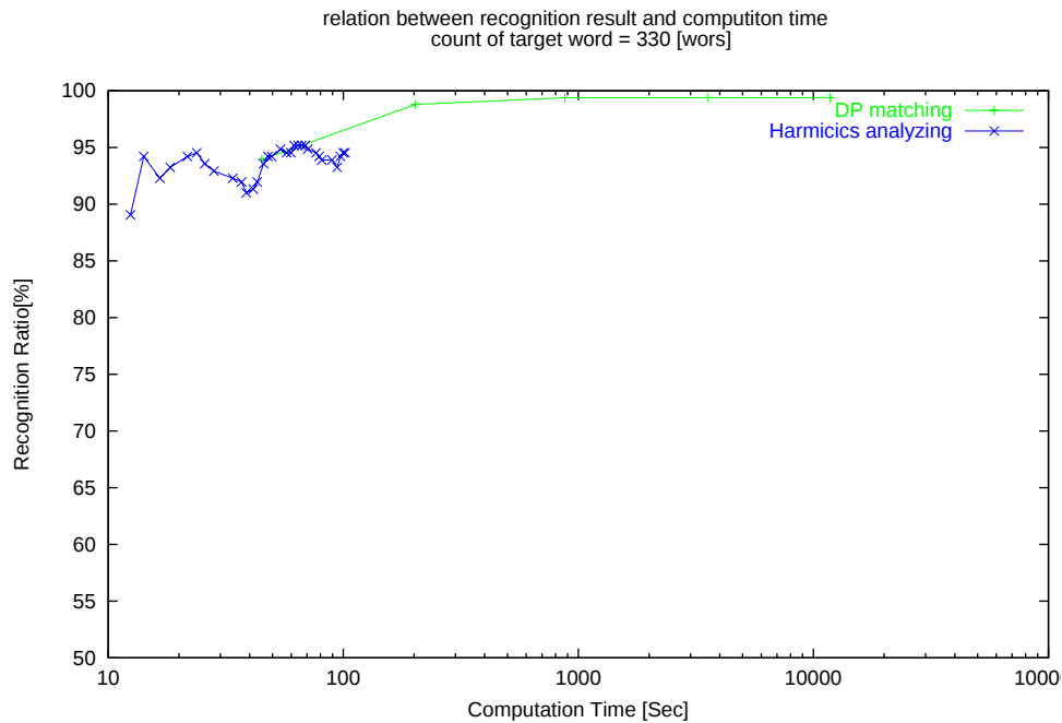
図 5.13: 認識時間の比較
