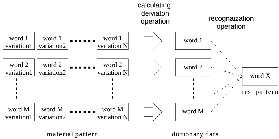
図 4.4: 単語対単語認識時の辞書作成
