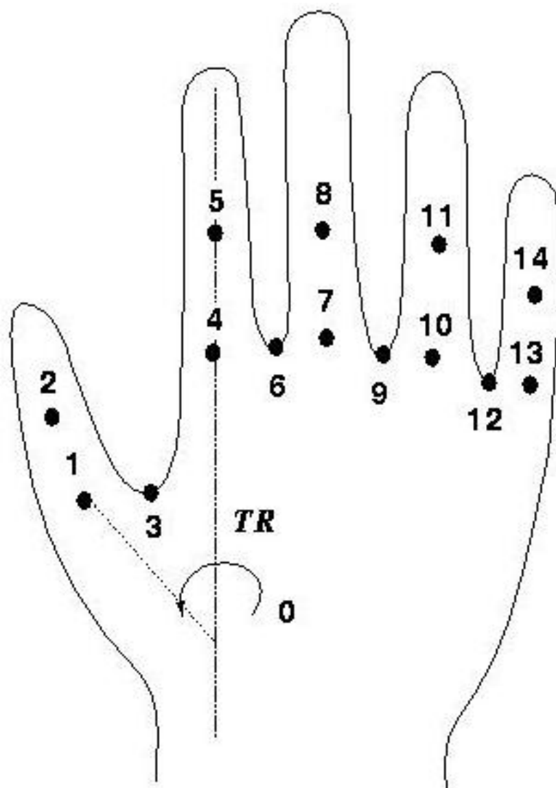
図 3.4: 手形状入力装置の関節角測定点
