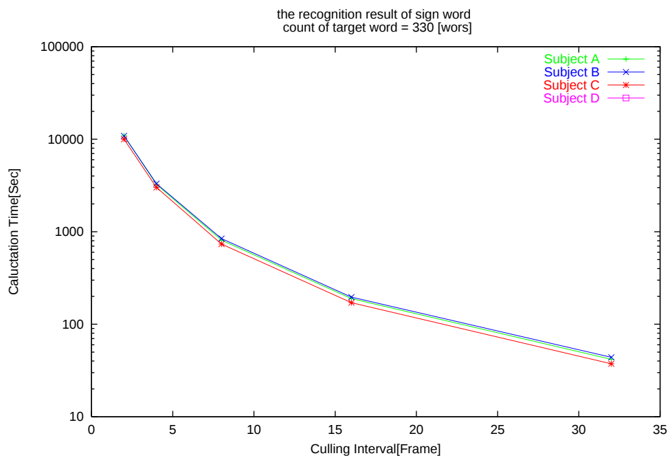
図 5.4: DP マッチングの間引き間隔による演算時間
