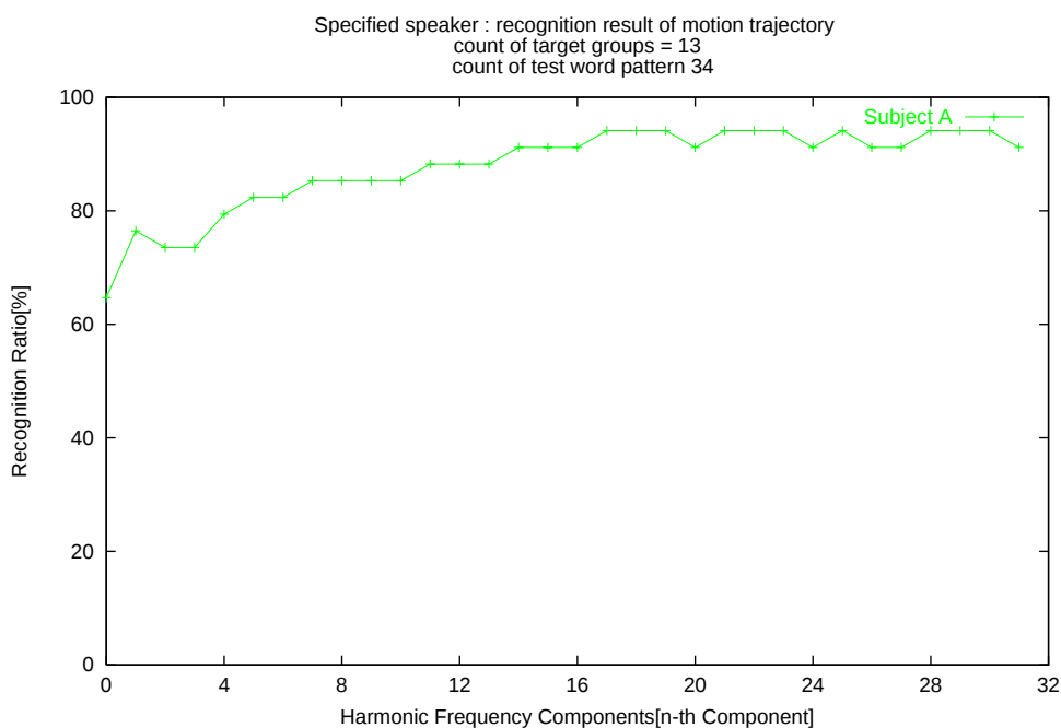
図 5.11: 34 単語に対する特定話者の運動軌跡認識結果
