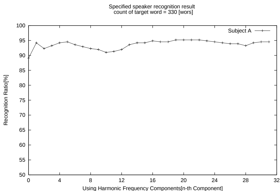
図 5.6: 周波数分析による特定話者認識結果
