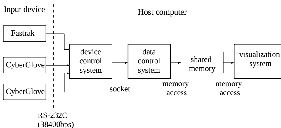
図 3.6: 手話単語データの流れ
