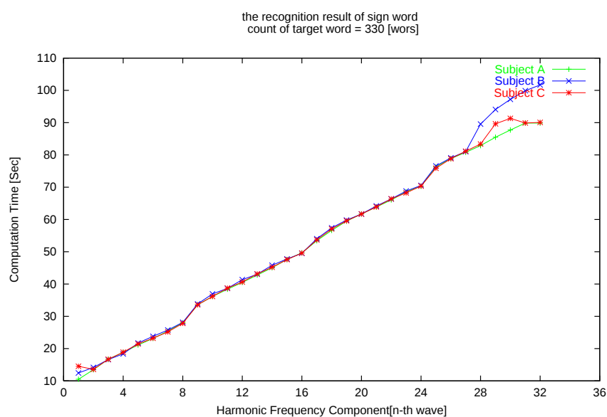
図 5.10: 有効高調波階数と認識時間の関係
