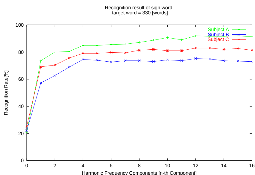
図 5.7: 3 名を対象とした有効高調波階数と認識率の関係
