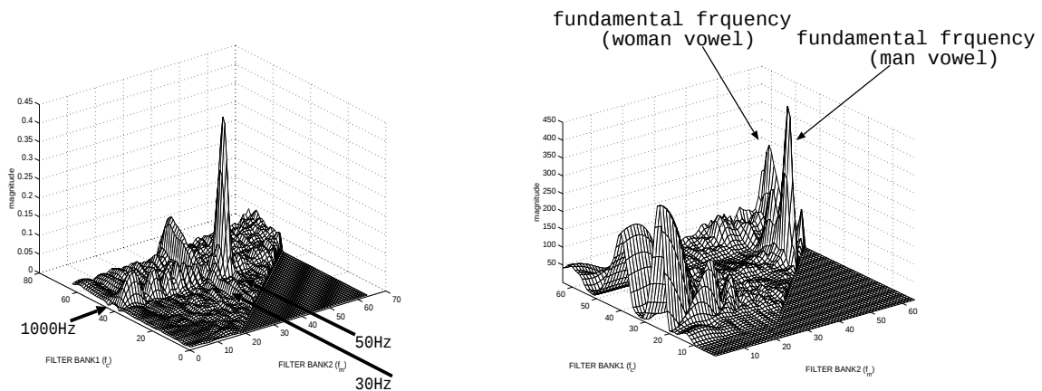
図 4: 変調－搬送周波数マップの検出結果 ( 時間平均 )
