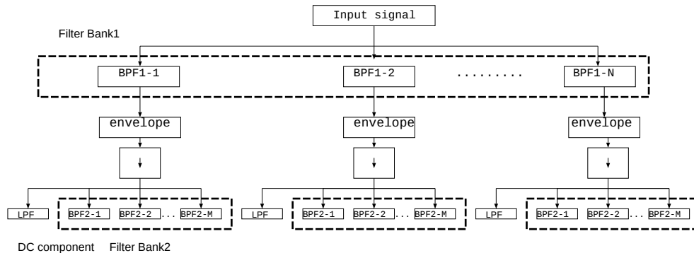
図 2: 変調－搬送周波数マップ検出モデル
