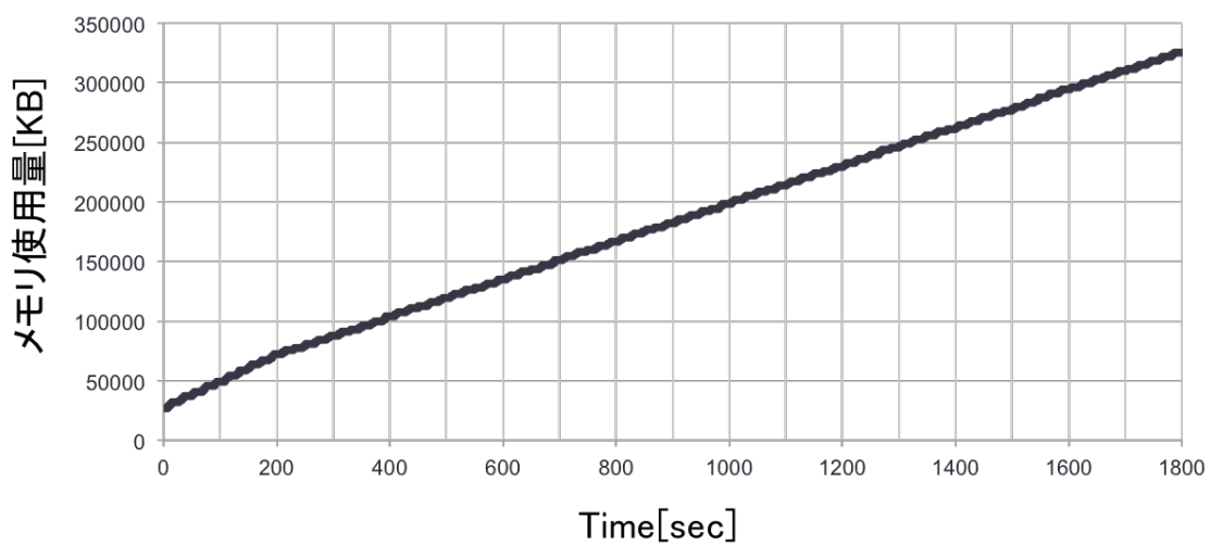
図 5.8: 軽量クライアントモジュールを 10000 台動作させた際のメモリ使用量
