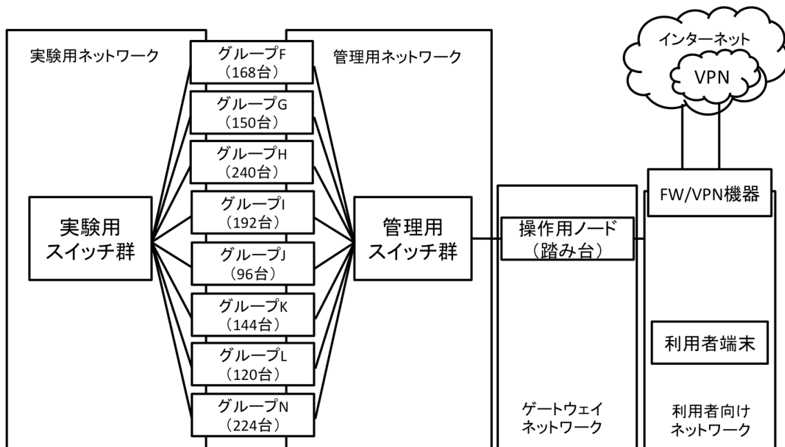
図 3.1: スターベッドのネットワーク構成
