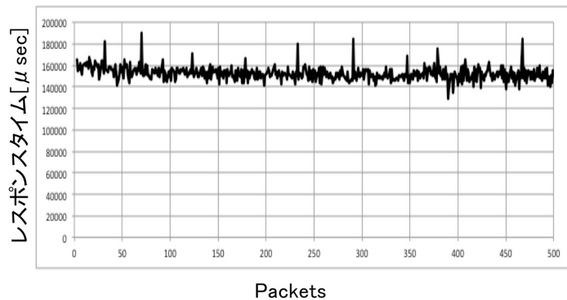
図 4.8: アプリケーションにおける HTTP のレスポンスタイム
