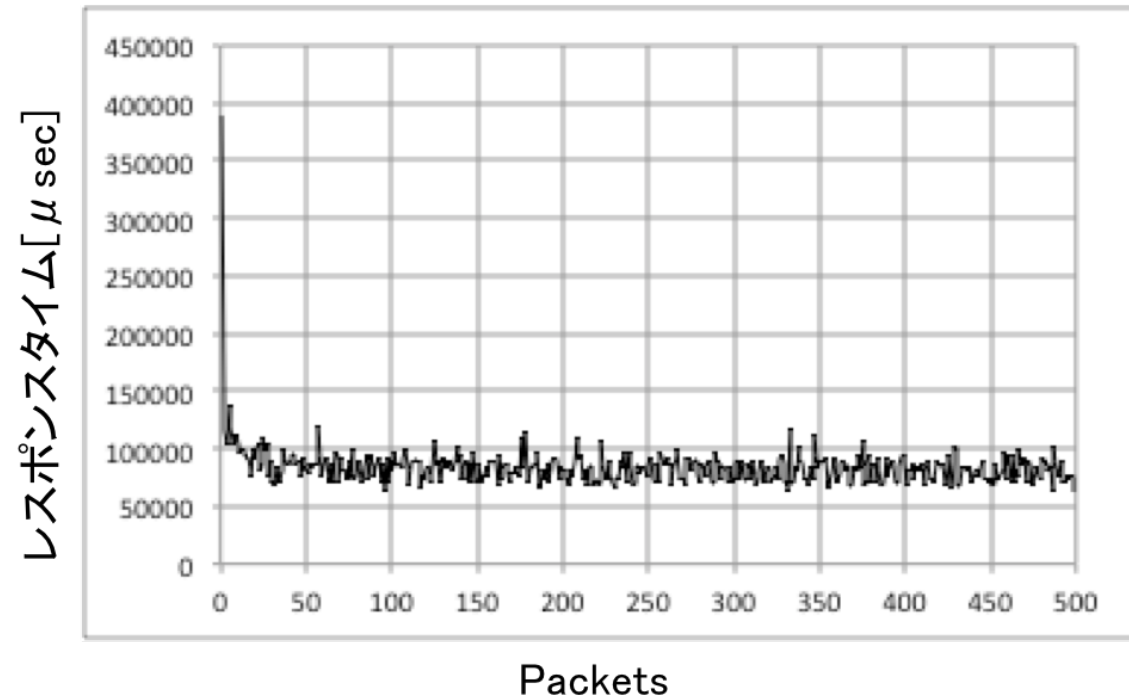
図 5.5: 軽量クライアントモジュールのレスポンスタイム
