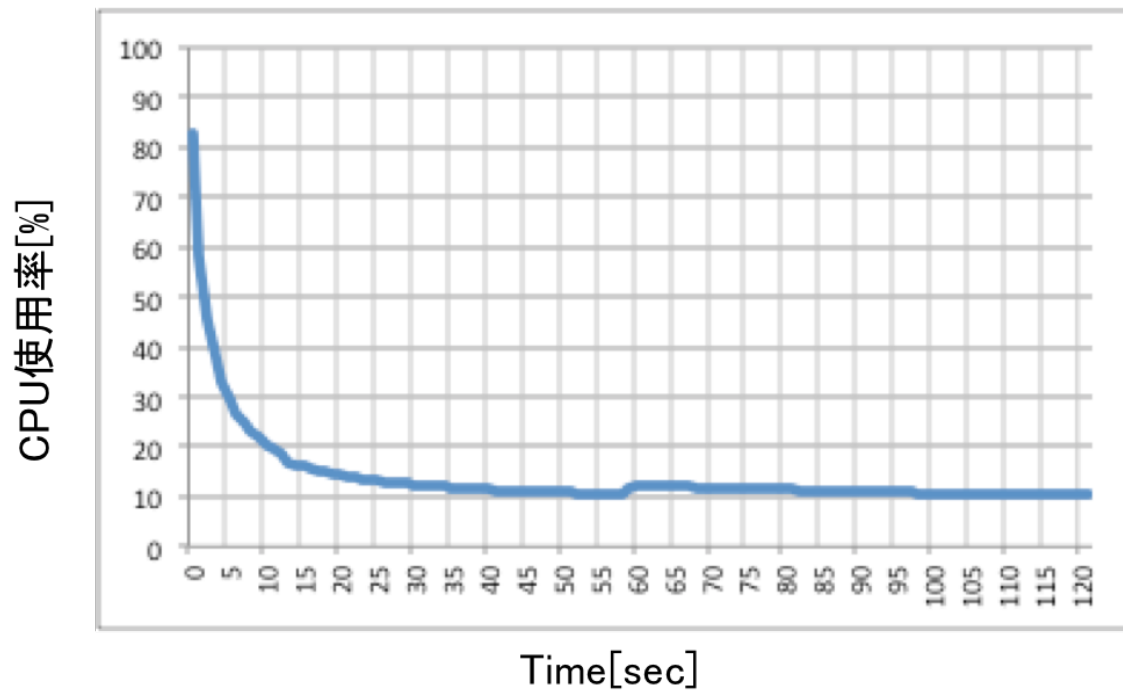
図 4.5: 通信中のアプリケーションの CPU 使用率
