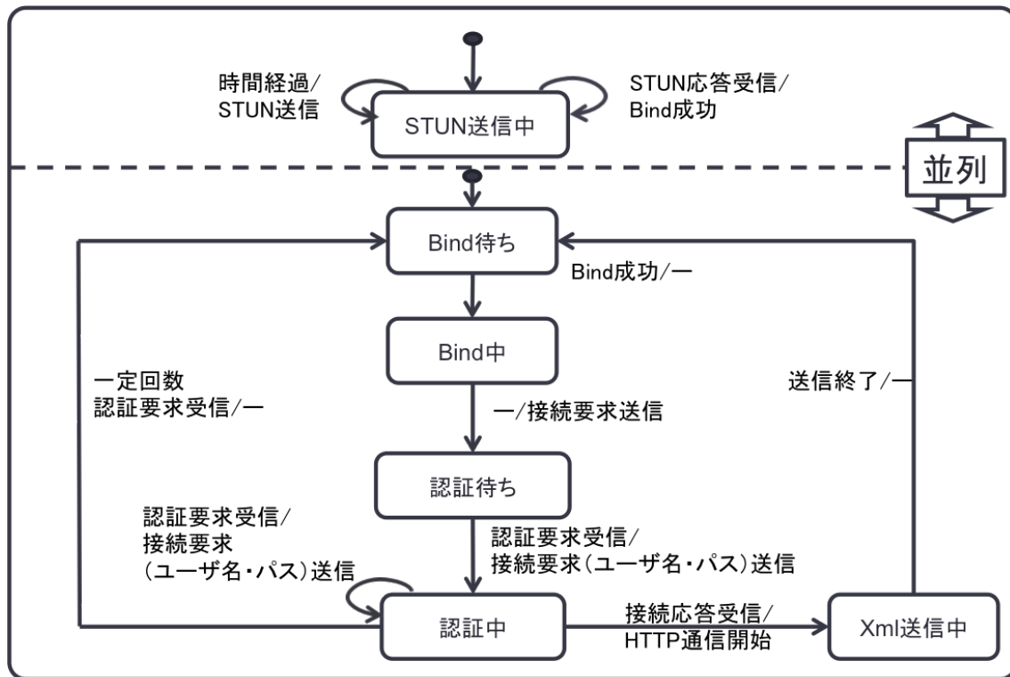
図 4.3: アプリケーションの状態遷移図
