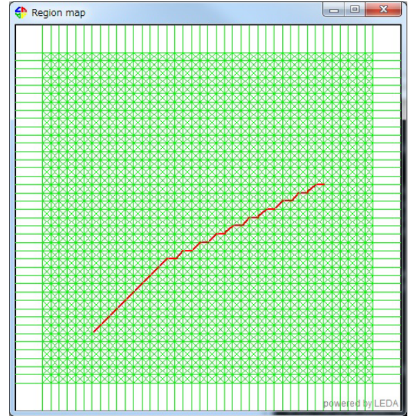
図 2.12: Algorithm3 導入後
