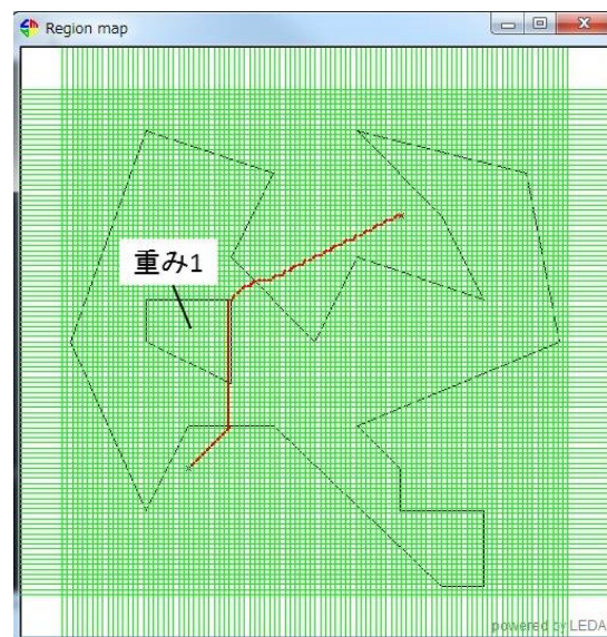
図 3.16: 重み 1 のとき
