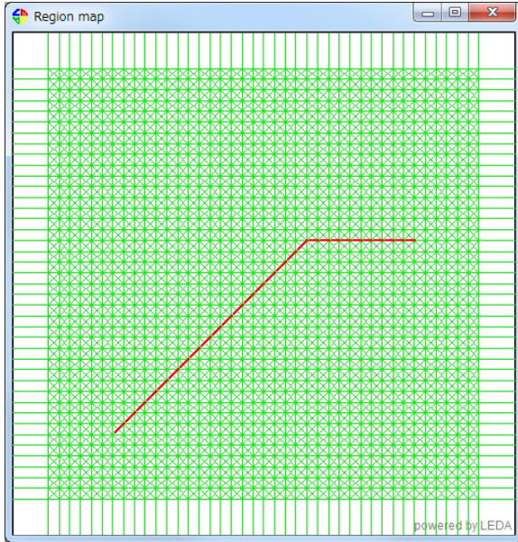
図 2.11: Algorithm3 導入前
