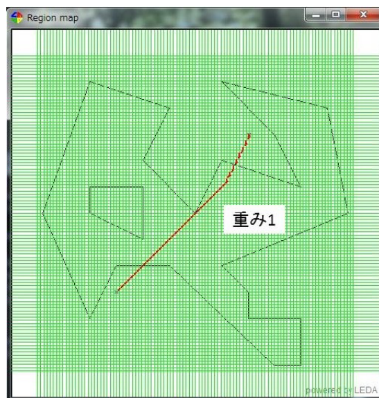
図 3.18: 重み 1 のとき
