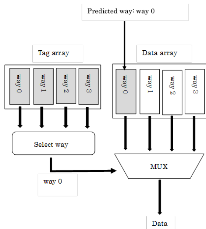
図 2.3: 予測によるウェイ限定参照を行う 4-way セットアソシエティヴ方式のキャッシュアクセス (読み込まれるウェイが影付けされている).
