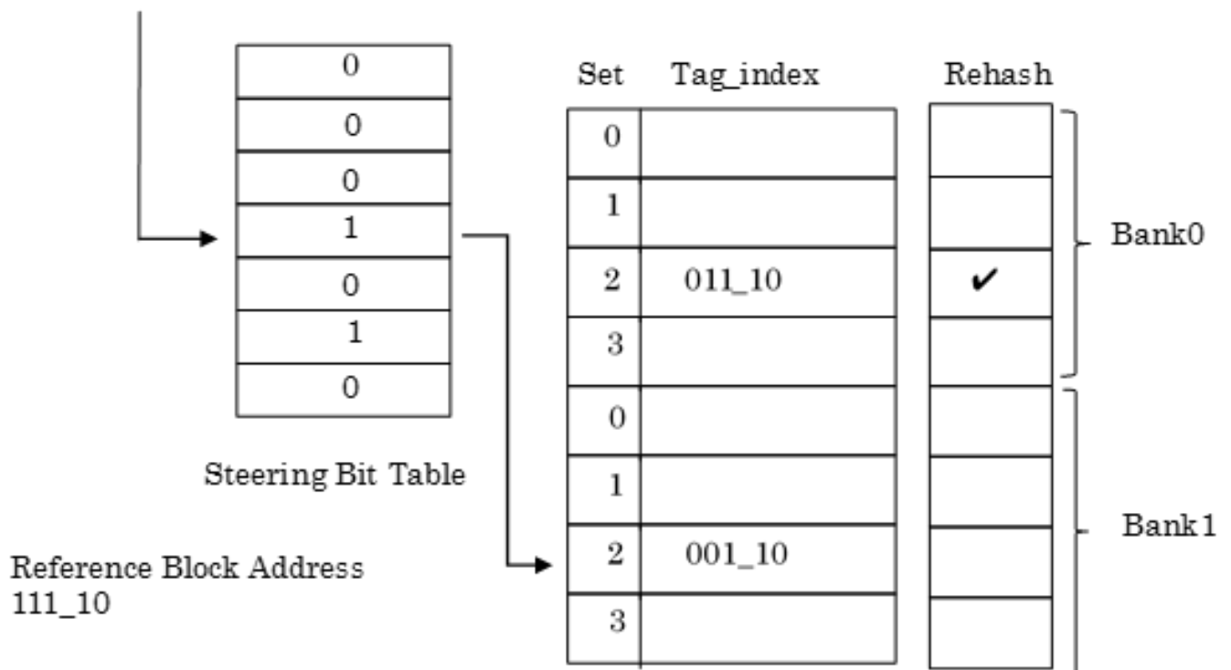
図 2.1: ブロックアドレス 110_10 を参照する際の PSA の振る舞い. まず, Prediction Address をインデックスとして Steering Bit Table のエントリーを参照し, そのエントリーを用いて Bank1 のセットを限定参照 (probe0) している. Bank1 の参照の際に Bank0 の対応するセットの Rehash Table を参照し, Rehash 値が有効となっているため Bank0 への probe1 を行う. しかしながら, Bank0 への probe1 はキャッシュミスとなり, LRU 管理によってブロックを置き換える.
