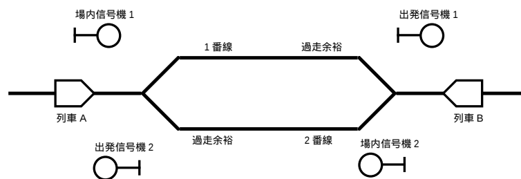
図 5.4: 過走余裕
