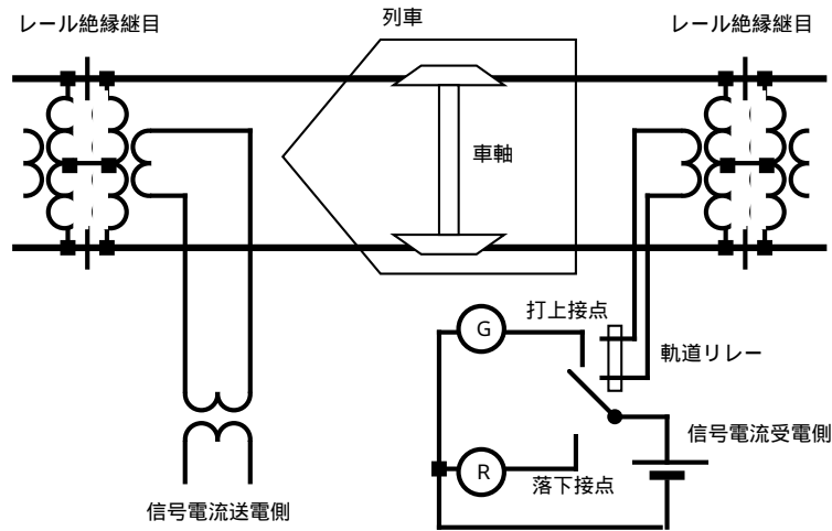
図 4.4: インピーダンスボンドと商用周波数軌道回路
