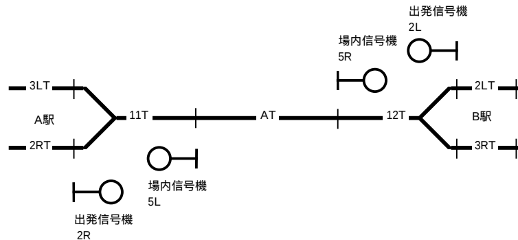
図 5.10: 典型的な単線自動閉そくの配線略図
