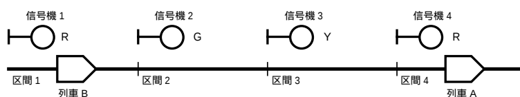
図 4.2: 追突防止の信号機
