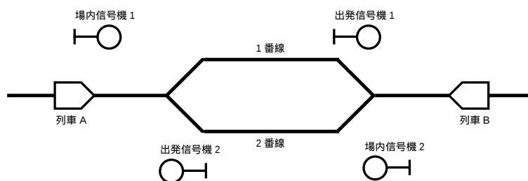
図 5.2: 最小限の行き違い設備
