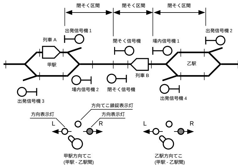
図 5.5: 単線区間における自動閉そくの設備
