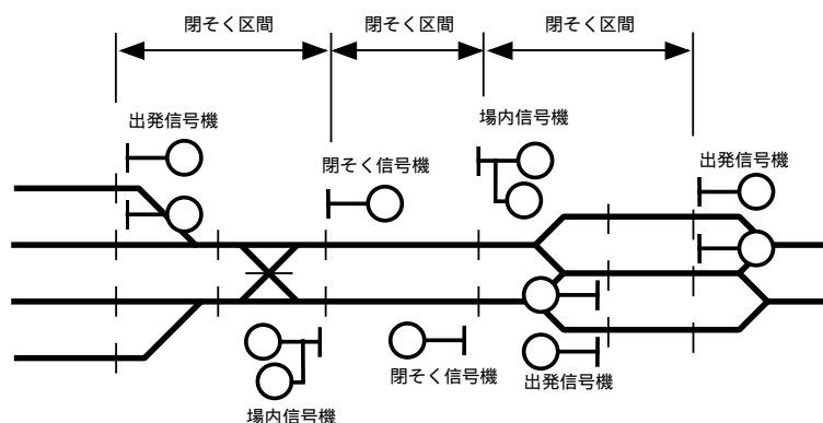
図 4.3: 複線区間における自動閉そくの設備
