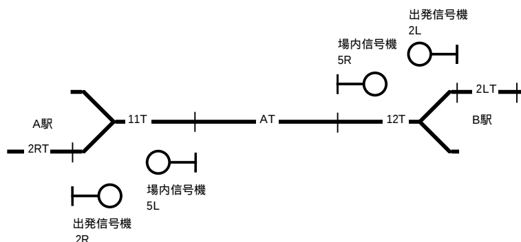
図 5.11: 自動 B の駅間コンポーネント
