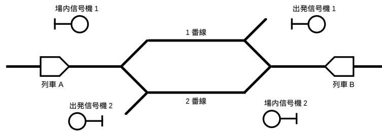
図 5.3: 安全側線
