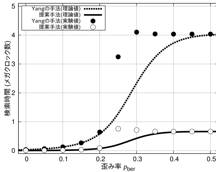
図 4.1: 歪み率と平均検索時間
