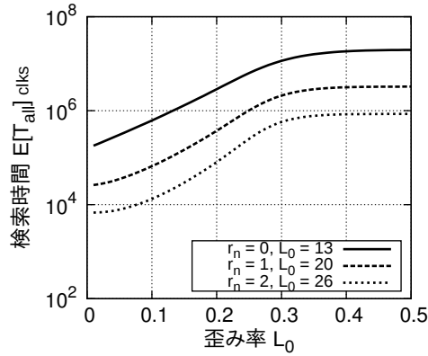
図 A.4: 全体の検索時間の期待値
