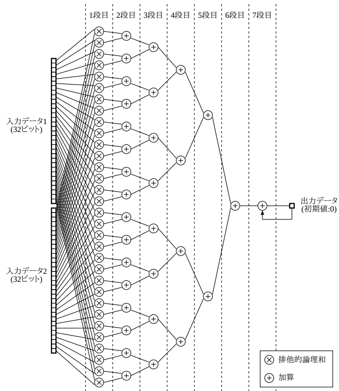
図 2.9: ハミング距離を計算するハードウェア
