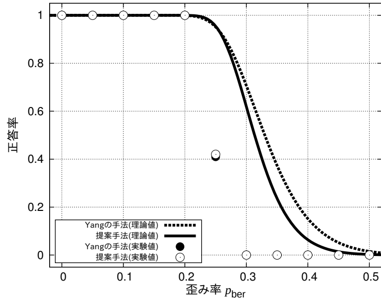
図 4.2: 歪み率と検索精度
