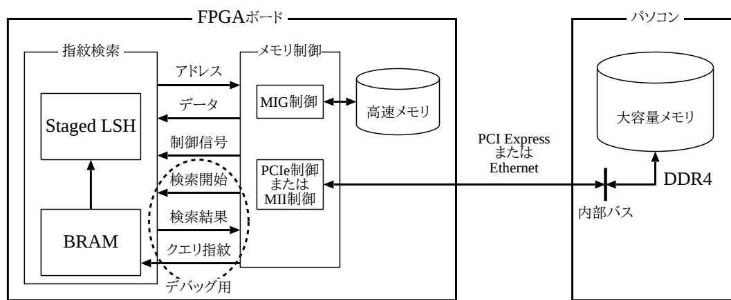
図 3.7: 音楽指紋検索のシステムと内部モジュールの構成図
