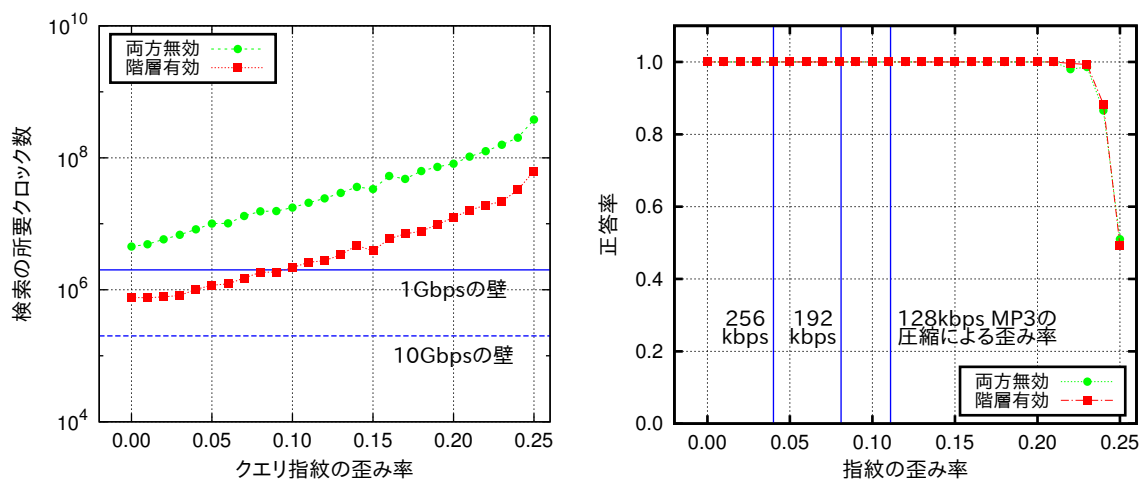
図 4.4: 隣接 LSH 探索の評価の歪み率と平均検索時間・検索精度
