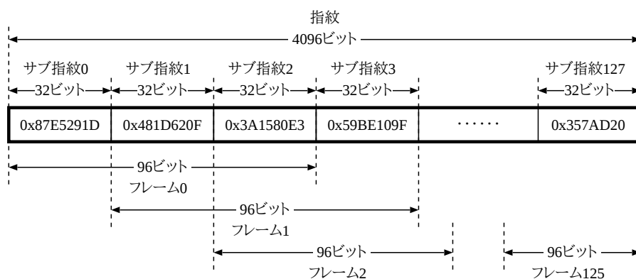
図 2.11: 指紋とサブ指紋とフレーム
