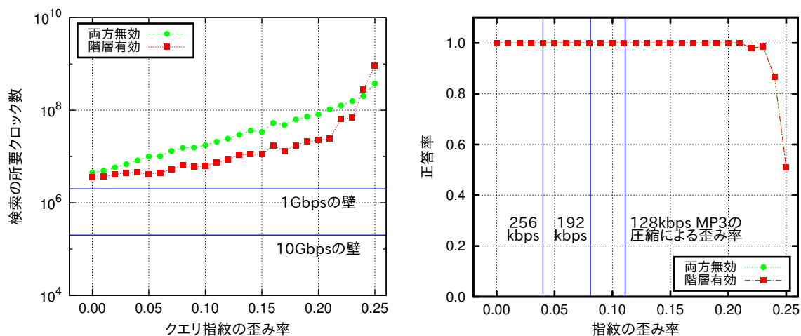
図 4.3: 階層化 Staged LSH の評価の歪み率と 平均検索時間・ 検索精度
