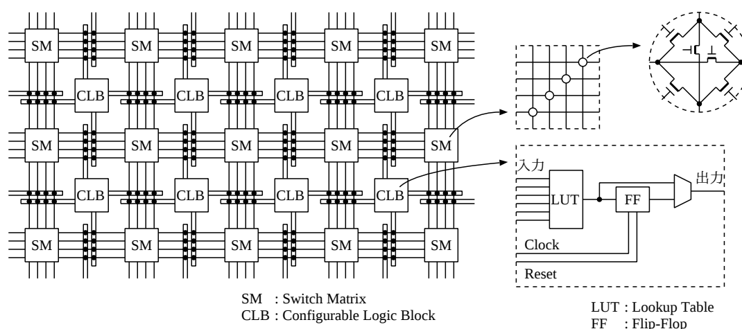
図 3.2: FPGA の基本的な構造の例
