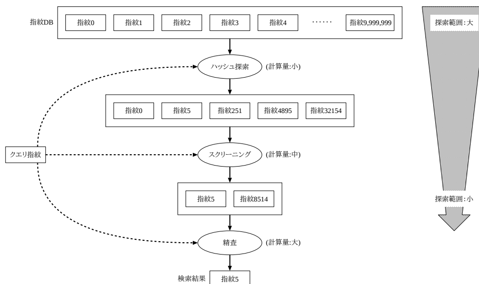
図 2.12: Staged LSH で徐々に指紋 DB の探索範囲を狭めていく様子
