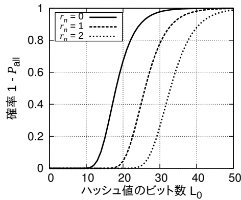
図 A.3: ハッシュ探索が126回全て失敗する確率
