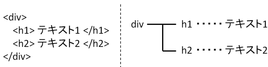
図 3.1: HTML ページと DOM の例
