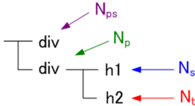
図 3.5: node の位置関係
