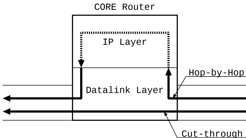
図 2.1: ホップ・バイ・ホップ状態とカット・スルー状態
