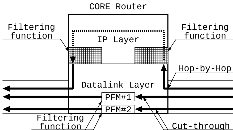
図 4.3: PFM による方式
