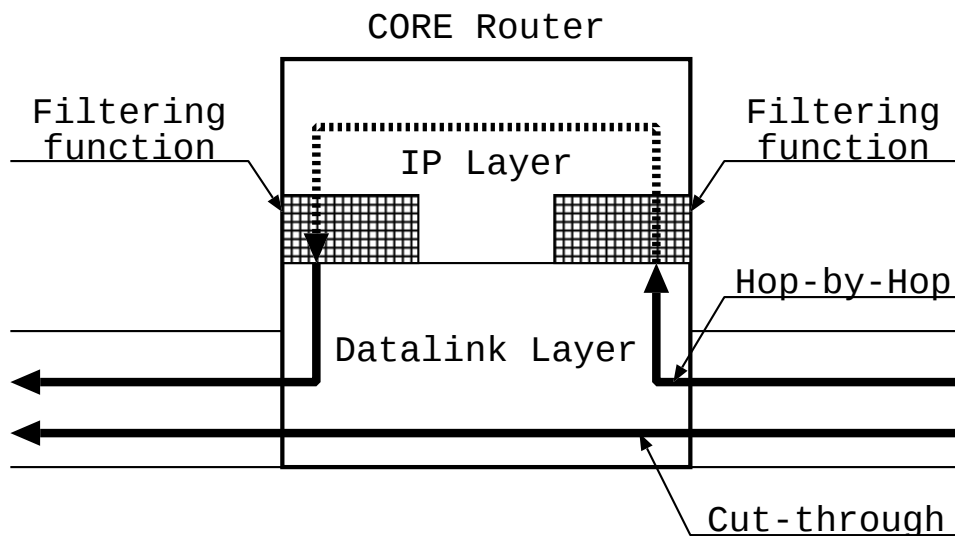
図 4.1: カット・スルーとパケット・フィルタ
