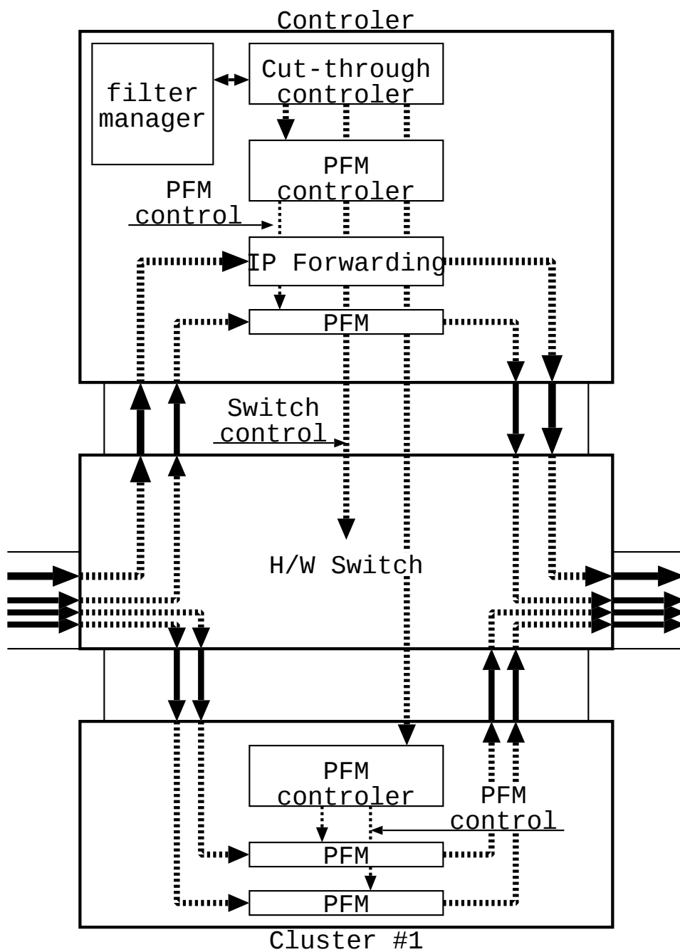
図 5.3: PFM 方式の全体構成 (クラスタリング)
