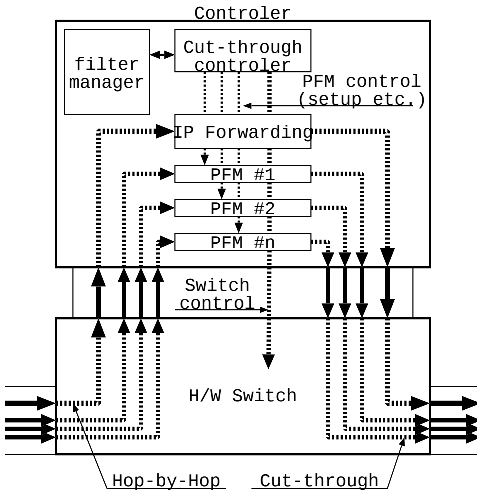
図 5.2: PFM 方式の全体構成
