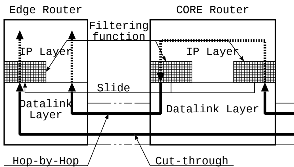
図 4.4: フィルタリングを行う位置をスライドさせる方式
