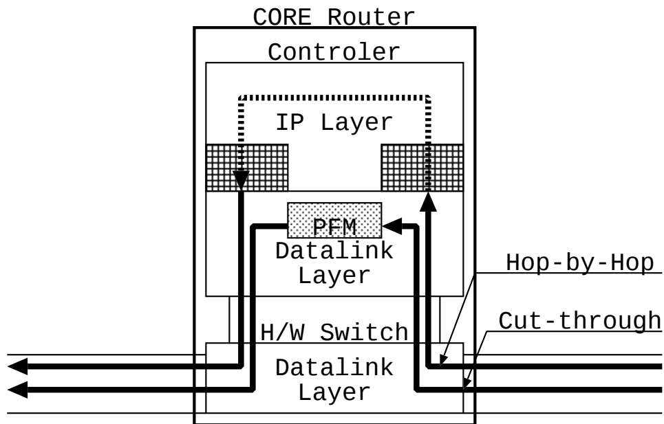
図 5.1: 擬似カット・スルー
