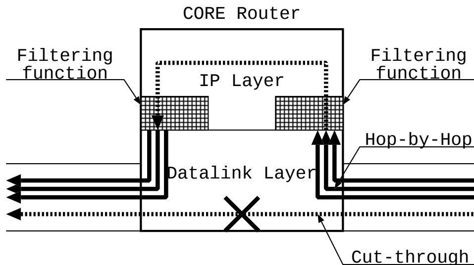
図 4.2: カット・スルーの禁止による方法
