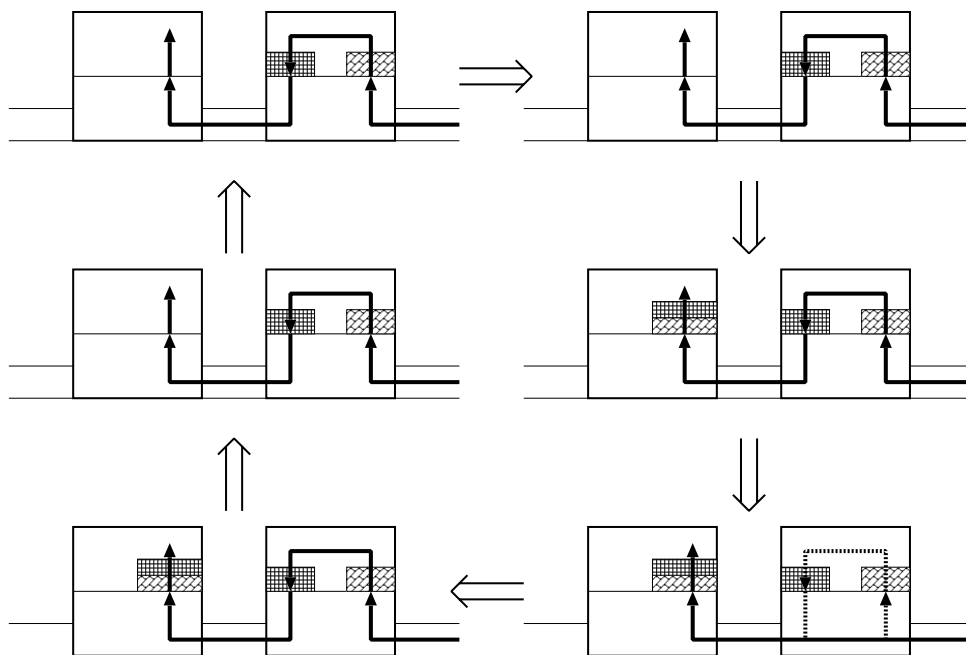
図 6.1: 次段ルータへ委託する場合の状態遷移
