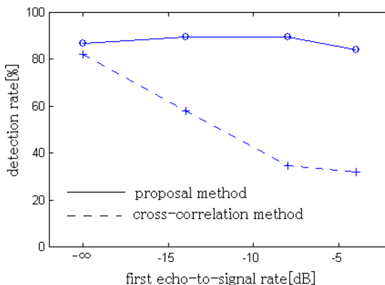
図 4.14: 音源方向推定結果：相関との比較
