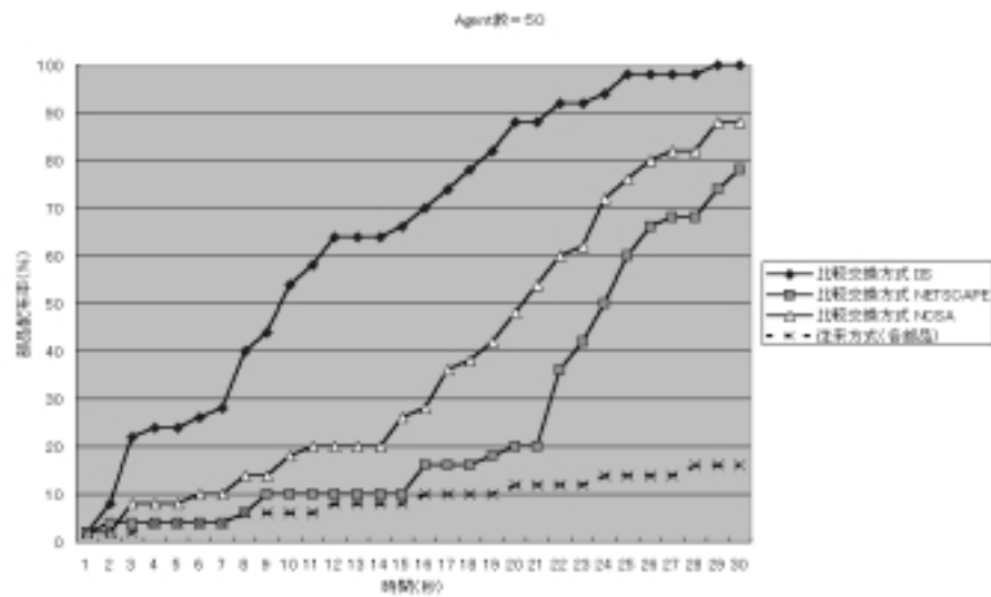
図 6.7: 部品配布率-エージェント数：50
