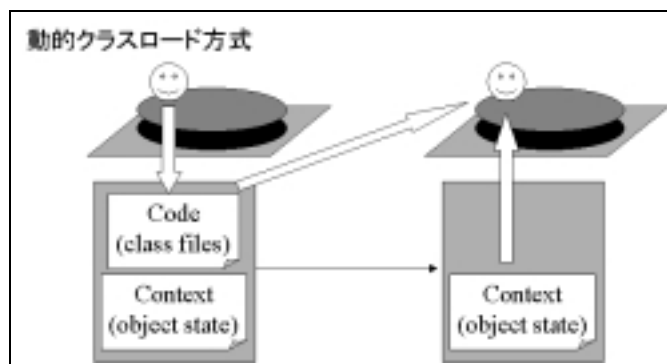
図 2.7: 動的クラスロード
