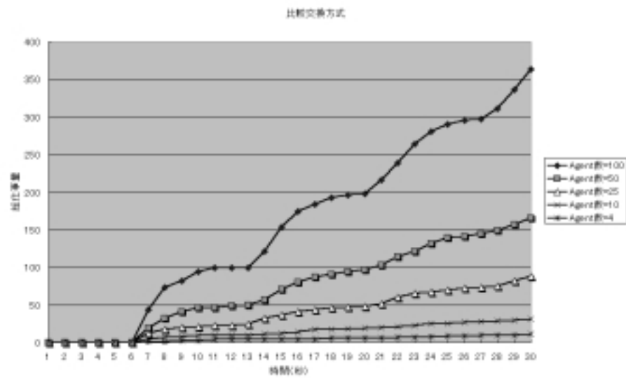
図 6.10: 総仕事量-比較交換方式
