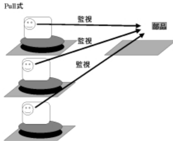
図 4.2: 部品配布方式-Pull 方式
