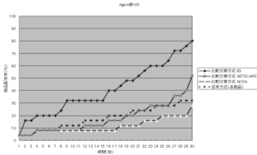
図 6.6: 部品配布率-エージェント数：25
