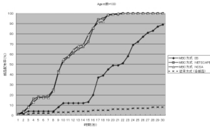
図 6.8: 部品配布率-エージェント数：100
