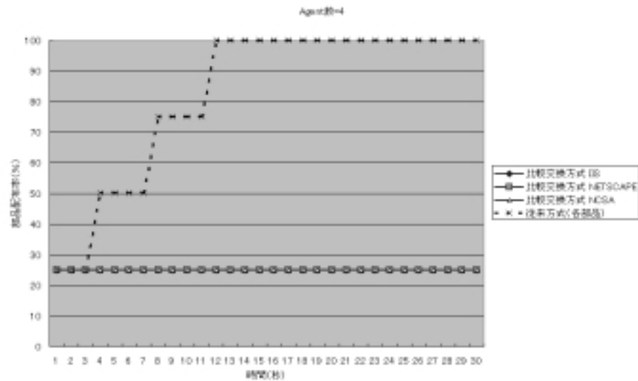
図 6.4: 部品配布率-エージェント数：4
